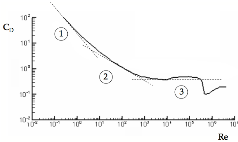
FIGURE 4.11 – Coefficient de traînée C_D = 2F/\rho_f \pi R^2 V^2 en fonction du nombre de Reynolds Re = \rho_f 2RV/\eta_f . Les droites pointillées dans les domaines 1, 2 et 3 ont respectivement une pente -1, -0,5 et 0. Graphique tiré de [63].
