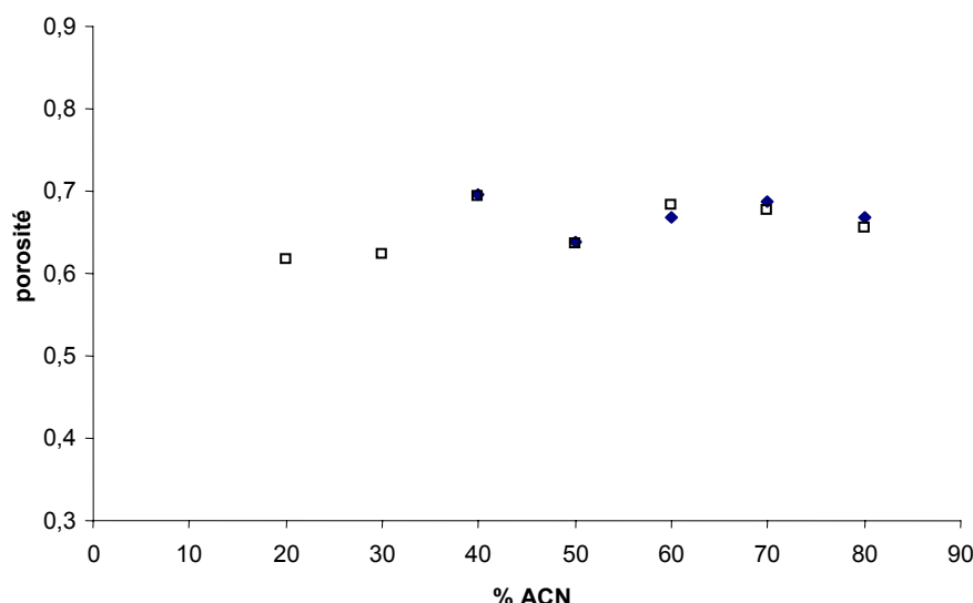
Figure 42 : Evolution de la porosité pour une colonne partiellement ( \square ) et une entièrement ( \blacklozenge ) polymérisée selon le modèle d'Archie en fonction du pourcentage d'acétonitrile de l'électrolyte. Monolithes à base d'hexylacrylate. Colonne partiellement polymérisée : L = 35,5 cm ; l = 27 cm ; d_i = 75 \mu m ; colonne entièrement polymérisée : L = 35,8 cm ; l = 27,3 cm ; d_i = 75 \mu m. Electrolyte : tampon phosphate pH 6,8 en milieu eau-acétonitrile (v/v variable), force ionique = 1,75 mM. Tension : + 25 kV. Température : 25°C.
