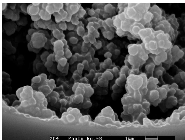
Figure 37: Image MEB d'une section de colonne monolithique obtenue à 2 \text{J}/\text{cm}^2 , capillaire de 75 \mu\text{m} de diamètre interne, mélange à base d'hexylacrylate.
