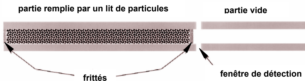
Figure 1: schéma descriptif des divers constituants d'un capillaire rempli par des particules de silice [1].
