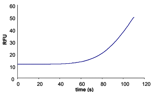
Figure 95 : Evolution du signal de fluorescence en fonction du temps de préconcentration de l'échantillon de fluoranthène ( 0,075 \text{ mg.mL}^{-1} dans eau/acétonitrile 75/25, v/v). Microsystème n°1 : voir Tableau 13. Phase mobile : tampon phosphate pH 6,8 en milieu eau-acétonitrile (80/20 v/v), force ionique = 1,75.10^{-3} \text{ M} . Injection en mode « gated » : 1 : 500 V, 2 : 500 V, 3 : 3000 V, 4 : -3000 V. Détection par fluorescence \lambda_{\text{exc}} = 310\text{-}390 \text{ nm} à 0,7 mm, fréquence d'acquisition 15pts/s. Largeur de la fenêtre de détection de 0,15 cm.
