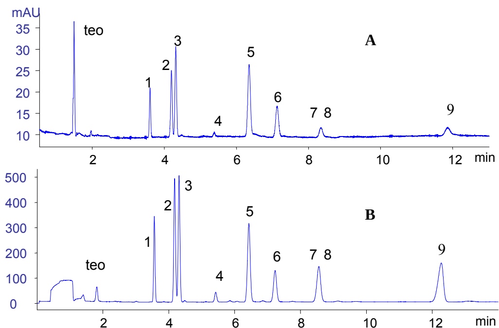
Figure 85 : Electrophorégrammes d'un mélange dilué de 9 HAP à la concentration de 40 ppm dans un milieu aqueux contenant 25 % d'acétonitrile. Séparation sous 30 kV à 25 °C avec une phase mobile constituée d'un mélange acétonitrile - tampon acétate, 5mM, pH 7,1 (80:20, v/v). Colonne à base
