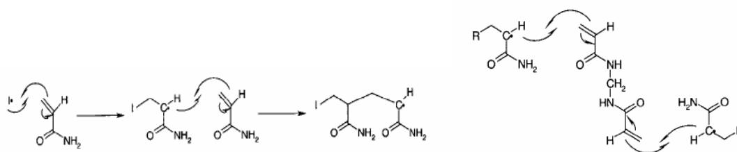
Figure 13 : Schéma réactionnel des différentes étapes de la réaction de polymérisation entre les monomères d'acrylamide et de N,N'-méthylènebis(acrylamide) : réaction de l'initiateur, propagation en chaîne et réticulation [58].
