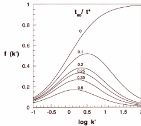
Figure 70 : Exemple d'influence des facteurs de rétention sur la résolution pour différentes valeurs de t_0/t_{mc} , avec f(k) = (k / (1+k)) \cdot (1 - t_0/t_{mc}) / (1 + (t_0/t_{mc}) \cdot k) , en supposant k_1 \approx k_2 [25,27].
