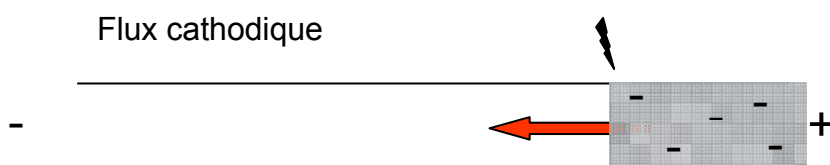
Figure 107 : Schéma du FEO engendré par les groupements carboxylates de la phase stationnaire monolithique.
