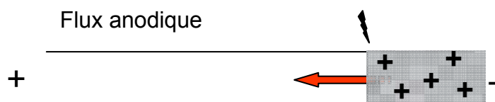
Figure 110 : Schéma du FEO engendré par les groupements amine protonés greffés sur les groupements carboxylate de la phase stationnaire.
