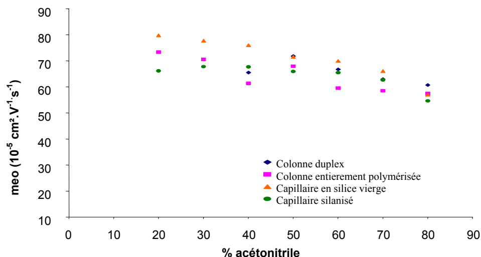
Figure 48 : Evolution de la mobilité électroosmotique réelle pour divers types de colonnes en fonction du pourcentage en volume d'acétonitrile présent dans l'électrolyte. Colonne : longueur utile 27.5 cm, longueur totale, 36 cm. Electrolyte : tampon phosphate pH 6,8 en milieu eau - acétonitrile (v/v variable), force ionique : 1,75 mM. Température : 25 °C. Détection par absorbance UV à 200 nm. Injection électrocinétique : 4 kV/ 4s
