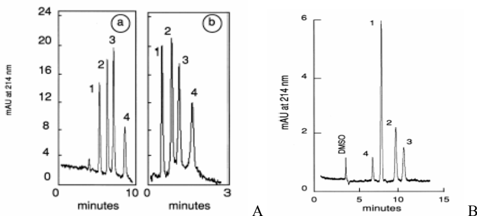
Figure 12 : (A) Chromatogrammes obtenus en micro-CPL sur une colonne monolithique de PS-DVB de dimension 75 \mu\text{m} x 27/ 38cm. Phase mobile : gradient linéaire de 20 à 75% d'acétonitrile dans l'eau contenant 0,1% d'acide trifluoroacétique. Echantillon : (1) ribonucléase, (2) cytochrome c, (3) lysosyme, (4) \beta -lactoglobuline B chacune à 1 mg/mL dans le tampon. (a) débit : 0,34 \mu\text{L/s} ; (b) débit : 1,5 \mu\text{L/s} . (B) électrochromatogramme de polypeptides acides et basiques. Même conditions qu'en (A) pour la phase mobile. Tension : -15 kV. Echantillon : (1) angiotensin II, (2) angiotensin I, (3) [Sar 1 -Ala 8 ]-angiotensin II et (4) insuline, chacun à 4mg/mL dans le tampon [78].
