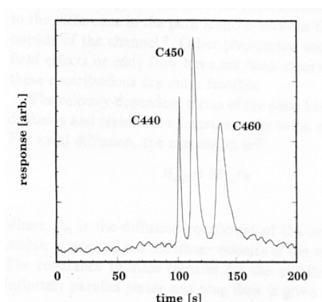
Figure 24 : Electrochromatogramme d'une séparation de 3 coumarines neutres à la vitesse linéaire de 0.65 mm/s. Microsystèmes en verre greffé par des groupements octadécylesilane. Phase mobile : acétonitrile-tampon tétraborate de sodium 10mM, pH=9.2 (25:75, v/v). Injection pincée . Champ électrique imposé : 138 V/cm [129]
