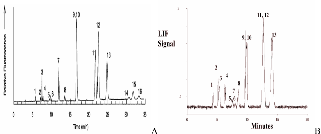
Figure 29 : (A) Séparation réalisée en ECC en capillaire de 16 HAP sur une phase à base de butylacrylate. Phase mobile : acétonitrile – tampon tris 5 mM, pH= 8 (75:25, v/v). Champ électrique : 833 V/cm [115]. Capillaire de 75 µm de diamètre interne. (B) Séparation réalisée en ECC en microsystème de 13 HAP sur une phase à base de butyl-laurylacrylate. Détection réalisée à 7 cm de zones d'injections. Tension de séparation 2 kV. Injection 2kV, 5 s. Phase mobile : acétonitrile, tampon tris 20 mM, pH=8.5 (80:20, v/v) [114].
