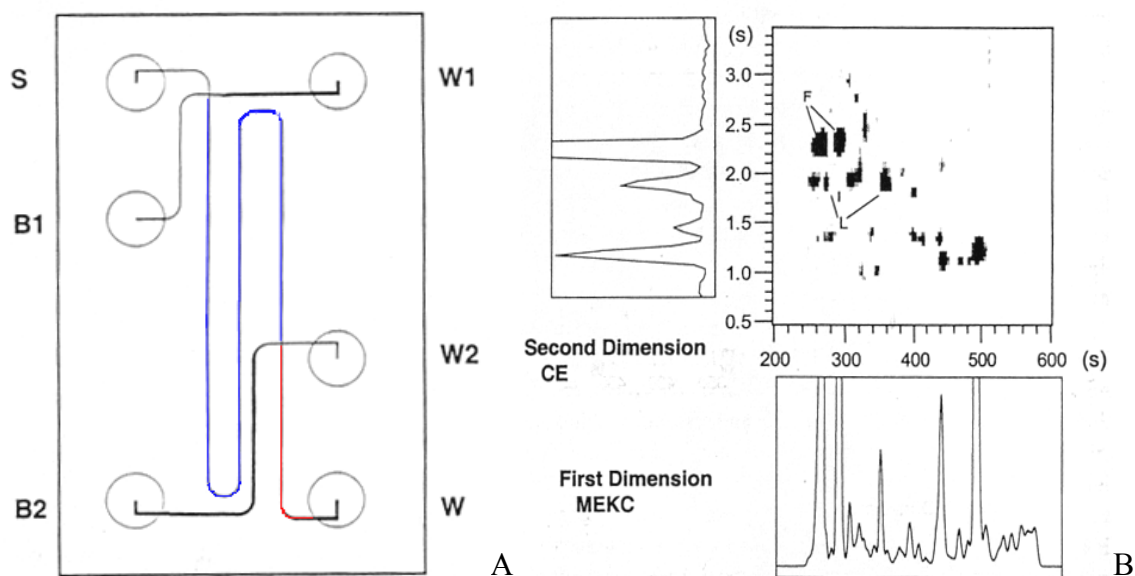
Figure 23 : (A) Schéma du microsystème utilisé pour réaliser des séparations bidimensionnelles. Le premier canal mesure 69 \mu m et le deuxième 10 \mu m. (B) Séparations 1D et 2D de peptides issu d'une digestion tryptique de cytochrome C. Les injections dans la deuxième dimension réalisées toutes les 3s.
