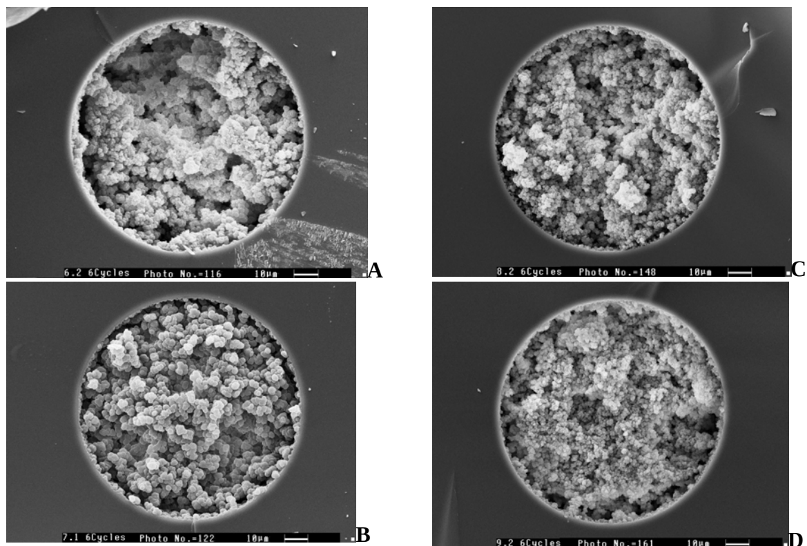
Figure 33 : Observations par microscopie électronique à balayage de colonnes monolithiques à base de butylacrylate dans des capillaires de silice vierge de 100 \mu\text{m} de diamètre interne. Chaque vue correspond à un des prétraitements testés : A, B, C, D.
