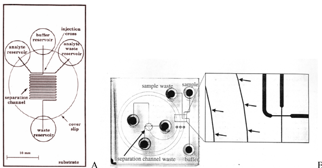
Figure 20 : Schéma de microsystèmes séparatifs électrophorétiques. Les puits sont désignés selon leur utilisation et sont reliés par des microcanaux. (A) [121]. (B) [122]
