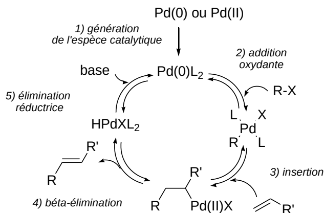
Schéma III.2 : Cycle catalytique de Heck
