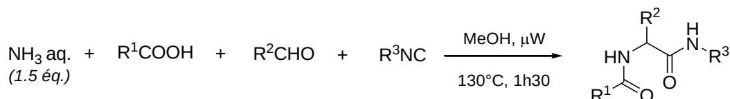
Schéma II.19 : Application à la réaction de Ugi
