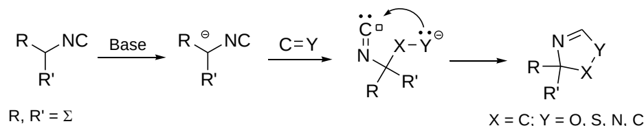
Schéma I.15 : Synthèse d'hétérocycles exploitant l'acidité du H en α d'un isonitrile
