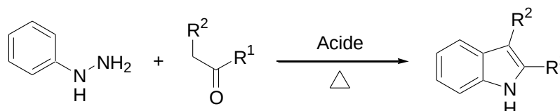
Schéma III.28 : Synthèse d'indole par Fischer
