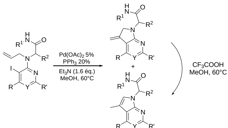
Schéma III.53 : Couplage de Heck sur les adduits de Ugi-Smiles issus d'hétérocycles
