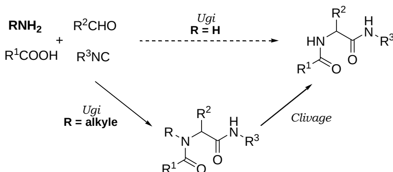
Schéma II.8 : Stratégie en deux temps pour l'obtention des adduits NH
