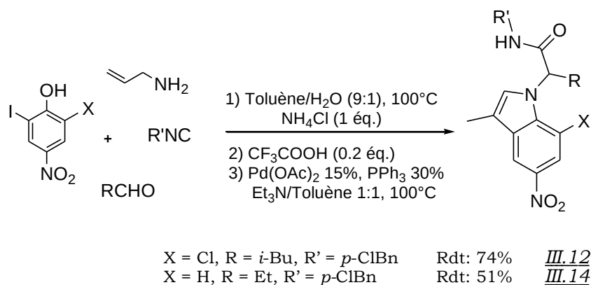
Schéma III.50: Version one-pot du tandem Couplage Ugi-Smiles / Réaction de Heck
