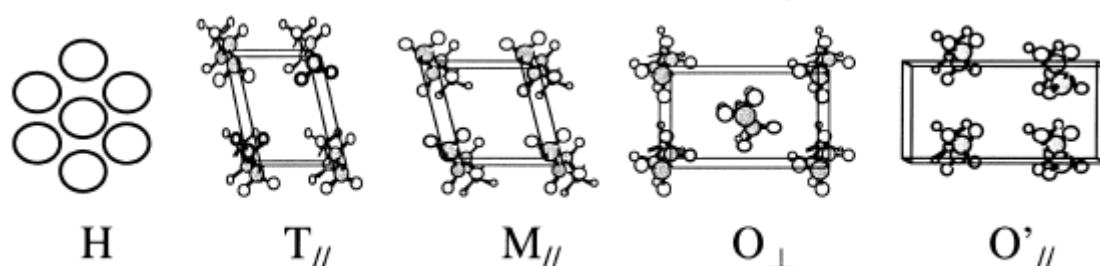
Figure 1.19. Types de sous-cellules adoptées par les chaînes hydrocarbonées cristallisées
