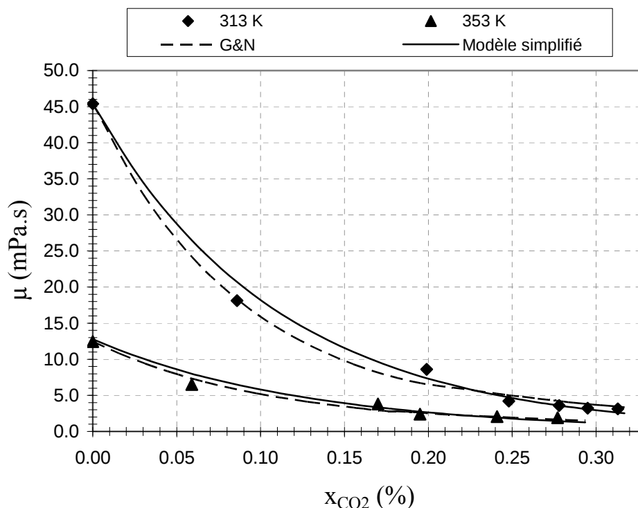
Figure 3.20. Représentation de la viscosité du BC saturé en \text{CO}_2 à 313 et 353 K par le modèle simplifié et le modèle de Grunberg et Nissan
