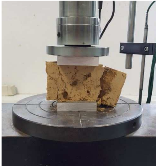
Figure II-18 : Essai de compression simple d'un échantillon prismatique
