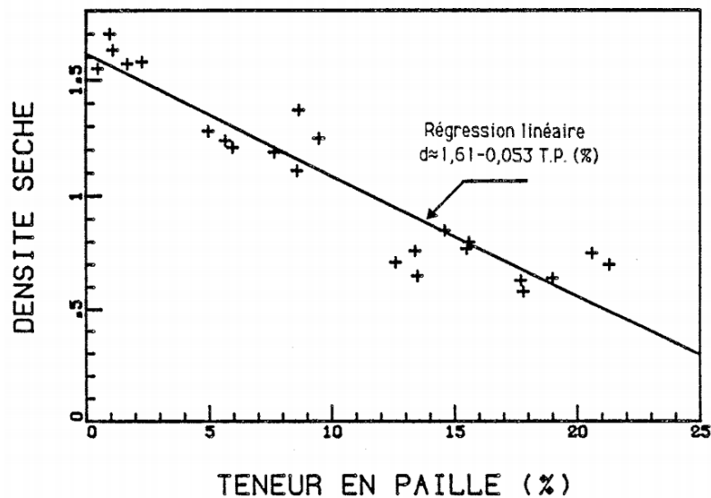
Figure I-37 : Relation teneur en paille/densité sèche ( \text{tonne.m}^{-3} ) correspondante (Laurent, 1986)
