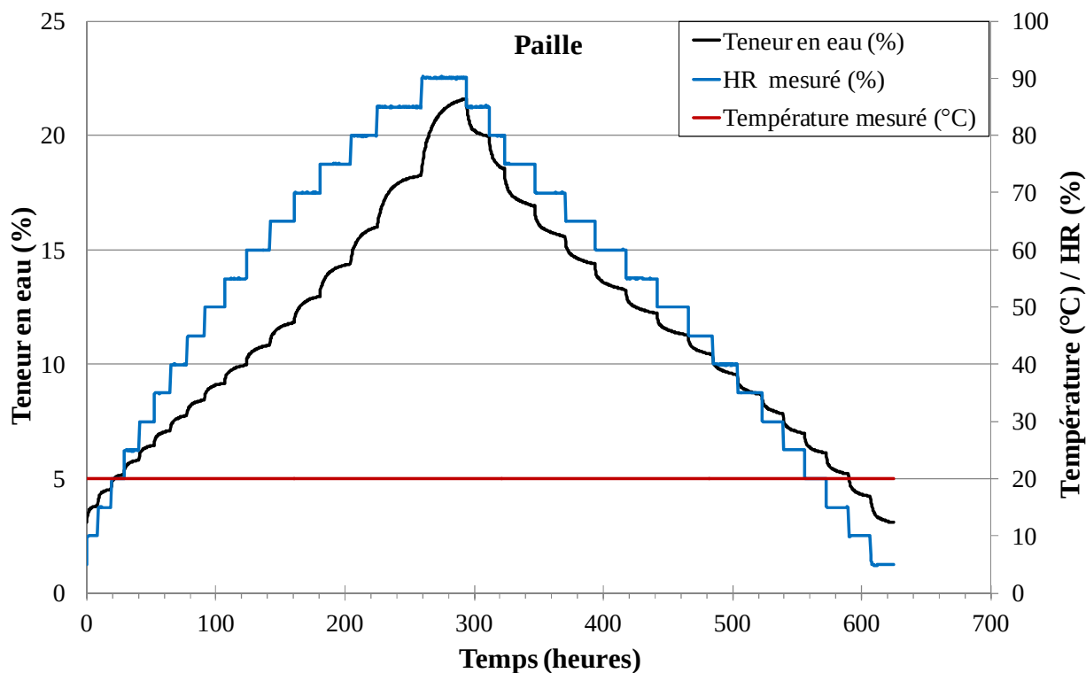
Figure IV-9 : Variation de la teneur en eau de la paille, de l'humidité relative et de la température au cours d'un cycle sorption/désorption
