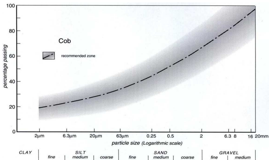
Figure I-7 : Courbe granulométrique recommandé par (Clark, 2013)
