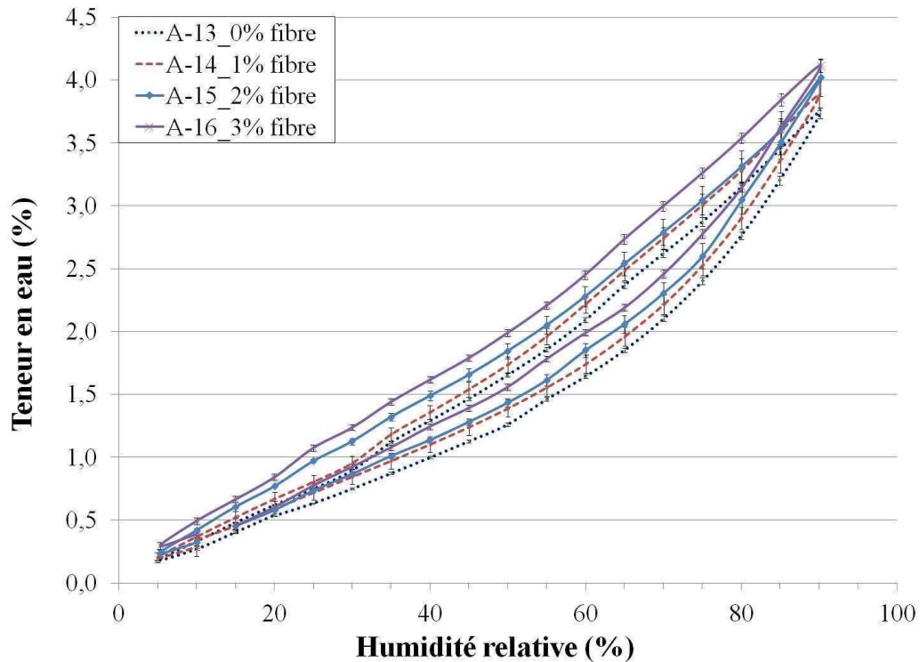
Figure IV-16 : Isotherme de sorption/désorption de différentes formulations du mélange A
