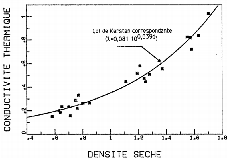
Figure I-38 : Variation de la conductivités thermique ( \text{W.m}^{-1}.\text{K}^{-1} ) en fonction de la densité sèche ( \text{tonne.m}^{-3} ) (Laurent, 1986)
