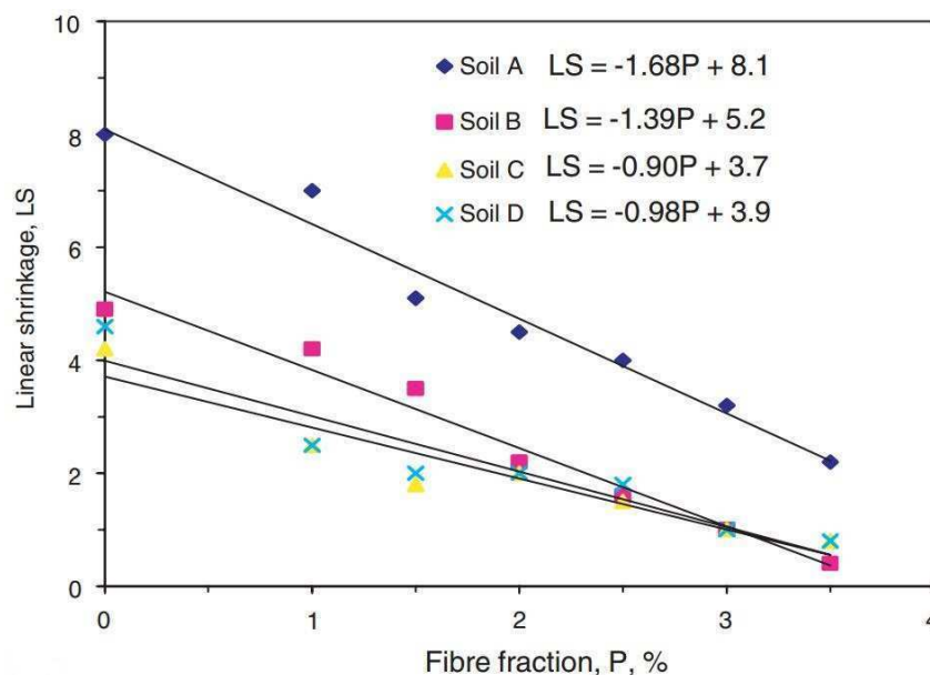
Figure I-23 : Variation du retrait en fonction de la teneur en fibre (Bouhicha et al., 2005)
