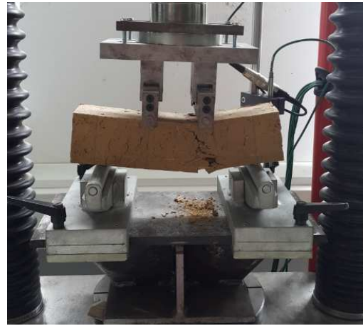
(b) Mélange B avec 2 % de fibre
