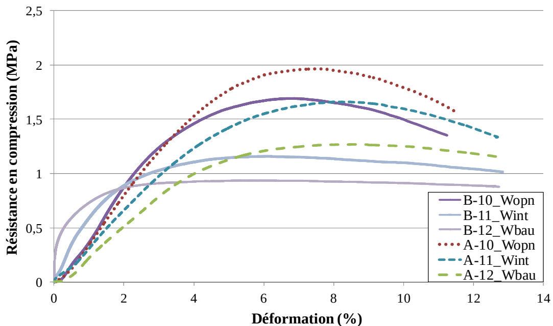
Figure III-7 : Courbe contrainte-déformation des deux mélanges à différentes teneurs en eau initiales
