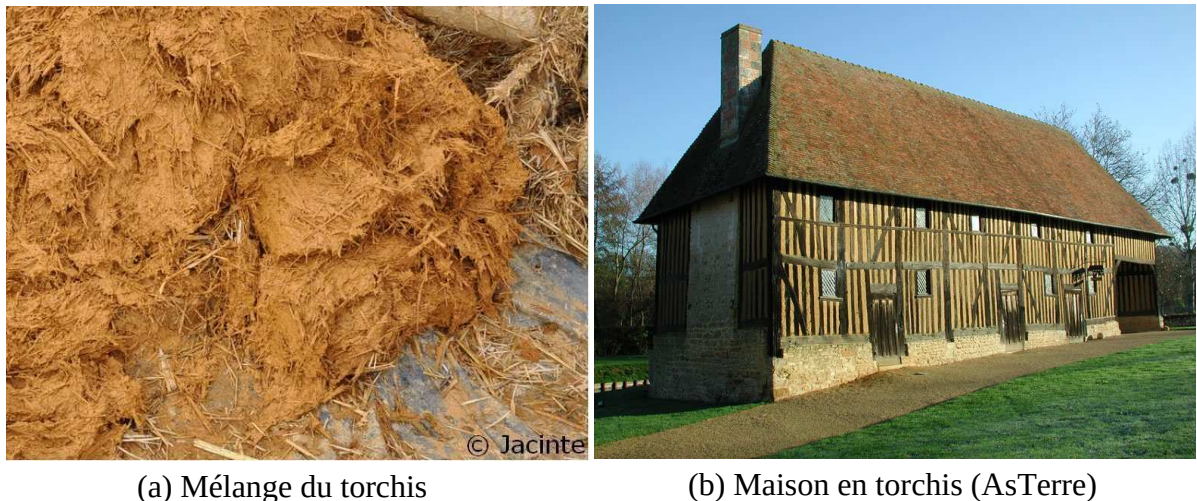
Figure I-3 : Construction en torchis (Sources Internet)
