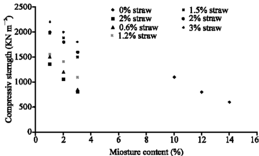
Figure I-30 : Variation de la résistance en compression en fonction de la teneur en eau (Akinkurolere et al., 2006)
