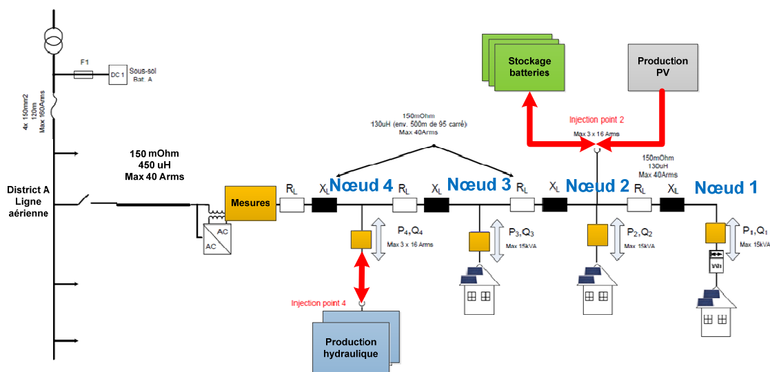
Figure 36 : Schéma électrique
