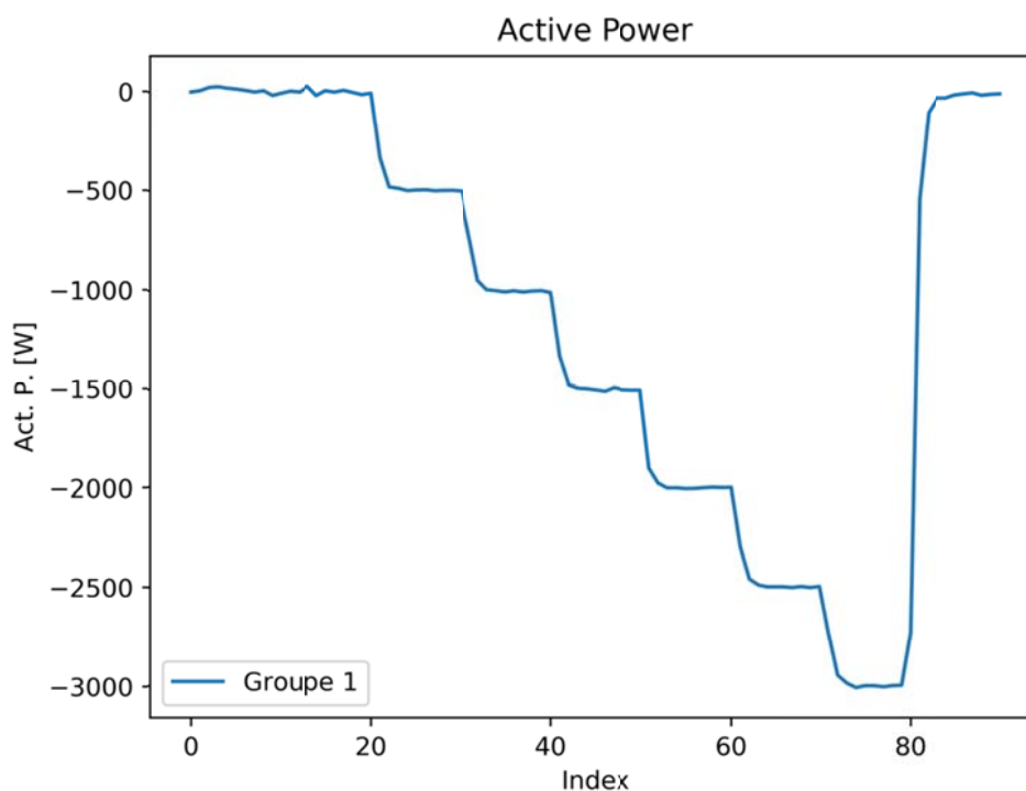
Figure 75 : Graphique puissance active (Dispatching)
