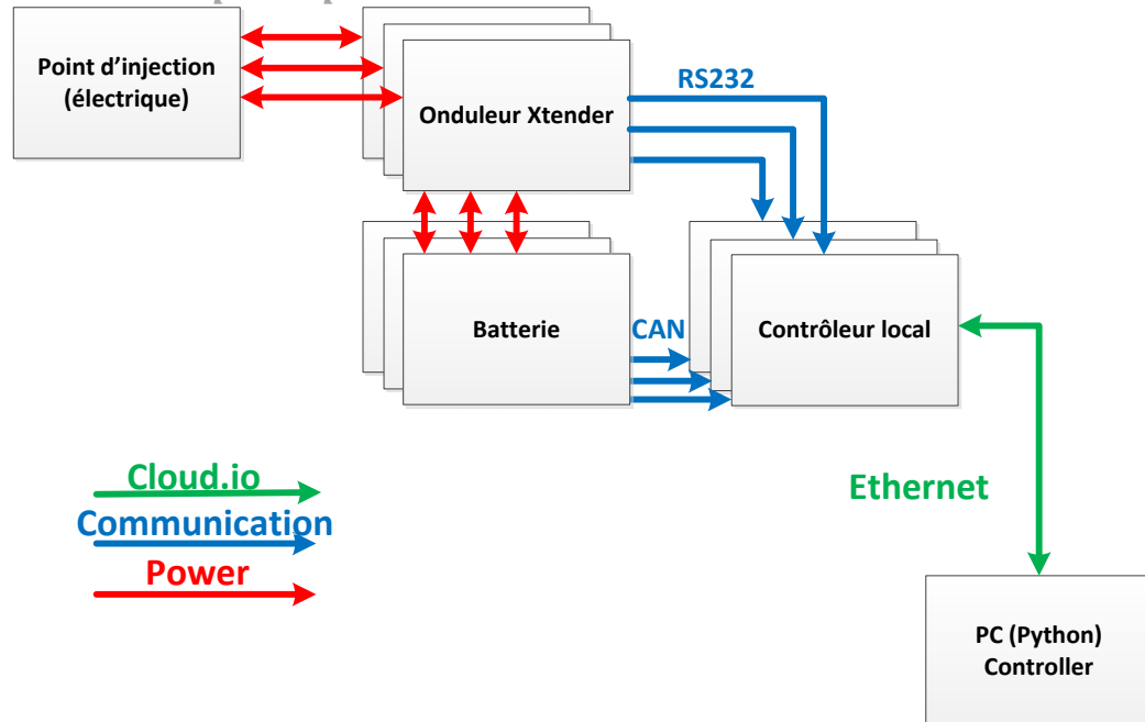
Figure 16 : Schéma batteries
