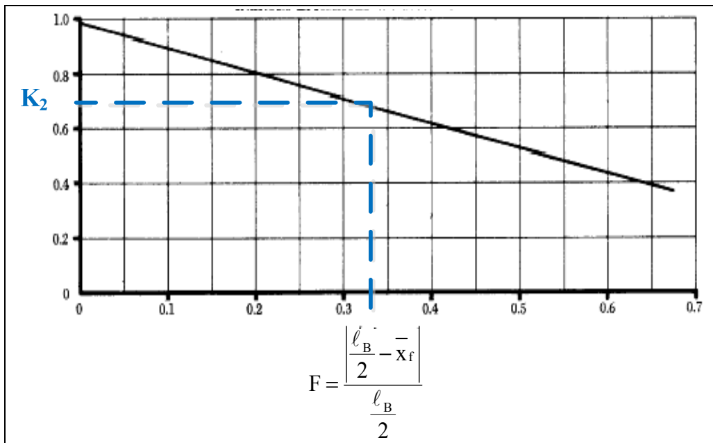
Figure 4.9 - Abaque représentant le facteur de corrélation K_2 de moment de tangage du fuselage (Finck, R. D., 1978)
