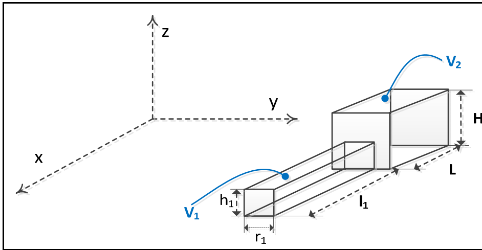
Figure 4.20 - Représentation du modèle de cargo
