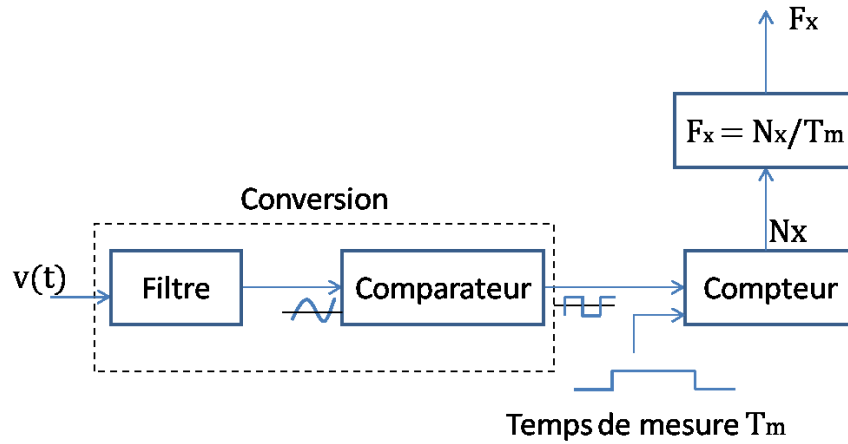
Figure III-13. Principe du fréquencesmètre.
