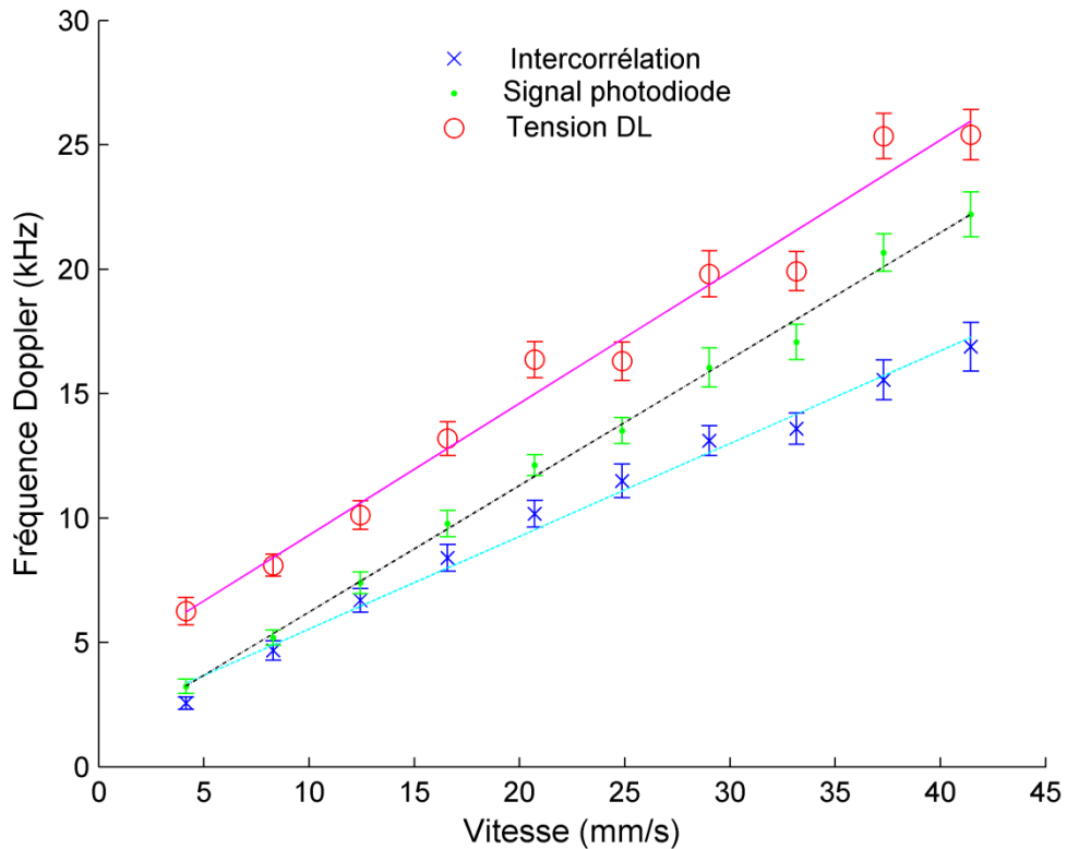
Figure IV-9. Tracé des fréquences Doppler, estimées avec le fréquencemètre, en fonction de la vitesse d'écoulement. L'intervalle de confiance de 95% est présenté. Les signaux de tension et de photodiode ont été filtrés par un filtre passe-bande.
