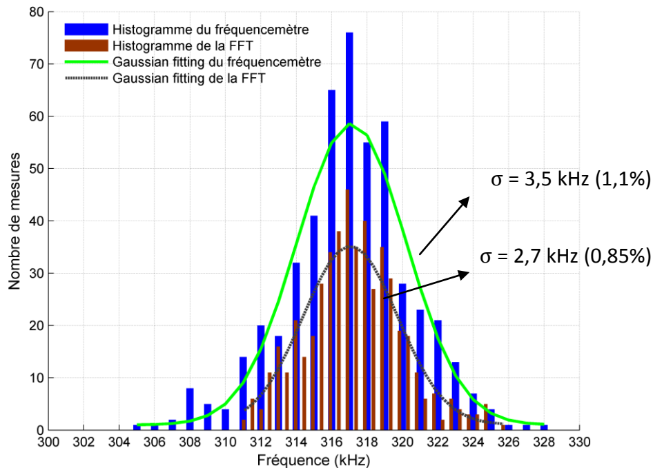
Figure III-32. Comparaison des fréquences estimées par la méthode FFT et le fréquencemètre conventionnel. L'équation de fit de y(x) est : \text{gauss} = A \cdot \exp(-(x-\mu)^2/(2\sigma^2)) + y_{\min} avec A , \mu et \sigma à déterminer et y_{\min} est une constante correspondant au minimum de y .
