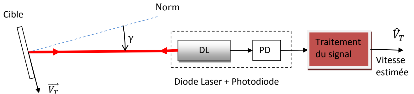
Figure II-1. Prototype du vélocimètre self-mixing mono-diode laser. La cible est en mouvement transverse avec une inclinaison d'un angle \gamma par rapport au faisceau laser à une distance fixe de la diode laser.
