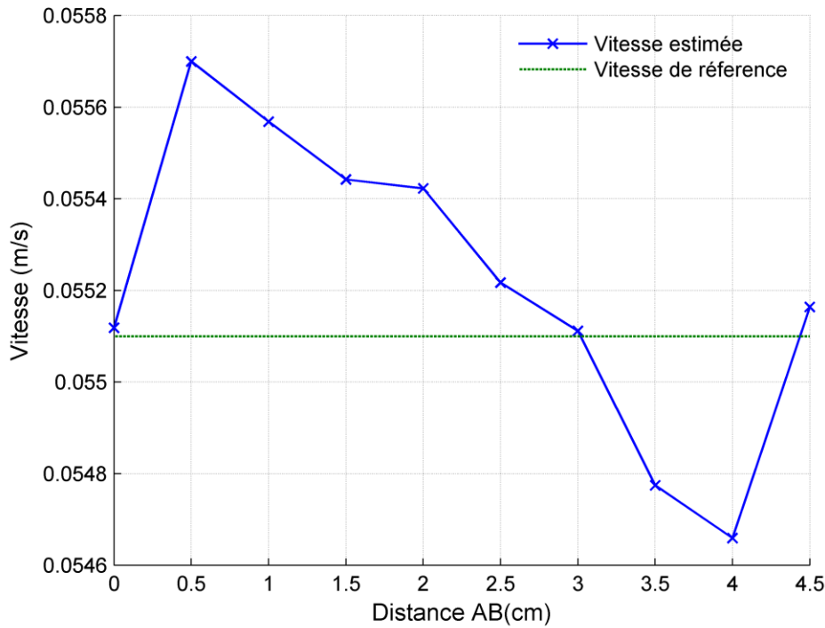
Figure II-18. Variations des mesures de vitesse quand les faisceaux laser sont coplanaires mais n'illuminent pas le même point sur la cible. Une moyenne de 600 mesures est représentée à chaque point.
