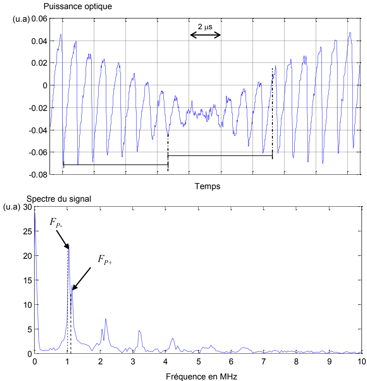
Figure III-9. Signal expérimental de self-mixing qui subit l'effet speckle. Deux pics apparaissent dans le spectre du signal à des fréquences aléatoires F_P et F_{P+} autour de la fréquence Doppler [120].
