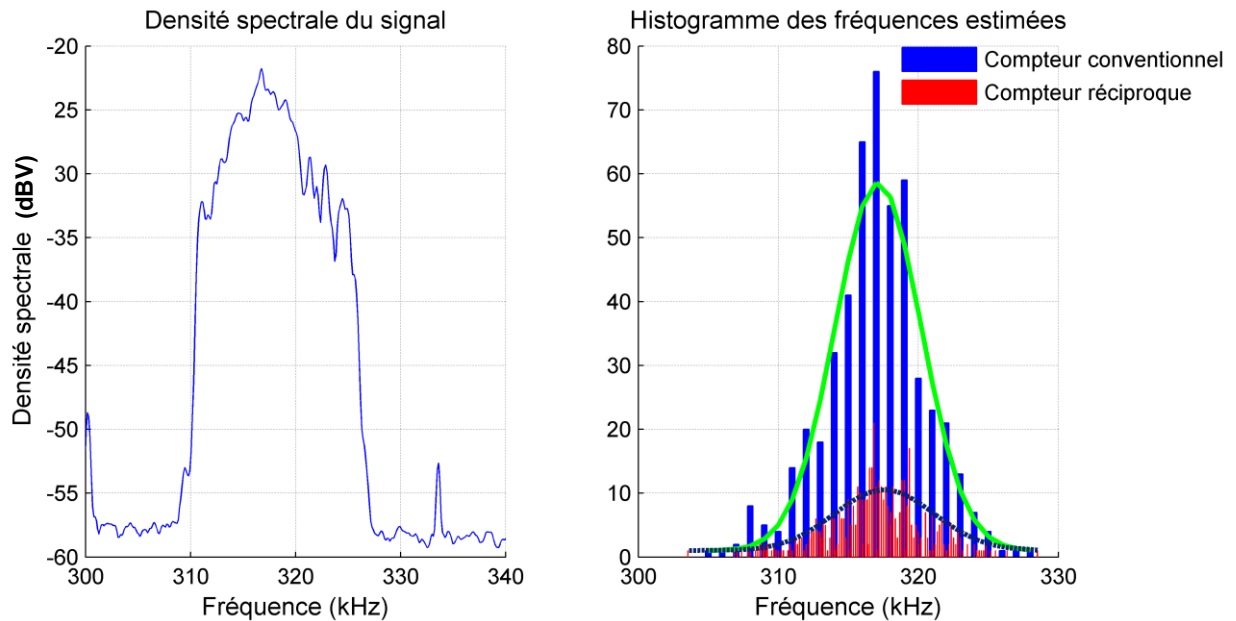
Figure III-31. Comparaison du spectre du signal avec l'histogramme des fréquences mesurées par la méthode de comptage présentées dans la Figure III-30. Les courbes en verre et noir sont des approximations gaussiennes des distributions des mesures de fréquence obtenues avec les compteurs conventionnel et réciproque. L'équation de fit de y(x) est : \text{gauss} = A \cdot \exp(-(x-\mu)^2/(2\sigma^2)) + y_{\min} avec A , \mu et \sigma à déterminer et y_{\min} est une constante correspondant au minimum de y . Conditions expérimentales : matériau : cuivre ; distance capteur-cible : 27 cm ; \gamma = 65^\circ ; fenêtre de mesure = 1ms ; nombre de mesures : 500 avec chaque compteur.
