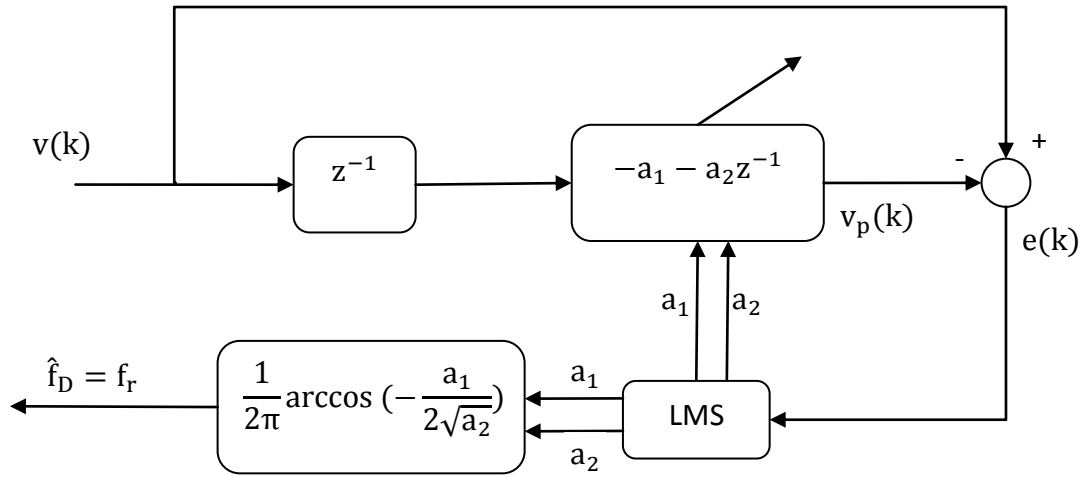
Figure III-12. Tracking de la fréquence Doppler basé sur l'algorithme adaptatif LMS qui permet de calculer de manière adaptative les coefficients a_1 et a_2 du modèle autorégressif AR2.
