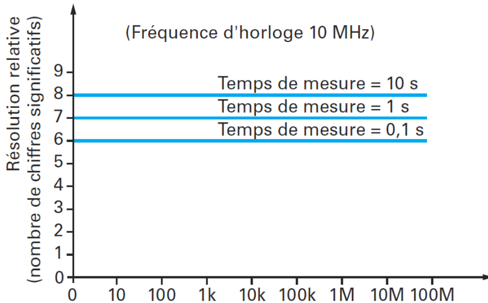
Figure III-21. La résolution relative est indépendante de la fréquence d'entrée pour un compteur de fréquence réciproque [156].
