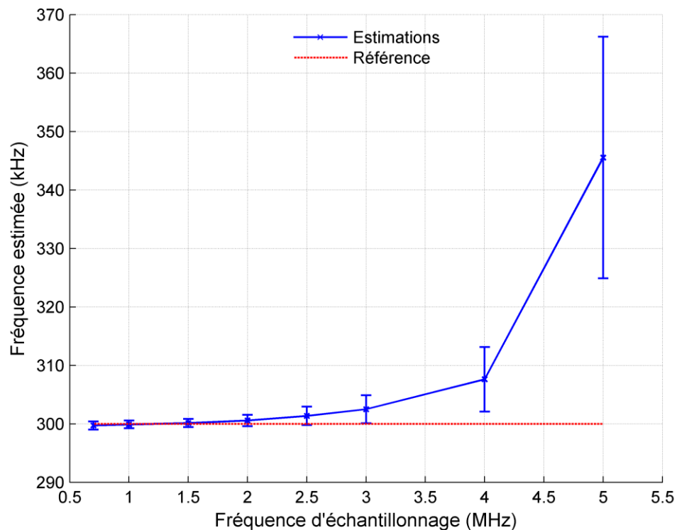
Figure III-25. Représentation des fréquences estimées moyennes en fonction de la fréquence d'échantillonnage (l'intervalle de confiance de 95% est représenté). T_m = 10 \text{ ms} ; F_D = 300 \text{ kHz} . Les basses fréquences sont éliminées avec un filtre passe bas de fréquence réduite de coupure égale à 0,005.
