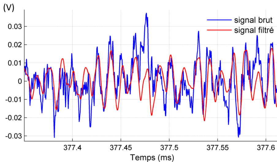
Figure III-40. Filtrage du signal acquis sur le verre avant de l'appliquer à l'entrée du trigger du fréquencesmètre.
