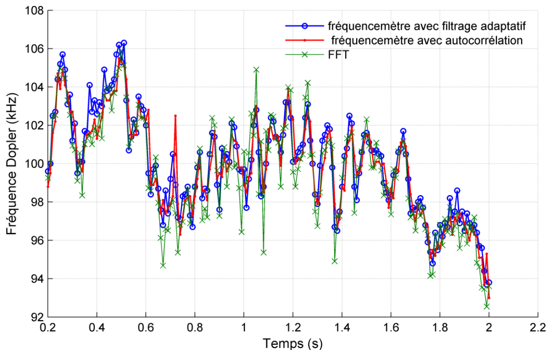
Figure III-44. Mesure de fréquence Doppler d'un signal de self-mixing obtenu sur du verre, utilisant le fréquencemètre avec filtrage adaptatif ou autocorrélation, et l'algorithme FFT.
