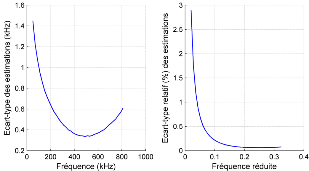
Figure III-24. Ecart-type des estimations de fréquence obtenues par les simulations de Monte Carlo du fré- quencemètre conventionnel. F_e = 2,5 \text{ MHz} ; T_m = 10\text{ms}
