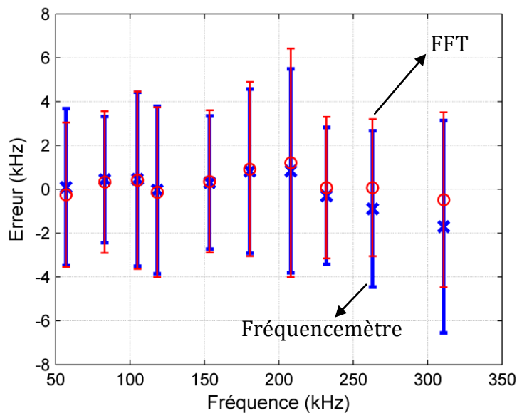
Figure III-36. Mesures de fréquence pour des signaux de self-mixing obtenus en illuminant une cible en cuivre. L'erreur est la différence entre la valeur mesurée et la valeur exacte calculée par un analyseur de spectre. L'intervalle de confiance de 95% est présenté.
