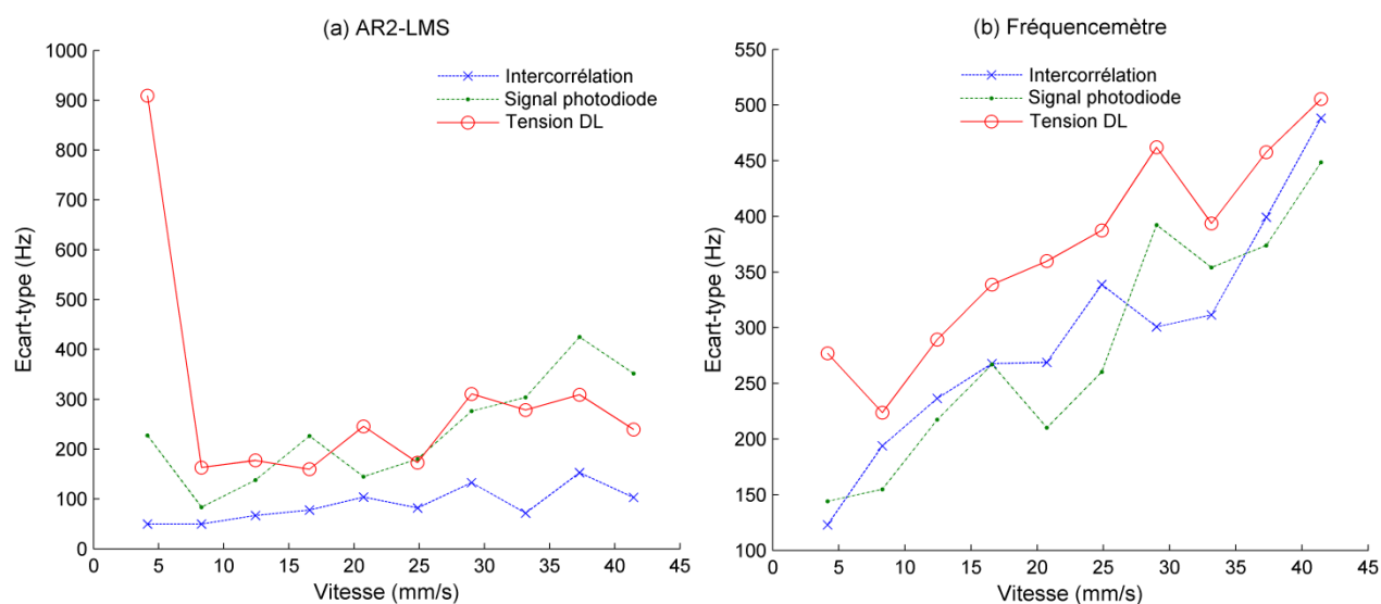
Figure IV-10. Ecart-type des estimations de fréquence Doppler par (a) l'AR2-LMS et (b) le fréquencesmètre. Les signaux de tension et de photodiode ont été filtrés par un filtre passe-bande.
