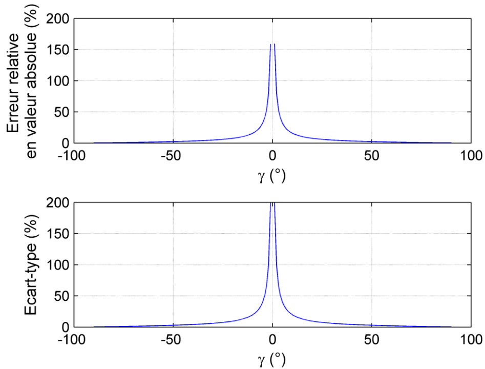
Figure II-6. Représentation des résultats de l'analyse d'incertitude qui sont l'erreur relative par rapport à la valeur exacte et l'écart-type de \tilde{V}_T . V_T = 1 m/s, \sigma_{FD} = 0,5/100 \cdot F_D , \sigma_{\gamma} = 2^{\circ} , -90^{\circ} \leq \gamma \leq 90^{\circ} , N_e = 100\,000 .
