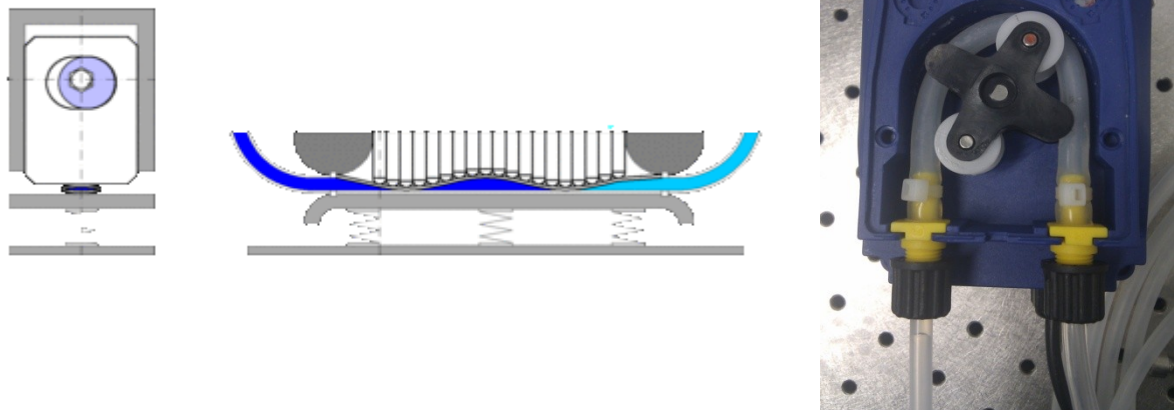
Figure IV-14. Mécanisme de pompe péristaltique.
