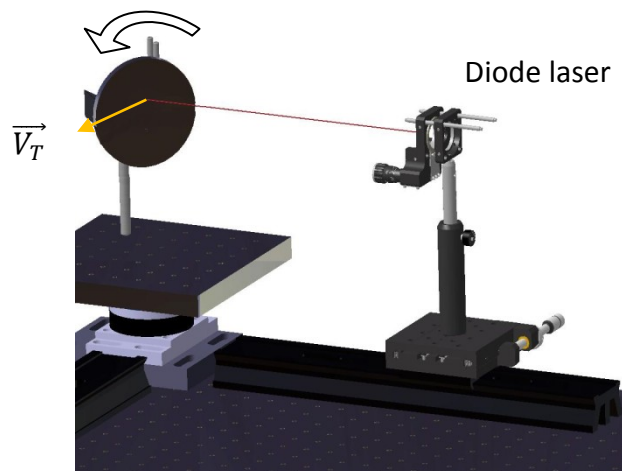
Figure III-28. Schéma représentant le dispositif expérimental. Une diode laser illumine un disque tournant autour de son centre à une vitesse constante. V_T est la vitesse au point illuminé de la cible.
