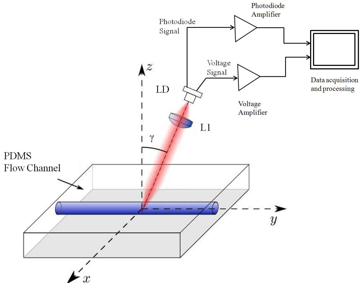
Figure IV-3. Dispositif expérimental micro fluide. \gamma = 11^\circ ; distance focale de L1 = 11mm ; diamètre interne du canal = 320\mu\text{m} ; indice de réfraction du PDMS = 1,4. Le liquide est injecté dans le canal à l'aide d'une pousse seringue avec un contrôle de débit, de marque HARVARD (HARVARD Apparatus PHD 22/2000 Infusion).
