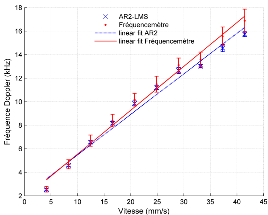
Figure IV-11. Tracé des fréquences Doppler, estimées en appliquant les algorithmes AR2-LMS et fréquencesmètre sur l'intercorrélacion, en fonction de la vitesse d'écoulement. L'intervalle de confiance de 95% est présenté. Les signaux de tension et de photodiode ont été filtrés par un filtre passe-bande.
