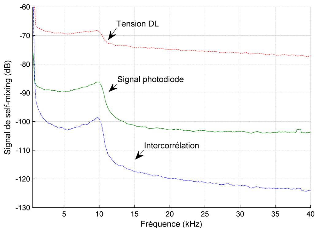
Figure IV-7. Signaux de self-mixing mesurés aux bornes de la jonction laser (DL), à la sortie de la photodiode (PD), et l'intercorrélation de ces deux signaux. Le signal d'intercorrélation présente un meilleur rapport signal sur bruit.
