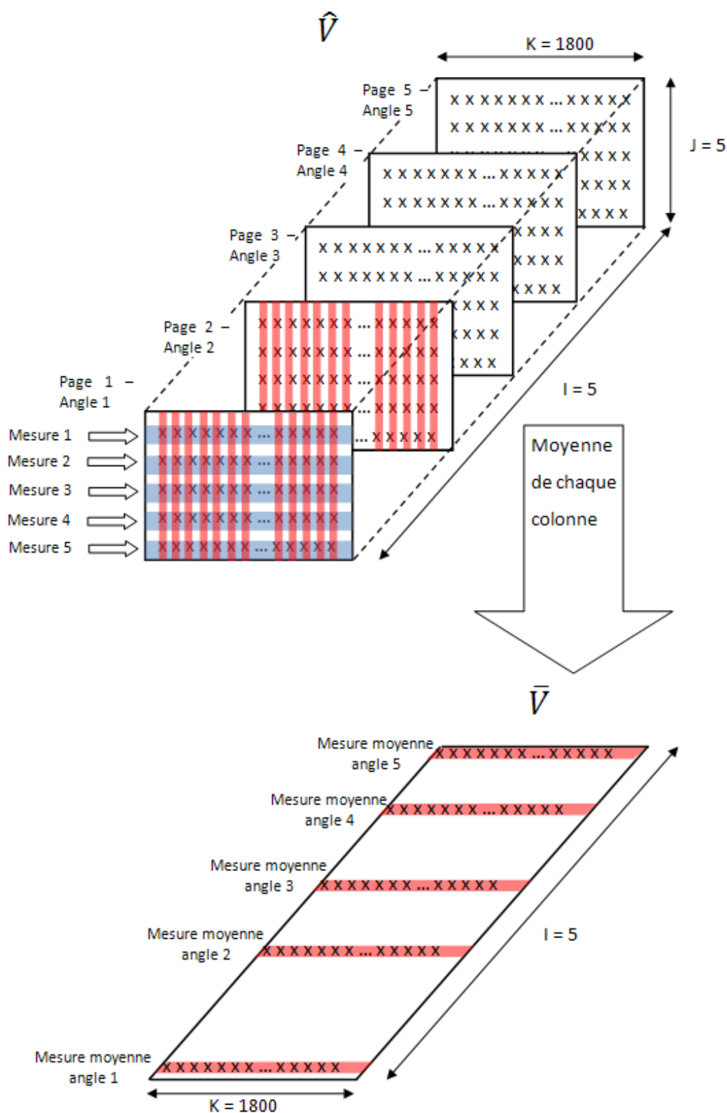
Figure IV-19. Architectures du tableau tridimensionnel contenant les mesures de vitesse et du tableau bidimensionnel contenant les valeurs moyennes de vitesse.
