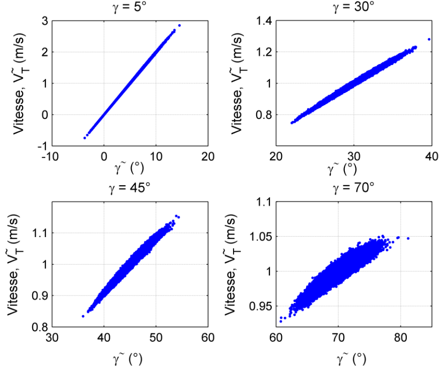
Figure II-4. Diagrammes de dispersion du résultat \tilde{V}_T de l'analyse d'incertitude et sensibilité par la méthode de Monte Carlo. V_T = 1 \text{ m/s} , \sigma_{FD} = 0,5/100 \cdot F_D , \sigma_\gamma = 2^\circ , \gamma = 5, 30, 45 et 70^\circ , N_e = 100\,000 .
