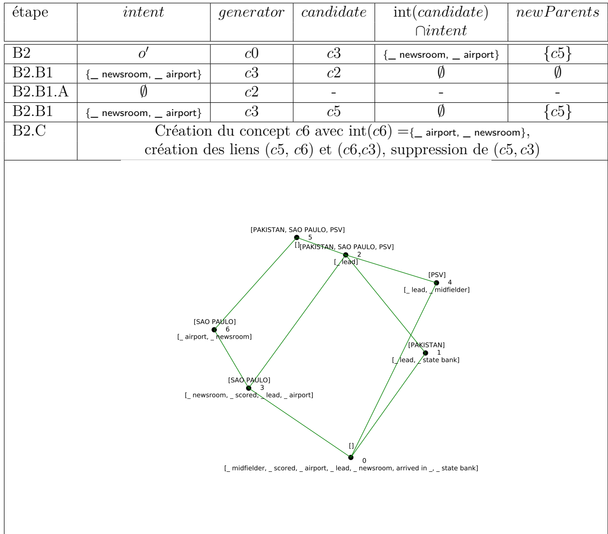
FIG. 2.9 – Ajout de l'objet o = \text{BELGRADE} : évolution du treillis et trace des variables manipulées par l'algorithme lors de la création du concept c6
