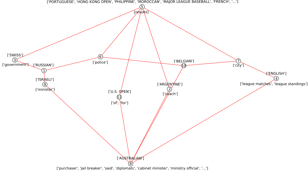
FIG. 3.2 – Sous-treillis des concepts contenant la relation ( Australian , results )
