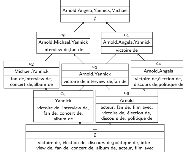
FIG. 1.7 – Treillis de Galois associé à un contexte formel (cf. figure 1.1)
