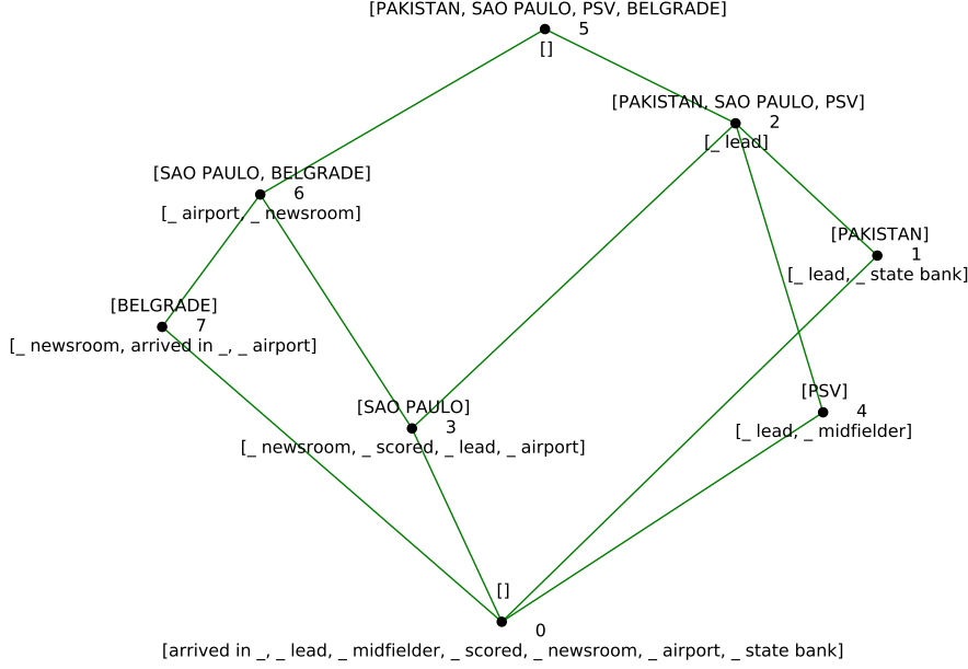
FIG. 2.7 – Modification du treillis de la figure 2.6 suite à l'intégration de l'objet o = \text{BELGRADE} avec ses attributs o' = \{\_airport, arrived\ in\ \_, \_newsroom\}
