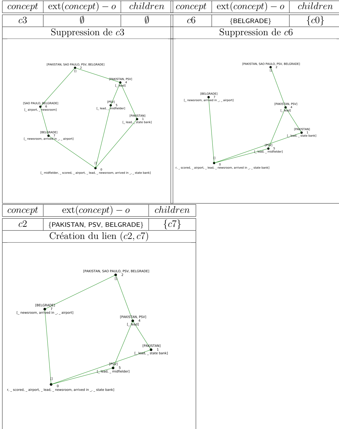
FIG. 2.12 – Suppression de l'objet o = \text{SAO PAULO} : évolution du treillis et des variables manipulées par l'algorithme 4 lors de la suppression du concept c3 (en haut, à gauche), de la suppression de c6 (en haut, à droite) et de la création du lien ( c2 , c7 ) (en bas, à gauche)
