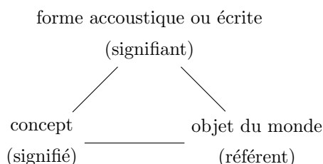
FIG. 1.1 – Représentation du signe linguistique dans un triangle sémiotique
