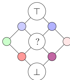
FIG. 5.8 – Treillis de Galois partiellement étiqueté
