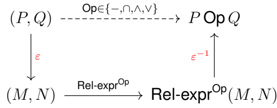
FIGURE 6.3 : Diagramme de l'encodage relationnel
