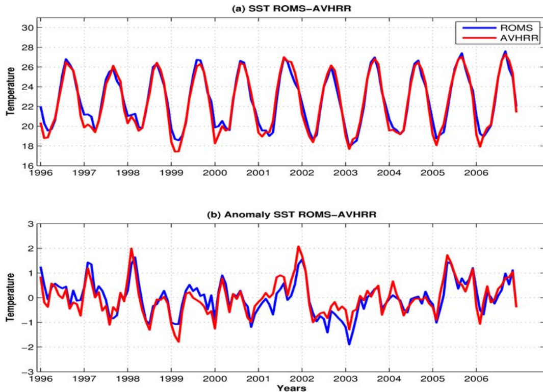
Figure 4.7 – (a) SST mensuelles moyennées entre les latitudes 12°N et 21°N et de la côte à l'isobathe 200m pour ROMS (bleu) et les observations satellites AVHRR (rouge). (b) Même chose pour l'anomalie du signal de SST.
