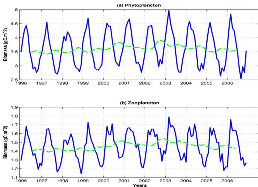
Figure 4.9 – (a) Biomasse de phytoplancton mensuelles intégrée sur les 60 premiers mètres et entre les latitudes 12° et 21°N et de la côte à l'isobathe 200m pour le modèle ROMS-PISCES (en bleu). (b) Même chose pour le zooplancton (en bleu). Les lignes vertes tiretées correspondent à la moyenne glissante sur 12 mois des biomasses calculées.
