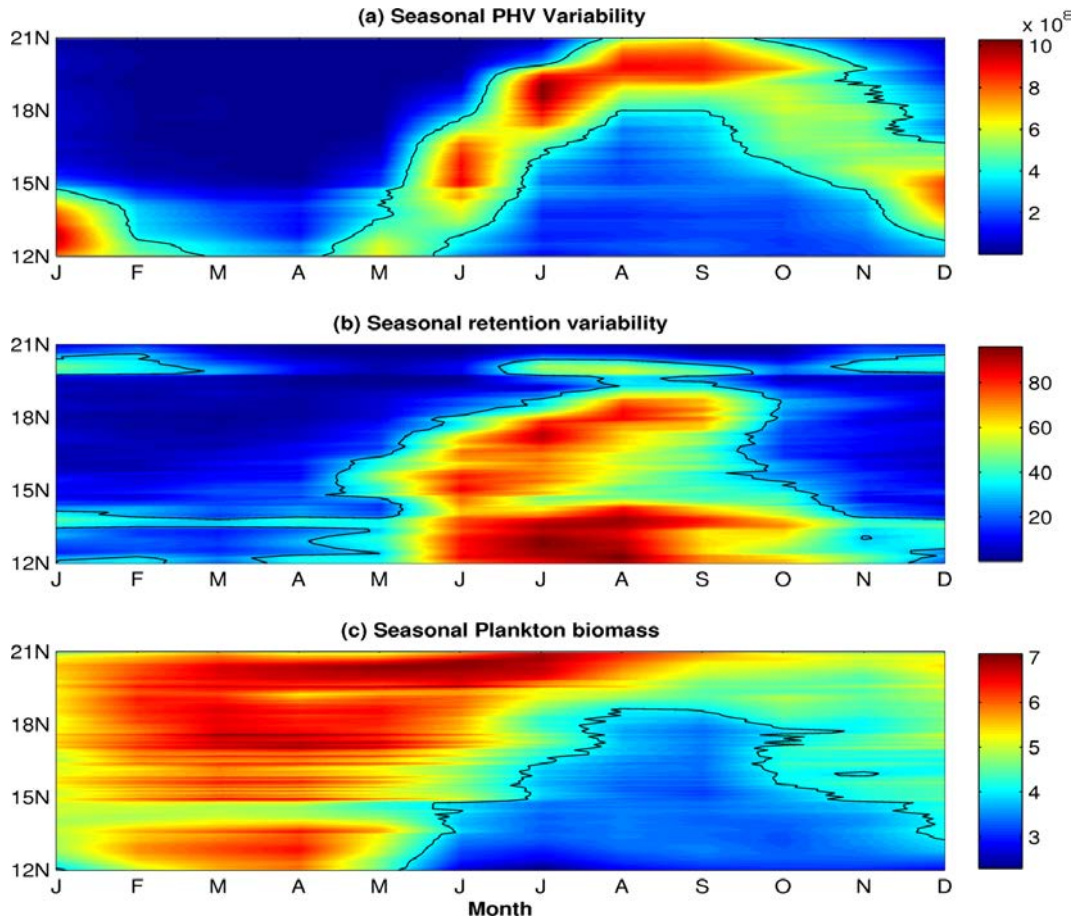
Figure 4.13 – Diagramme Latitude \times Temps du (a) volume d'habitat potentiel ( m^3 ), de la (b) rétention (%) et de la biomasse totale de plancton ( g.C.m^{-2} ) moyennée dans la zone sénégal-mauritanienne.
