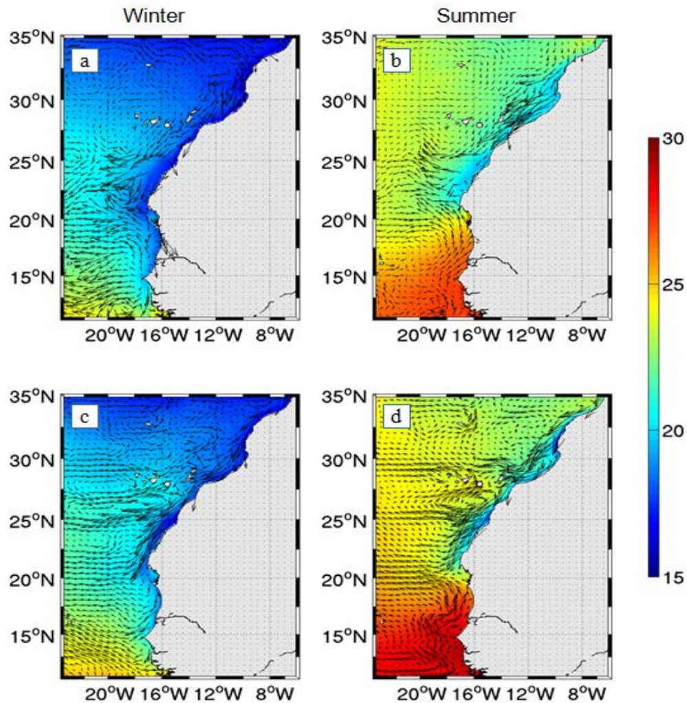
Figure 4.4 – 4 Moyenne saisonnière de la température de surface de la mer (SST) (1985-2009) pour les données satellites AVHRR (a,b) et pour le modèle ROMS (c,d). Les vecteurs correspondent au courants de surface issus du Programme Global Drifter (1979- 2013, Lumpkin and Johnson, 2013) (b,d) et pour le modèle ROMS (c,d) : en hiver (à gauche) et en été (à droite). Tirée de Auger et al. (2015).
