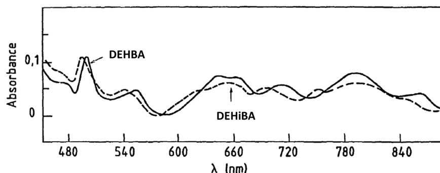
(a) Plutonium(IV) extrait par une phase de DEHBA ( 1,45 \text{ mol.L}^{-1} ) et DEHiBA (pur) à partir d'une phase aqueuse ( [\text{HNO}_3] = 1 \text{ mol.L}^{-1} ).
