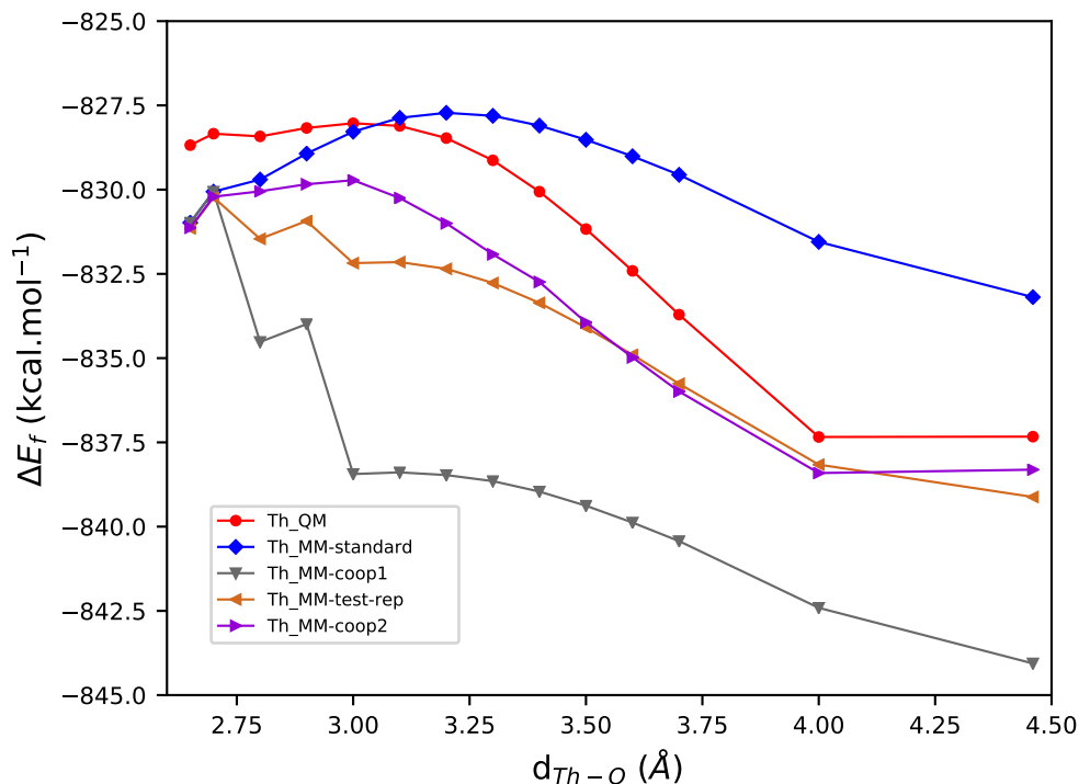
FIGURE 51 – Potentiel de dissociation relaxée de Th^{IV}(H_2O)_{10} : comparaison entre les résultats QM et les différents modèles MM considérés
