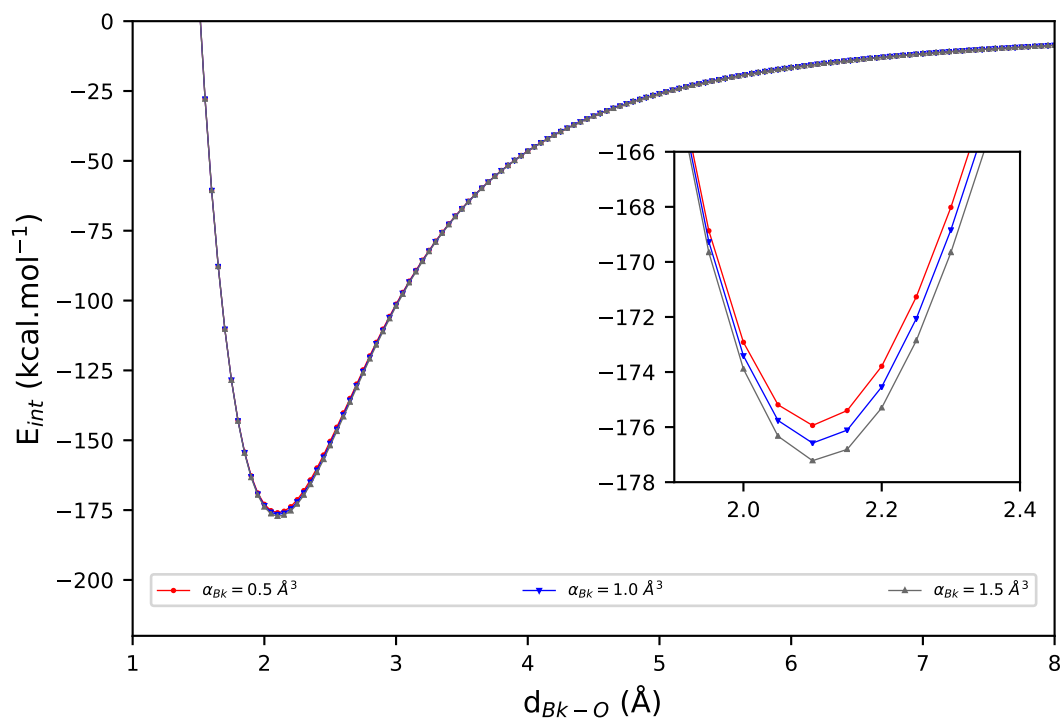
FIGURE 56 – Courbe d'interaction de paire \text{Bk}^{4+} - \text{H}_2\text{O} pour différentes valeurs de polarisabilité de \text{Bk}^{4+}
