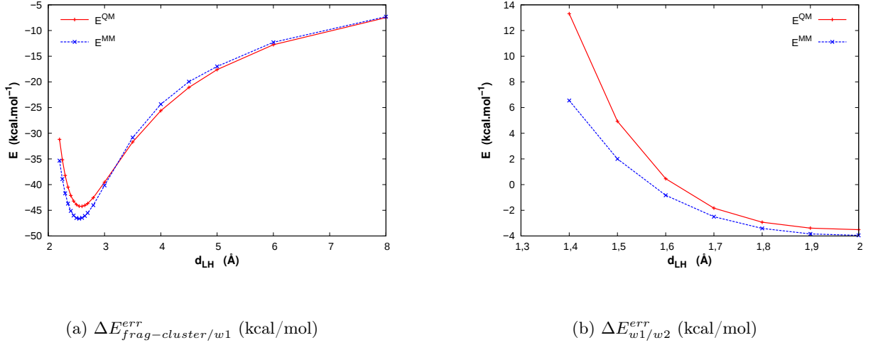
FIGURE 48 – Caractérisation des erreurs dans les cas des interactions sans coopération
