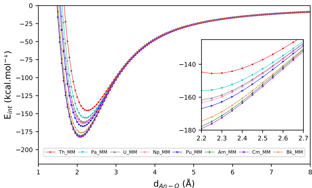
FIGURE 32 – Interaction de paire An^{IV} - H_2O
