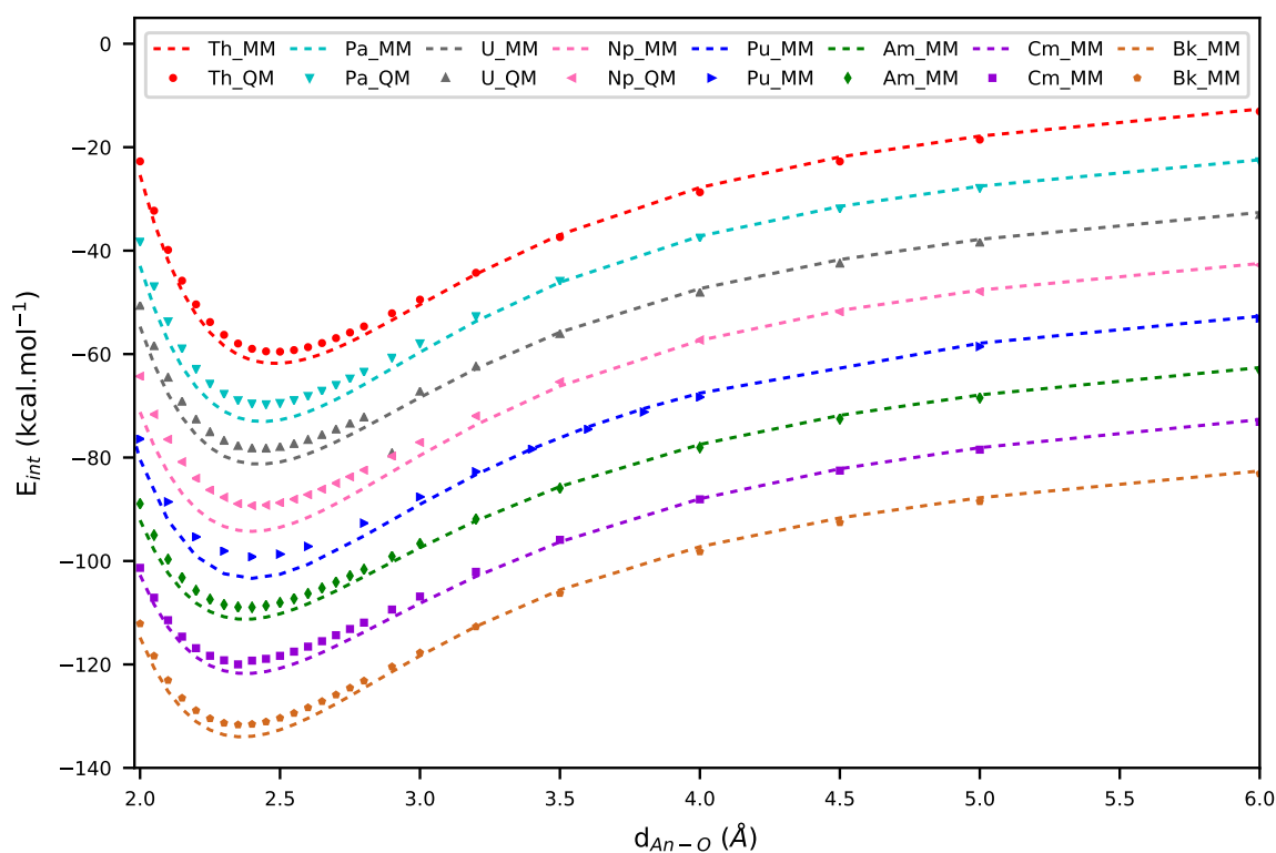
FIGURE 55 – Courbes de dissociation d’une molécule d’eau d’un cluster An^{IV}(\text{H}_2\text{O})_8 : comparaison QM et MM. Les énergies d’interaction entre la molécule d’eau dissociée et le cluster restant sont reportées et décalées en énergie pour plus de clarté. La courbe MM correspond au jeu de paramètres retenus pour le potentiel final.
