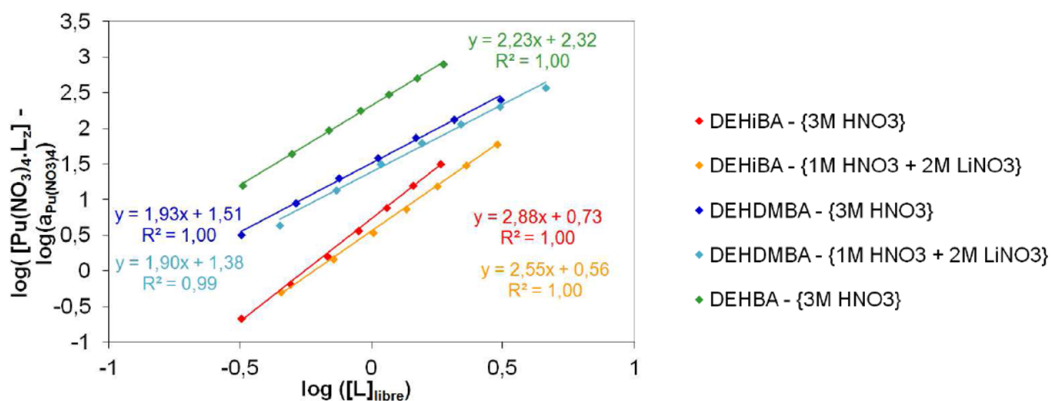
FIGURE 8 – Extraction du nitrate de plutonium par des solutions de DEHBA, DEHDMBA, DEHiBA en fonction de la concentration en extractant. Hypothèse retenue pour l'extraction d'acide nitrique : \{L(\text{HNO}_3), L_2(\text{HNO}_3), L(\text{HNO}_3)_2\} . Phase aqueuse : \{\text{Pu}(\text{NO}_3)_4 \cdot 10^{-4} \text{ mol.L}^{-1} + \text{HNO}_3\} . Phase organique : solution de dialkylamide dans le dodécane pré-équilibrée. Figure reproduite du travail de F. Rodrigues [22].
