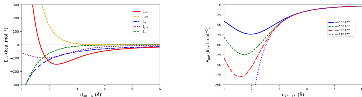
(a) Décomposition (classique) du potentiel de paire \text{An}^{\text{IV}}\text{-H}_2\text{O}
