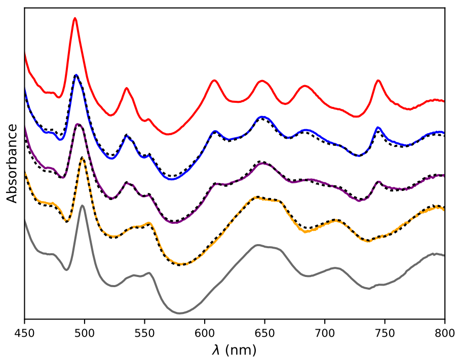
FIGURE 21 – Spectres UV-visible d’une phase organique {Pu-DEHBA} après extraction pour différentes concentrations [\text{HNO}_3]_{\text{aq}} = \{2,8; 3,3; 5; 8; 11\} \text{ mol.L}^{-1} . Les concentrations en extractant utilisées sont respectivement [\text{L}]_{\text{org}} = \{1; 1,2; \text{pur}; \text{pur}; \text{pur}\} \text{ mol.L}^{-1} . Les courbes en pointillés sont les ajustements des spectres réalisés par combinaison linéaire des spectres extrêmes obtenus à [\text{HNO}_3]_{\text{aq}} = 2,8 et 11 \text{ mol.L}^{-1} .
