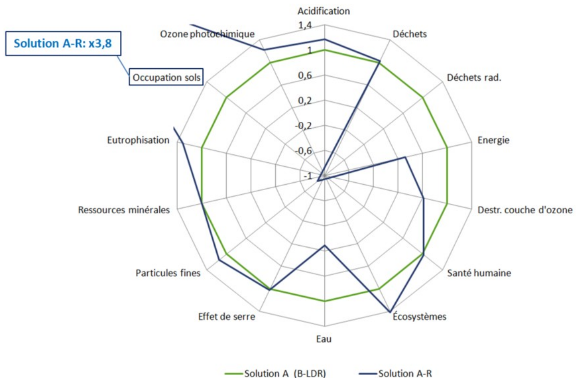
Figure 5.17 – Comparaison des impacts en ACV des solutions A initiale et A-R
