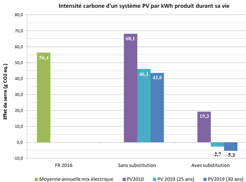
Figure 2.9 – Comparaison de l'intensité carbone d'un kWh produit par un système PV avec différentes hypothèses
