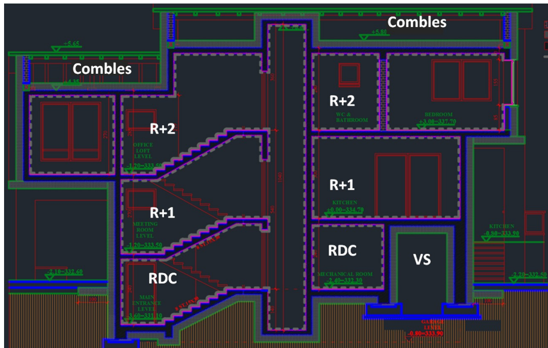
Figure 2.18 - Plan de coupe, visualisation des étages en quinconce. En gris l'épaisseur d'isolant et en noir l'épaisseur de béton (VS = vide-sanitaire).
