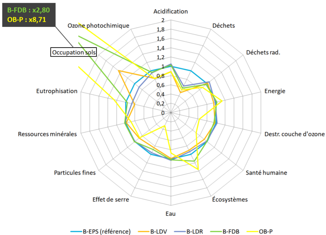
Figure 3.10 – Graphe radar des impacts totaux des variantes du système constructif avec B-EPS comme référence
