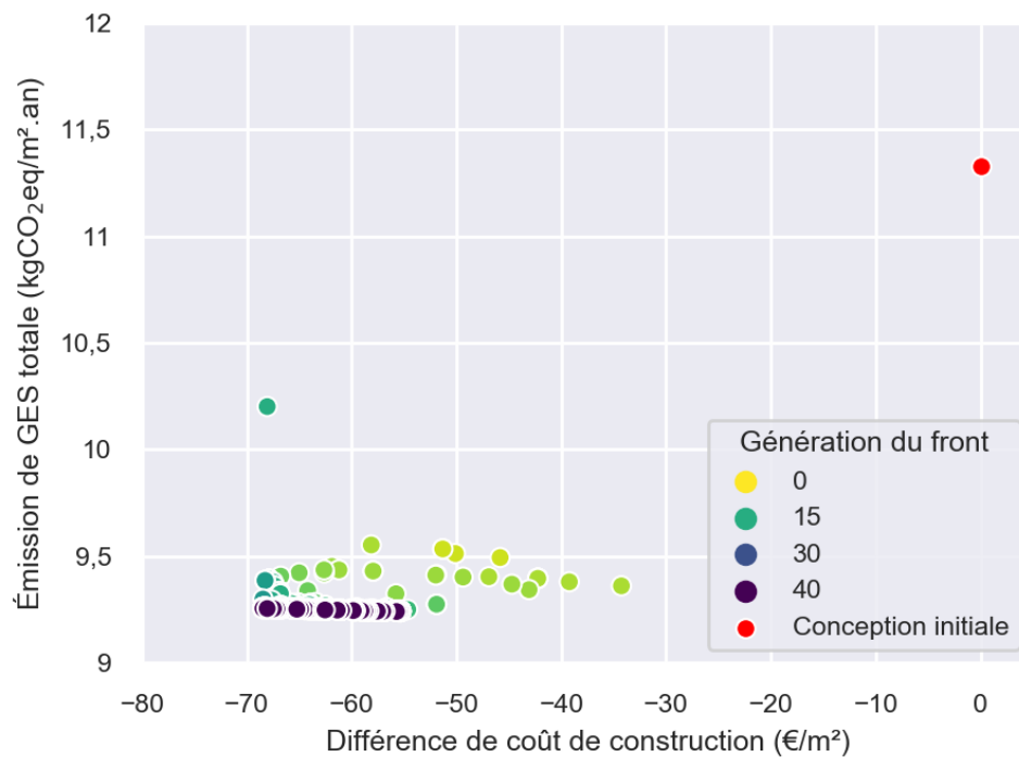
Figure 3.3 – Évolution du front de Pareto du POM simple
