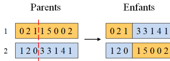
Figure 2.5 – Illustration du croisement à un point de coupure de la représentation du génome en une chaîne d'entiers
