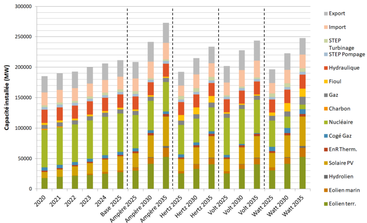
Figure 4.15 – Capacités installées des scénarios des bilans prévisionnels 2017 et 2019 de RTE
