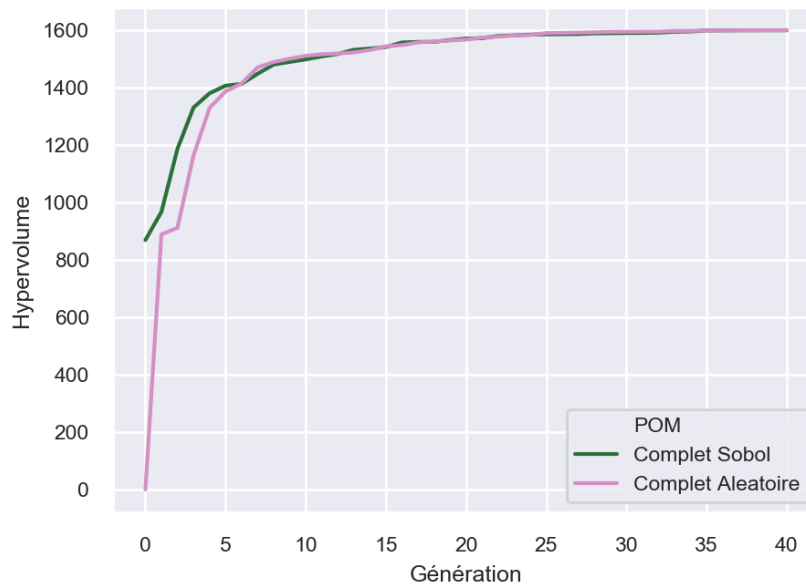
Figure 3.15 – Évolution de l'hypervolume de trois POM
