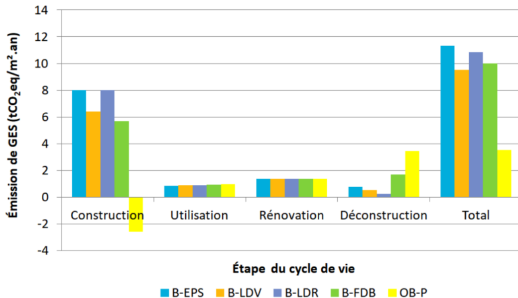
Figure 3.11 – Émission de GES par étape du cycle de vie des variantes du système constructif
