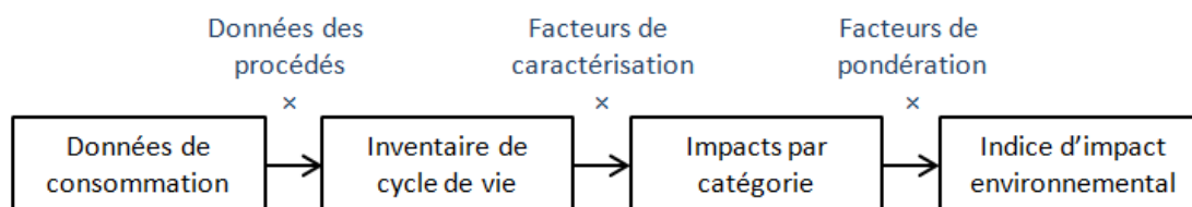
Figure 1.10 – Étapes de l'ACV de bâtiment
