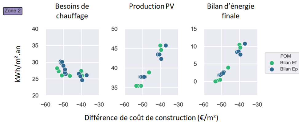
Figure 3.36 – Comparaisons de la zone 2 des POM avec bilan Ef et avec bilan Ep
