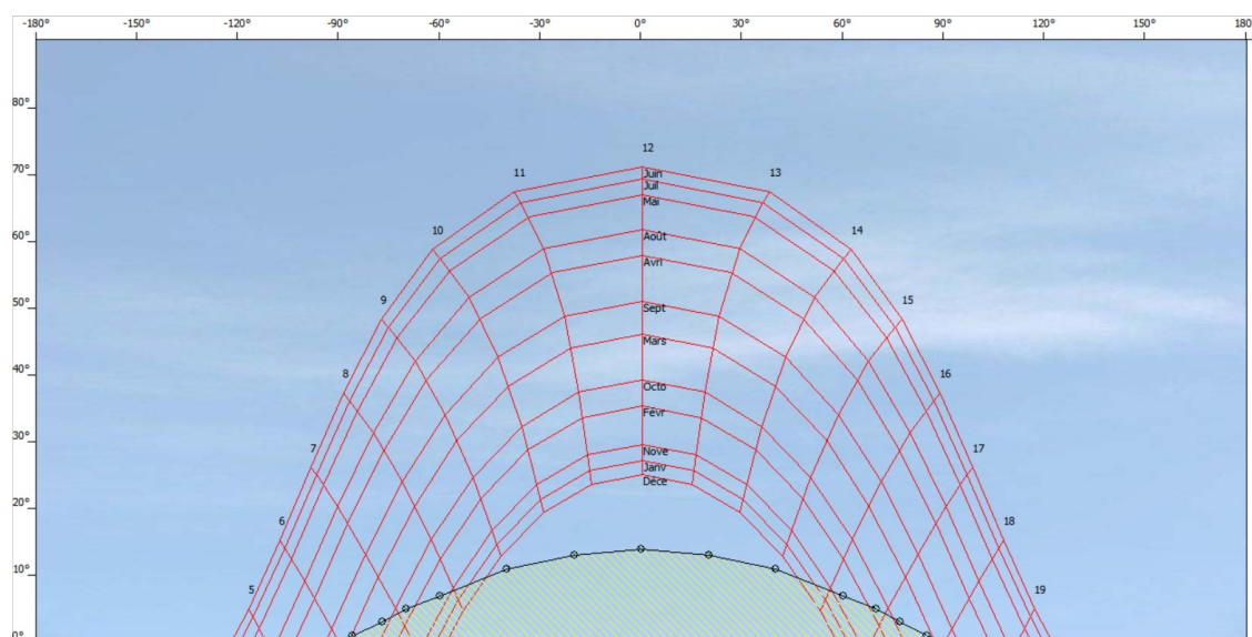
Figure 2.17 – Masque solaire vu depuis la façade Sud
