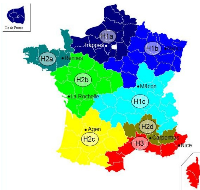
Figure 4.3 – Zones climatiques dans la réglementation thermique 2012 (RT2012)
