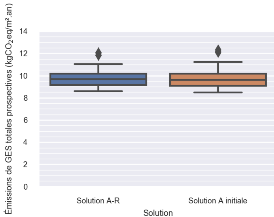
Figure 5.15 – Boîtes à moustache des émissions de GES totales prospectives pour les solutions A-R et A initiale
