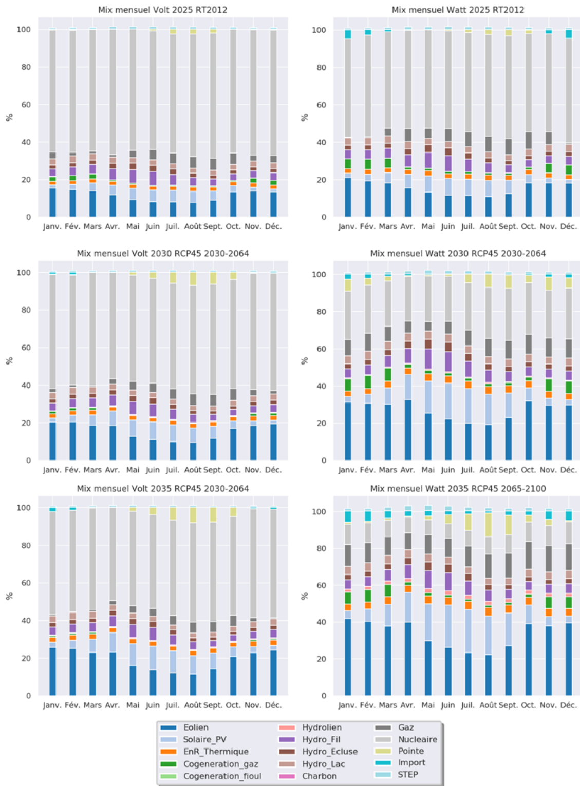
Figure 4.22 – Mix mensuels des scénarios Volt et Watt issus du modèle
