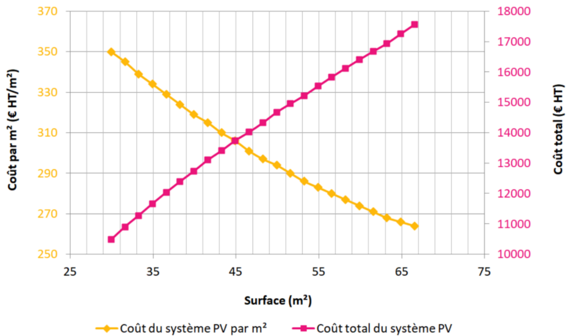
Figure 3.2 – Coûts d'un système PV d'une puissance de 150Wc/m²
