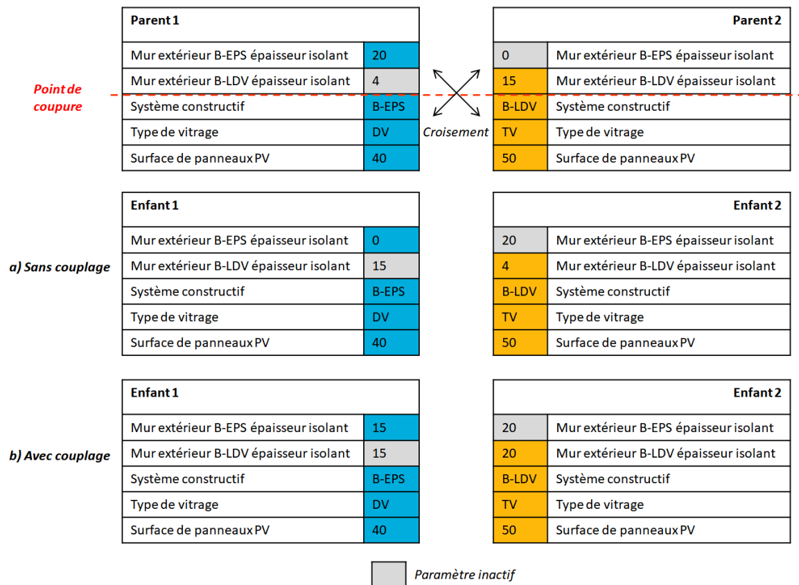
Figure 3.12 – Illustration de la problématique du couplage des paramètres de conception dans une opération de croisement à un point de coupure
