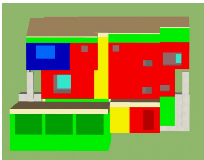
Figure 2.20 - Zonage thermique. Rouge : zone jour, bleu : zone nuit, jaune : LNC étanches, vert : LNC non-étanches
