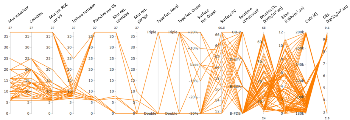
Figure 3.23 – Coordonnées parallèles pour la visualisation des solutions du front de Pareto global
