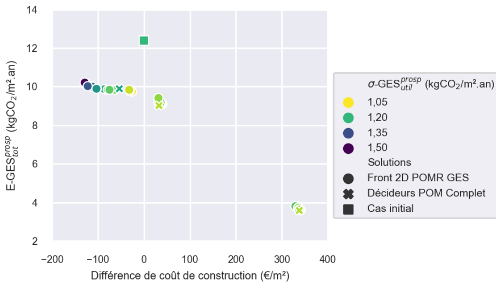
Figure 5.12 – Solutions du front 2D du POMR GES, des décideurs du POM Complet et cas initial dans l'espace des objectifs prospectifs
