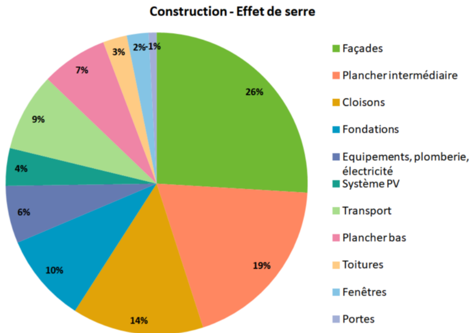
Figure 2.26 – Contributions à l'effet de serre de l'étape de construction
