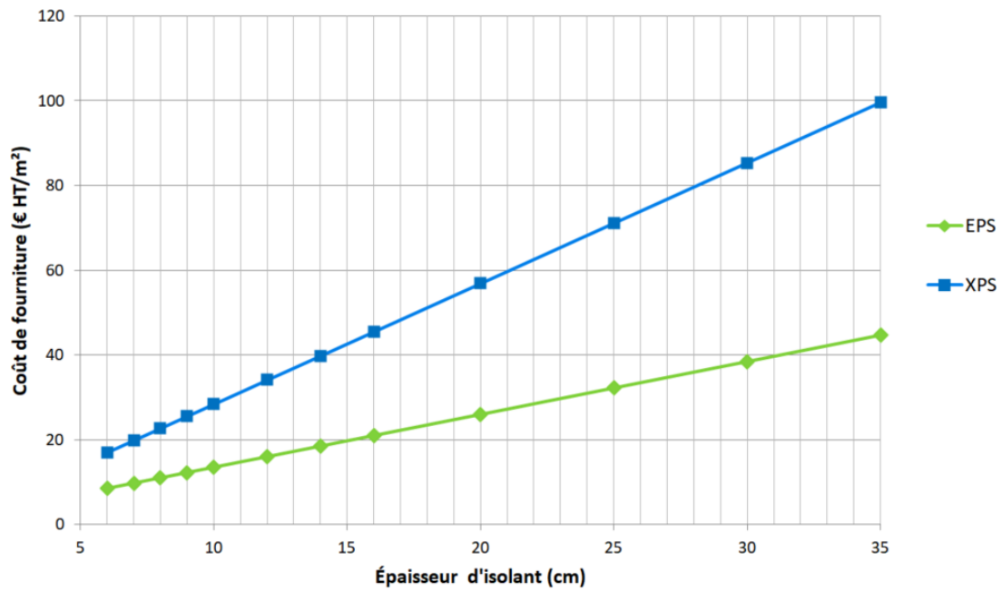
Figure 3.1 – Coût en € HT/m² des isolants en polystyrène en fonction de l'épaisseur
