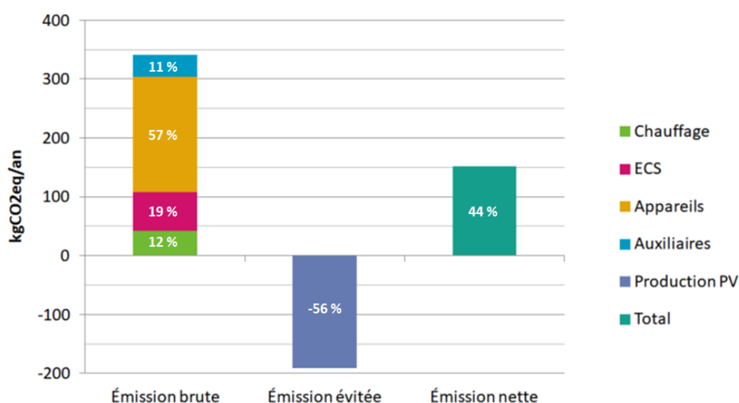
Figure 2.27 – Contribution des postes aux émissions de GES de l'étape d'utilisation
