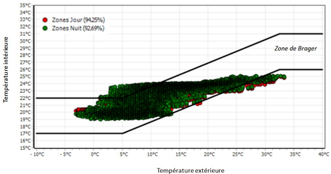
Figure 2.22 - Diagramme de Brager et taux de confort
