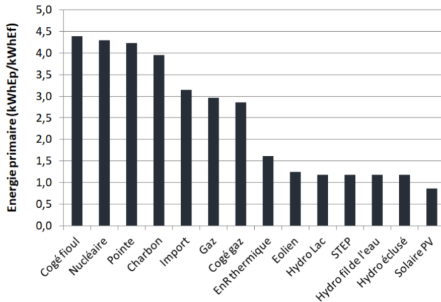
Figure 3.31 – Contenu en énergie primaire d'un kWh d'électricité produit par différentes technologies d'après ecoinvent 3.4 et CED (Hischier et al., 2010)
