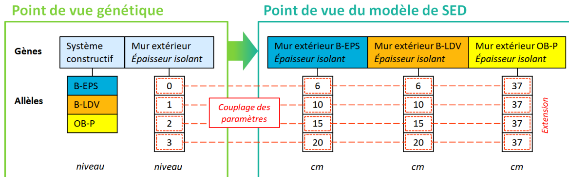
Figure 3.13 – Exemple du couplage de paramètres de conception et de l'extension des allèles associées aux compositions de la variante OB-P
