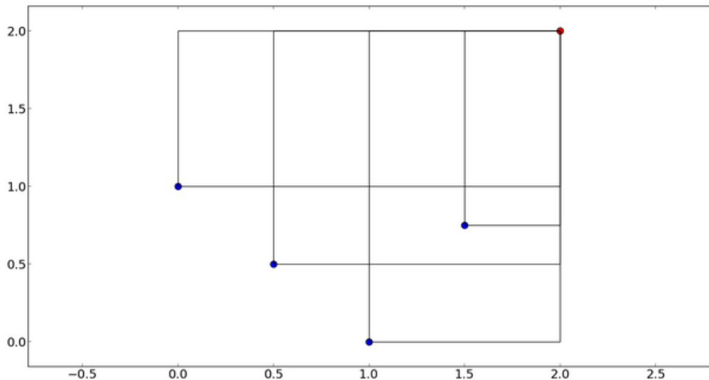
Figure 3.14 – Représentation des hypervolumes exclusifs de solutions (bleu) par rapport à un point de référence (rouge)
