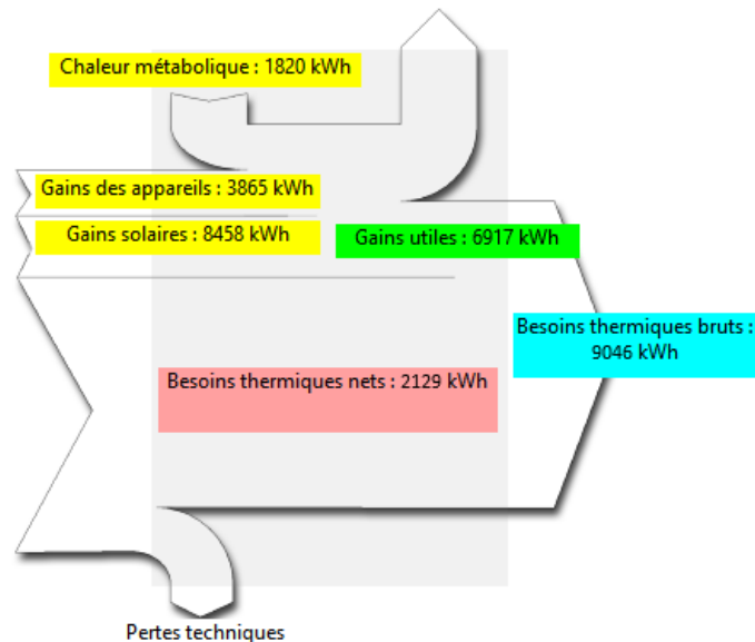
Figure 2.21 - Diagramme de Sankey des besoins chauds de l'enveloppe
