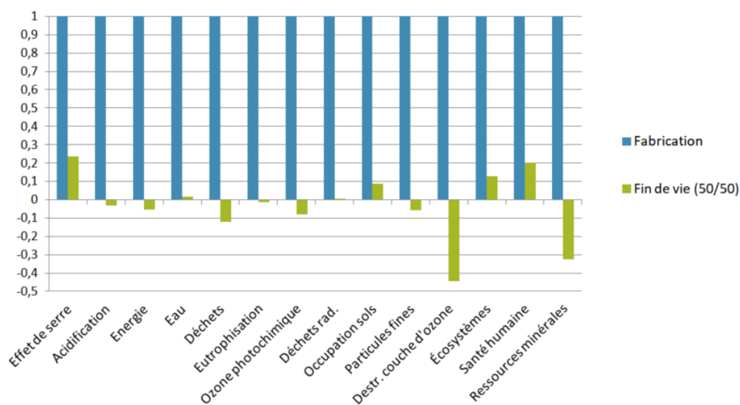
Figure 2.13 – Comparaison des impacts de fabrication et de fin de vie d’une pompe à chaleur. Unité fonctionnelle de 1 kW
