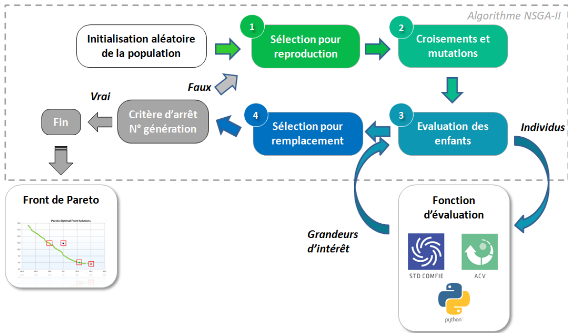
Figure 2.4 – Schéma de fonctionnement de NSGA-II
