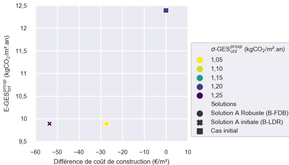
Figure 5.13 – Solution robuste sélectionnée et comparaison avec la solution du POM
