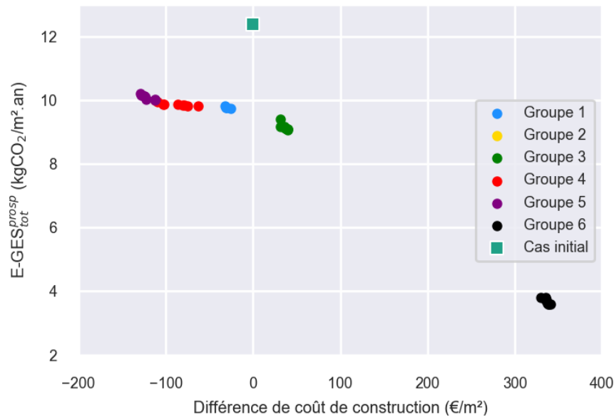
Figure 5.11 – Front à deux dimensions extrait du front de Pareto 3D du POMR GES
