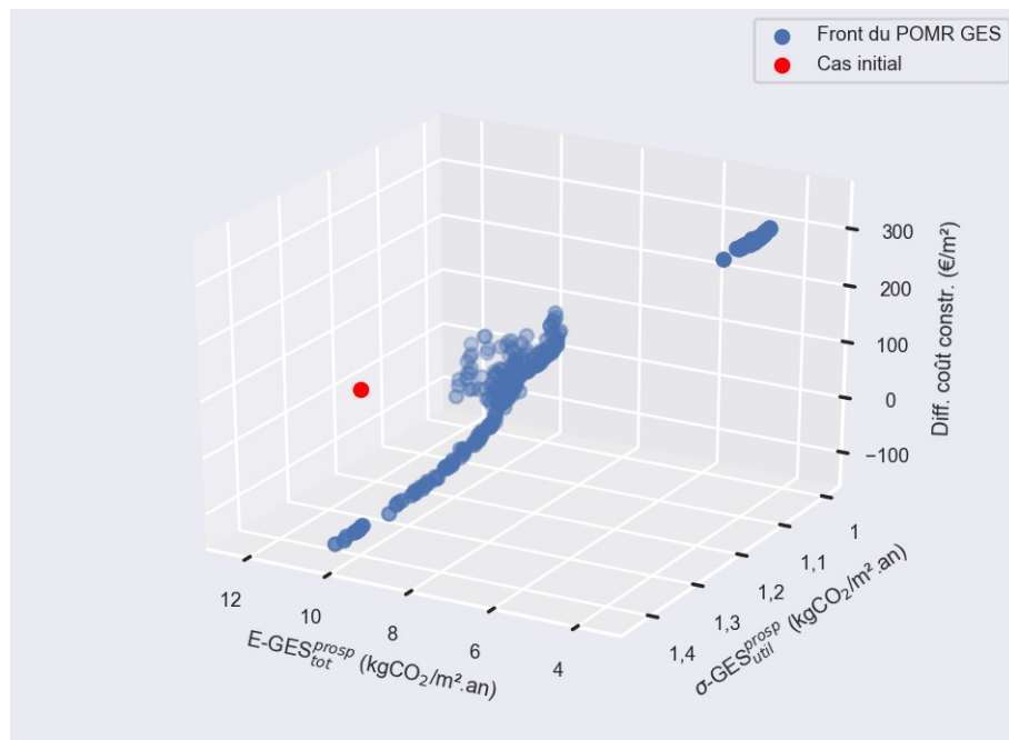
Figure 5.6 – Front de Pareto en 3D du POMR GES
