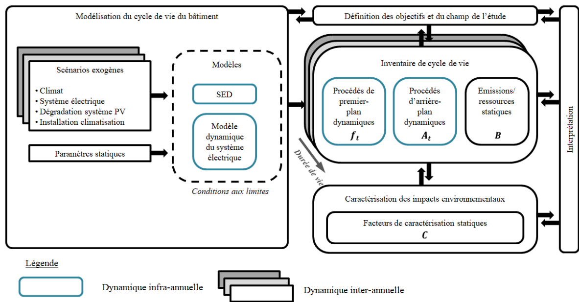
Figure 4.2 – Approche d’ACV prospective du bâtiment illustrée dans le cadre de l’ACV dynamique
