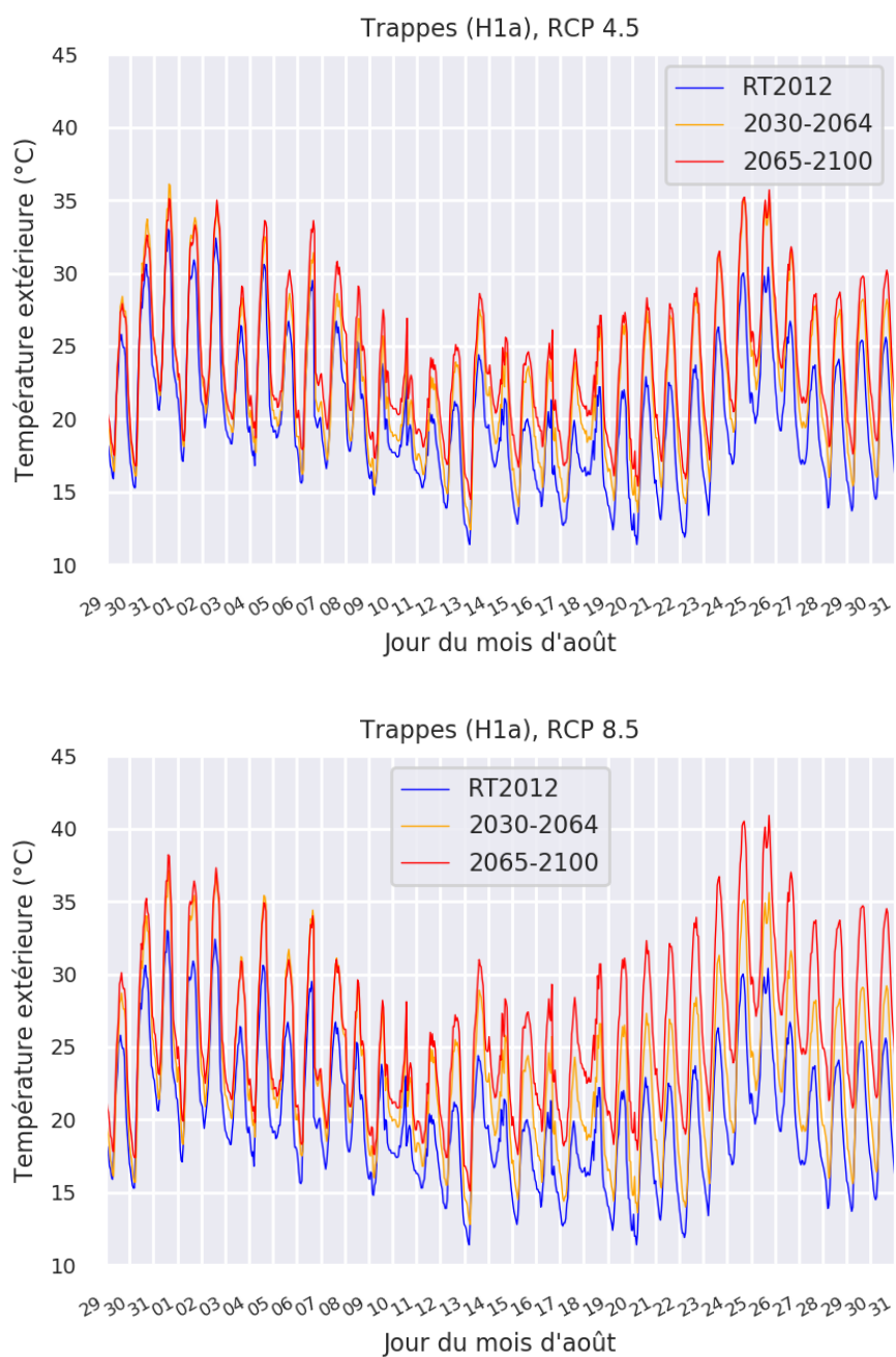
Figure 4.10 – Température extérieure du mois d’août dans les scénarios RCP 4.5 et 8.5
