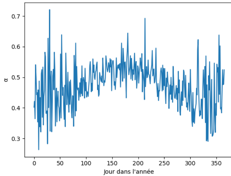
Figure 4.5 – Ratio \alpha sur une année de référence de la période 1982-2018
