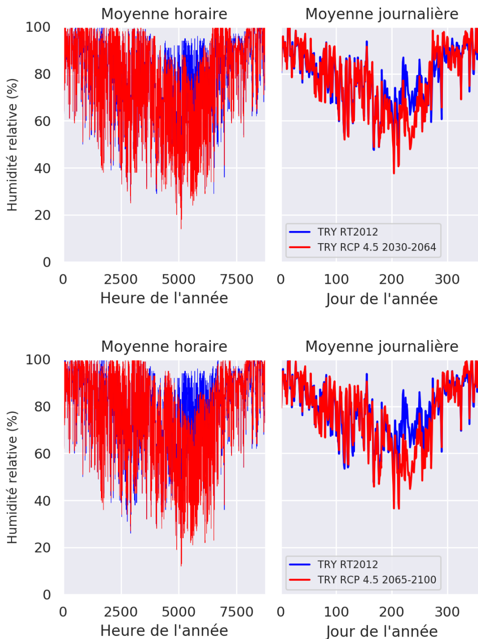
Figure 4.13 – Humidité relative dans les données issues du morphing appliqué à la station de Trappes (H1a), scénario RCP 4.5
