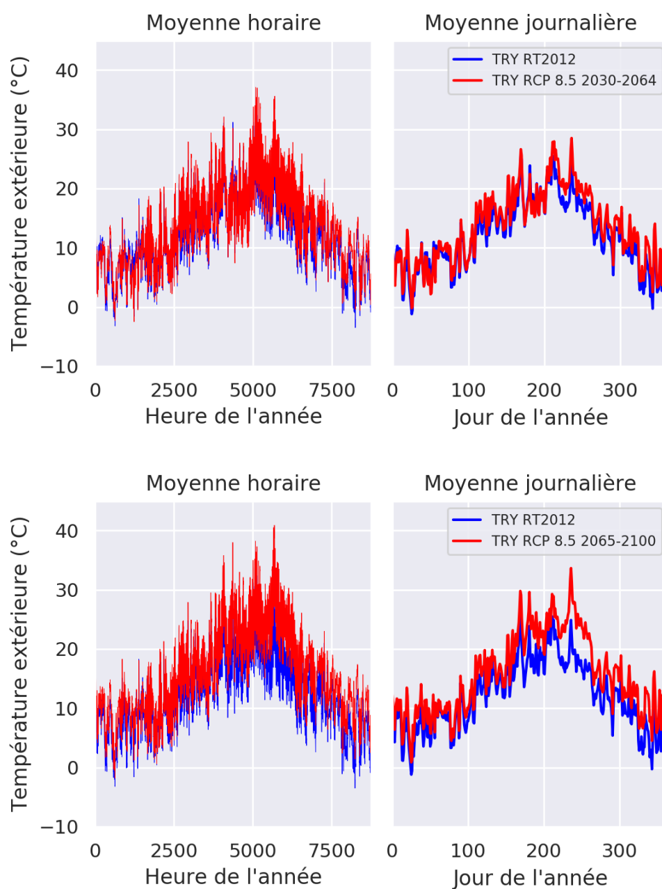
Figure 4.8 – Température extérieure des données issues du morphing appliqué à la station de Trappes (H1a), scénario RCP 8.5
