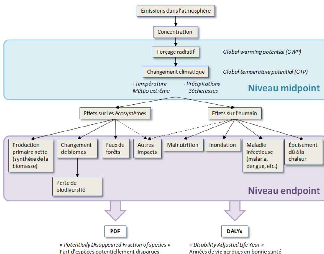
Figure 2.7 – Mécanismes environnementaux du changement climatique. Adapté de European Commission - Joint Research Centre (2011)
