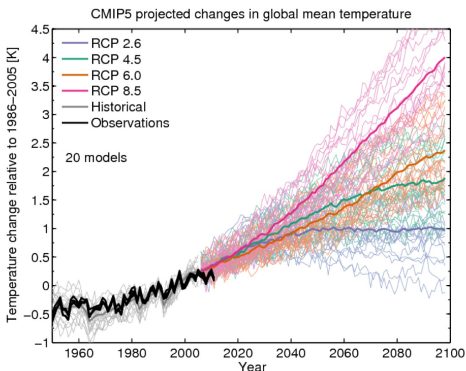
Figure 4.4 – Projection des scénarios RCP sur la différence de température globale avec la période 1986-2005 (source : Ed Hawkins)
