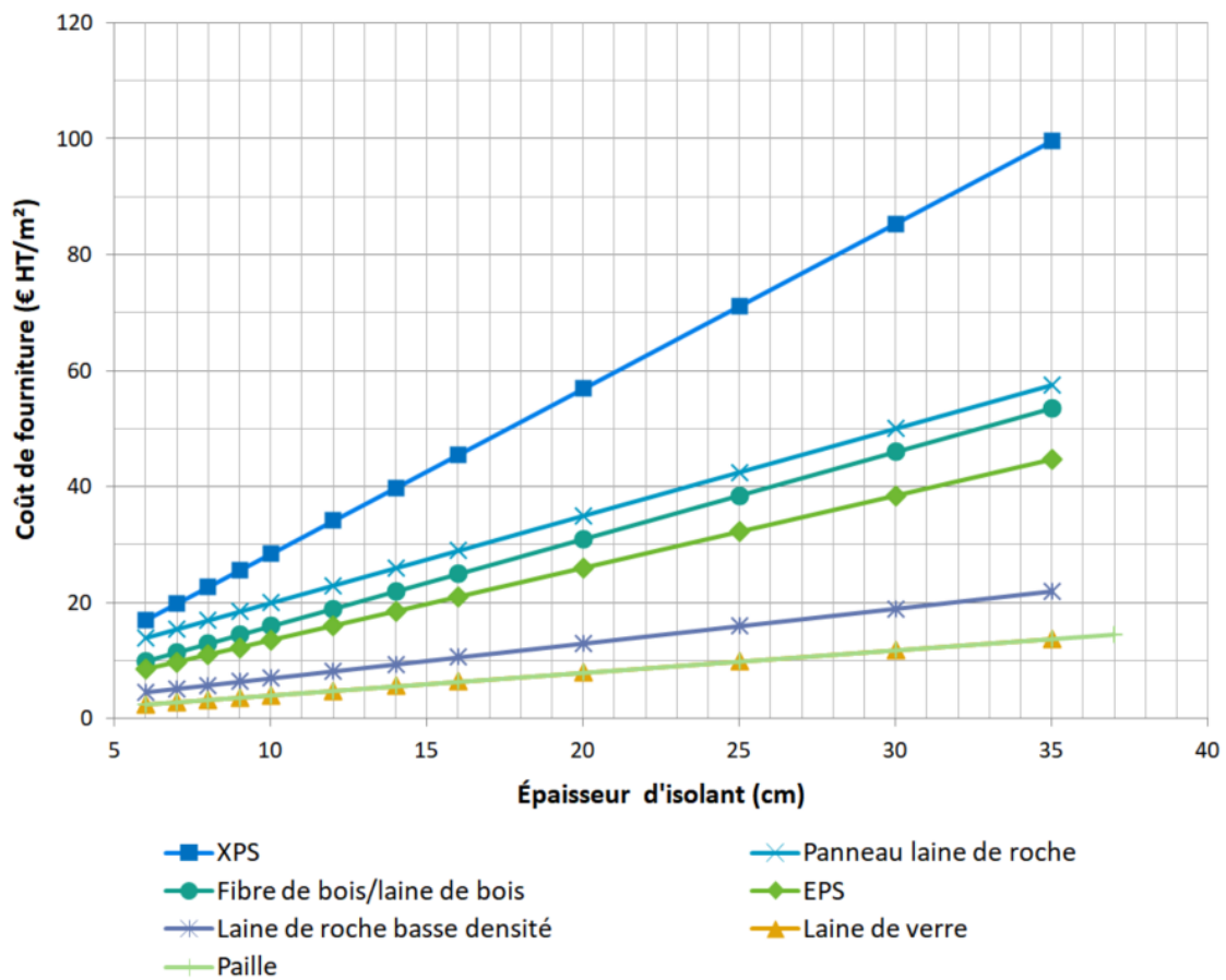
Figure 3.9 – Coûts de fourniture des isolants en € HT/m 2 en fonction de leur épaisseur
