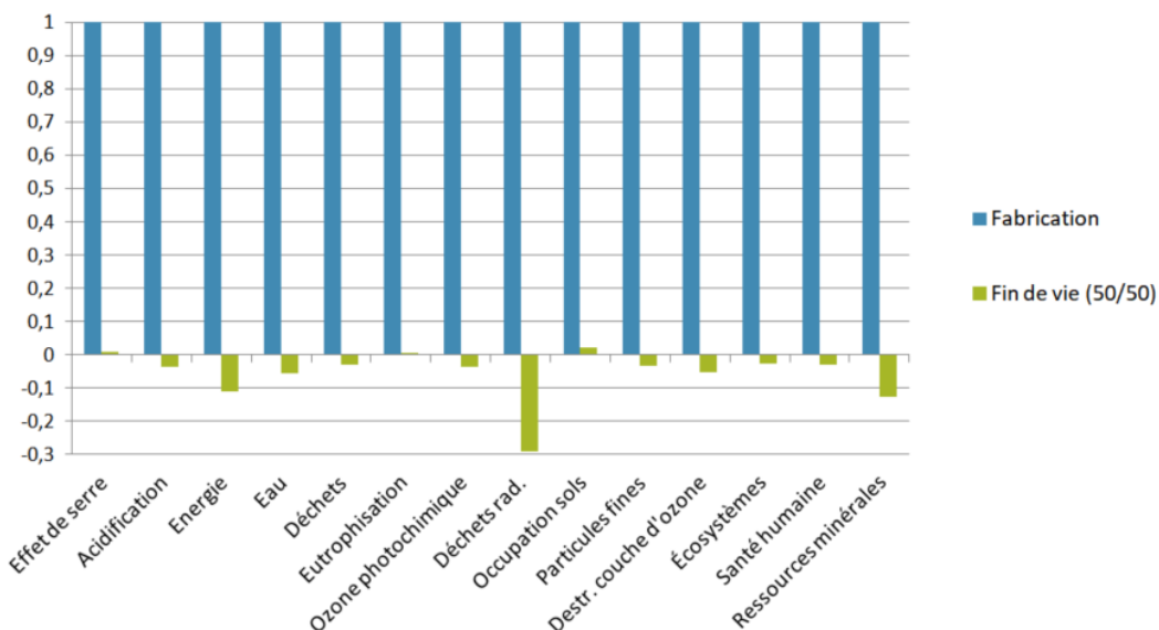
Figure 2.12 – Comparaison des impacts de fabrication et de fin de vie d'un système solaire thermique. Unité fonctionnelle de 1 m 2
