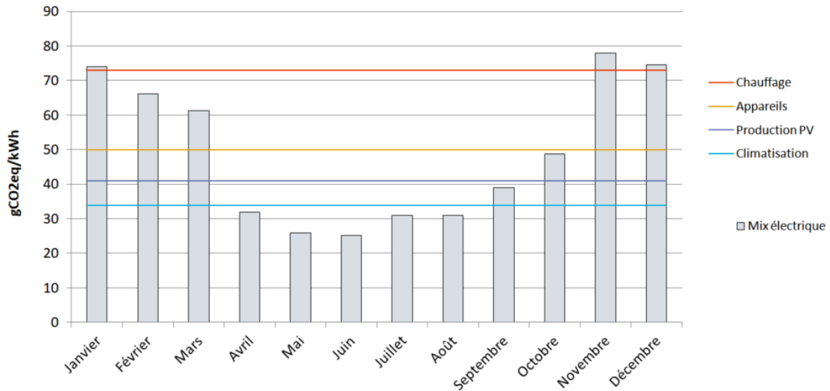
Figure 2.28 – Émission de GES annuelle d'un kWh de différents usages de l'électricité et émission mensuelle d'un kWh provenant du mix électrique (ACV attributionnelle)
