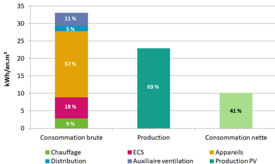
Figure 2.23 – Détails des postes de consommation d'électricité, de la production et de la consommation nette et pourcentages de la consommation brute totale.
