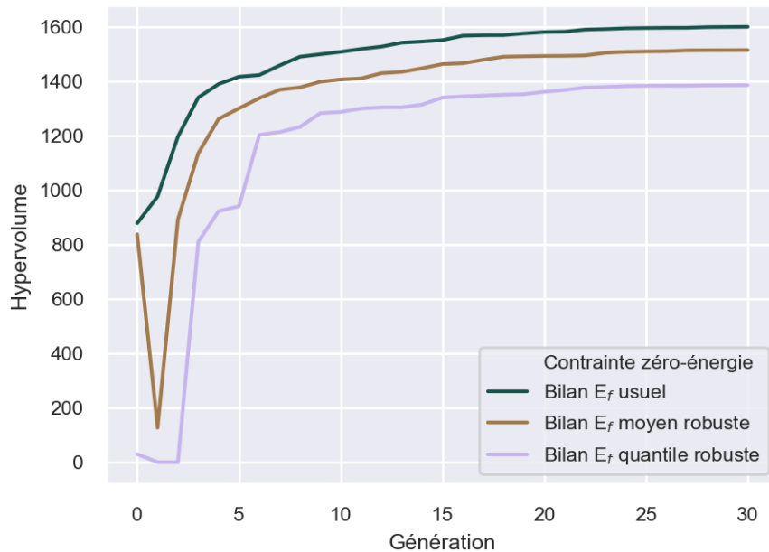
Figure 5.2 – Hypervolumes des POM/POMR avec différentes contraintes zéro-énergie
