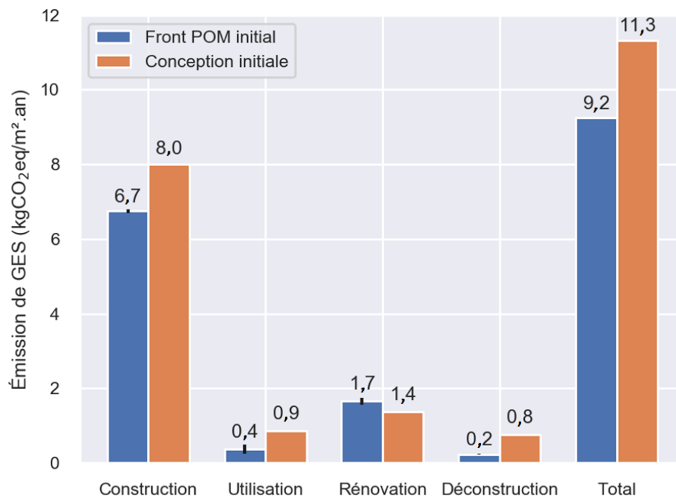
Figure 3.7 – Comparaison des émissions de GES moyennes des solutions optimales avec les émissions de la conception initiale
