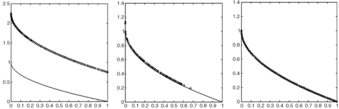
Figure 1.16 – Exemples de fronts de Pareto : mauvaise convergence et bonne diversité (gauche), bonne convergence et mauvaise diversité (centre), bonne convergence et bonne diversité (droite). Source : El-Ghazali Talbi (2009)
