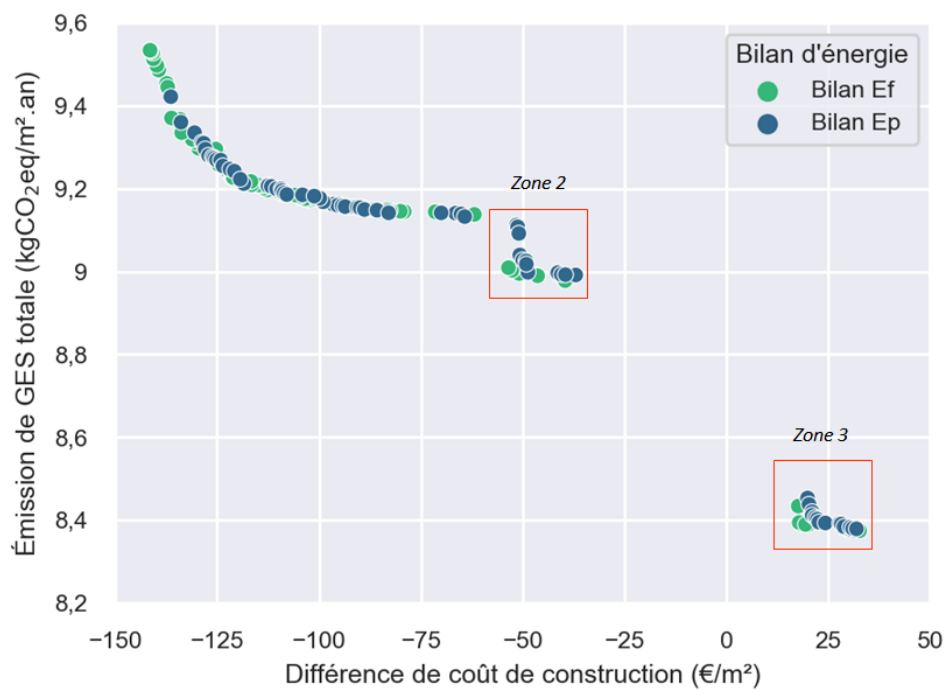
Figure 3.35 – Comparaison des fronts locaux des POM avec bilan Ef et bilan Ep
