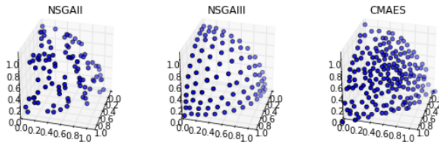
Figure 1.20 - Répartition des solutions des surfaces de Pareto de différents algorithmes d'optimisation pour un problème test DTLZ2 (concave) à 3 fonctions objectif (Hadka – documentation de Platypus)
