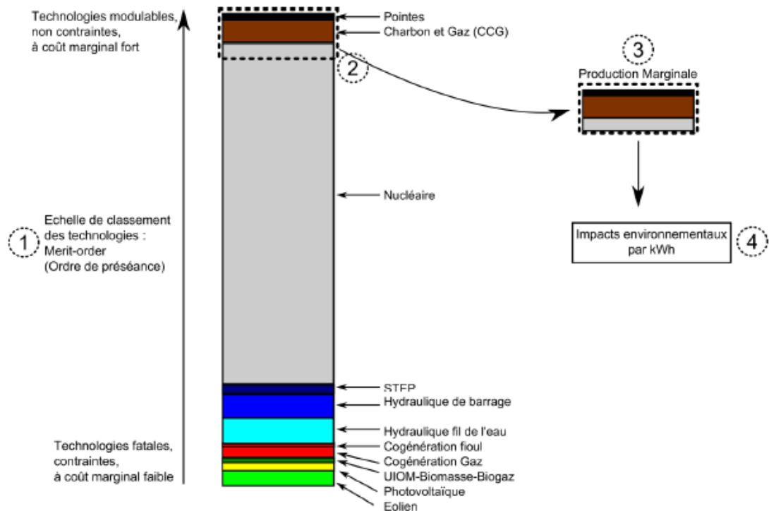
Figure 2.2 – Schéma du principe du mix marginal GHG-P, tiré de Roux (2016)
