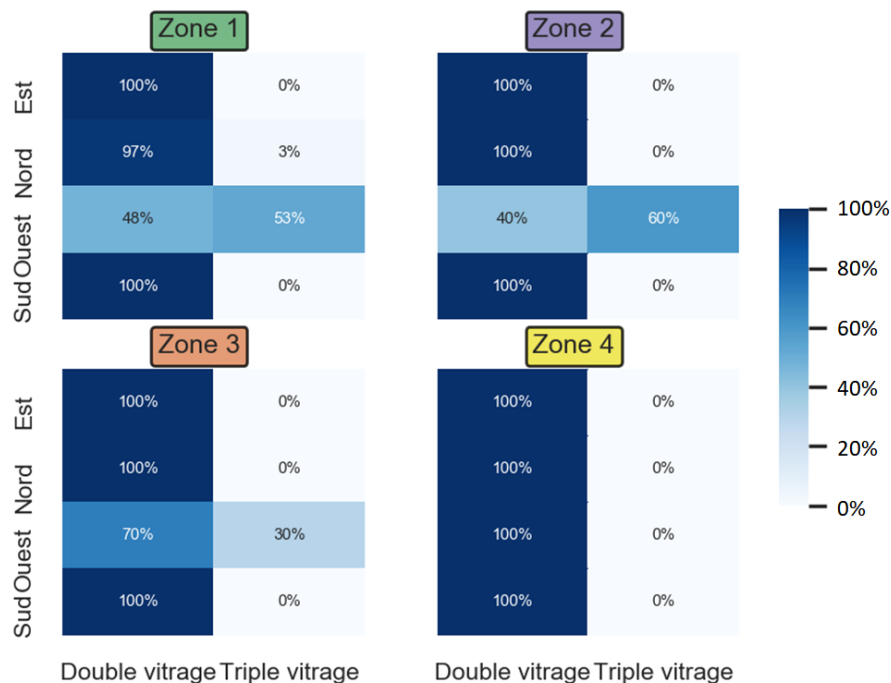
Figure 3.20 – Répartition des types de vitrage parmi les solutions des zones d'optimum local
