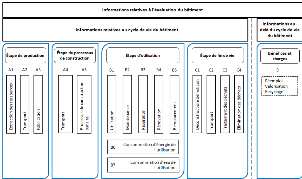
Figure 1.8 – Étapes et modules du cycle de vie d'un bâtiment selon la norme CSN EN 15978:2011
