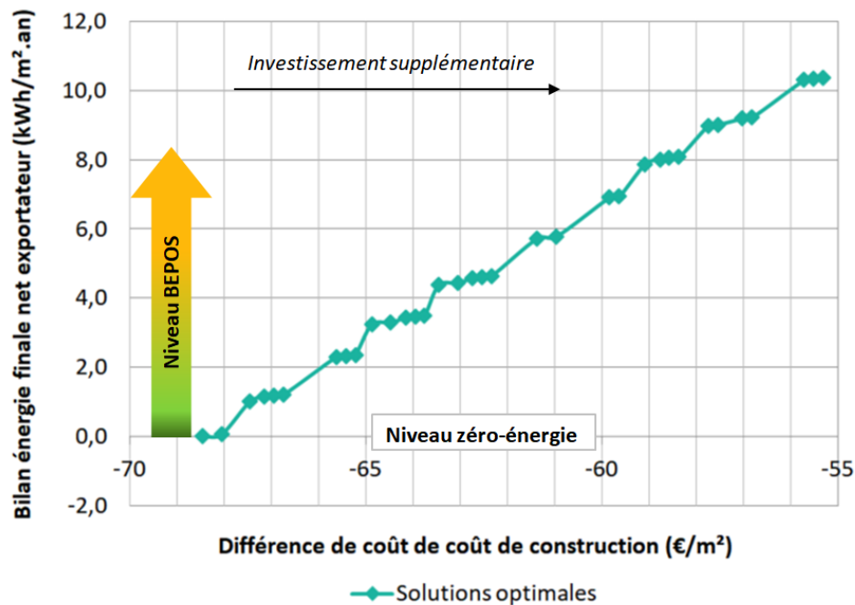
Figure 3.5 – Évolution du bilan d'énergie des solutions optimales du POM simple en fonction du coût de construction
