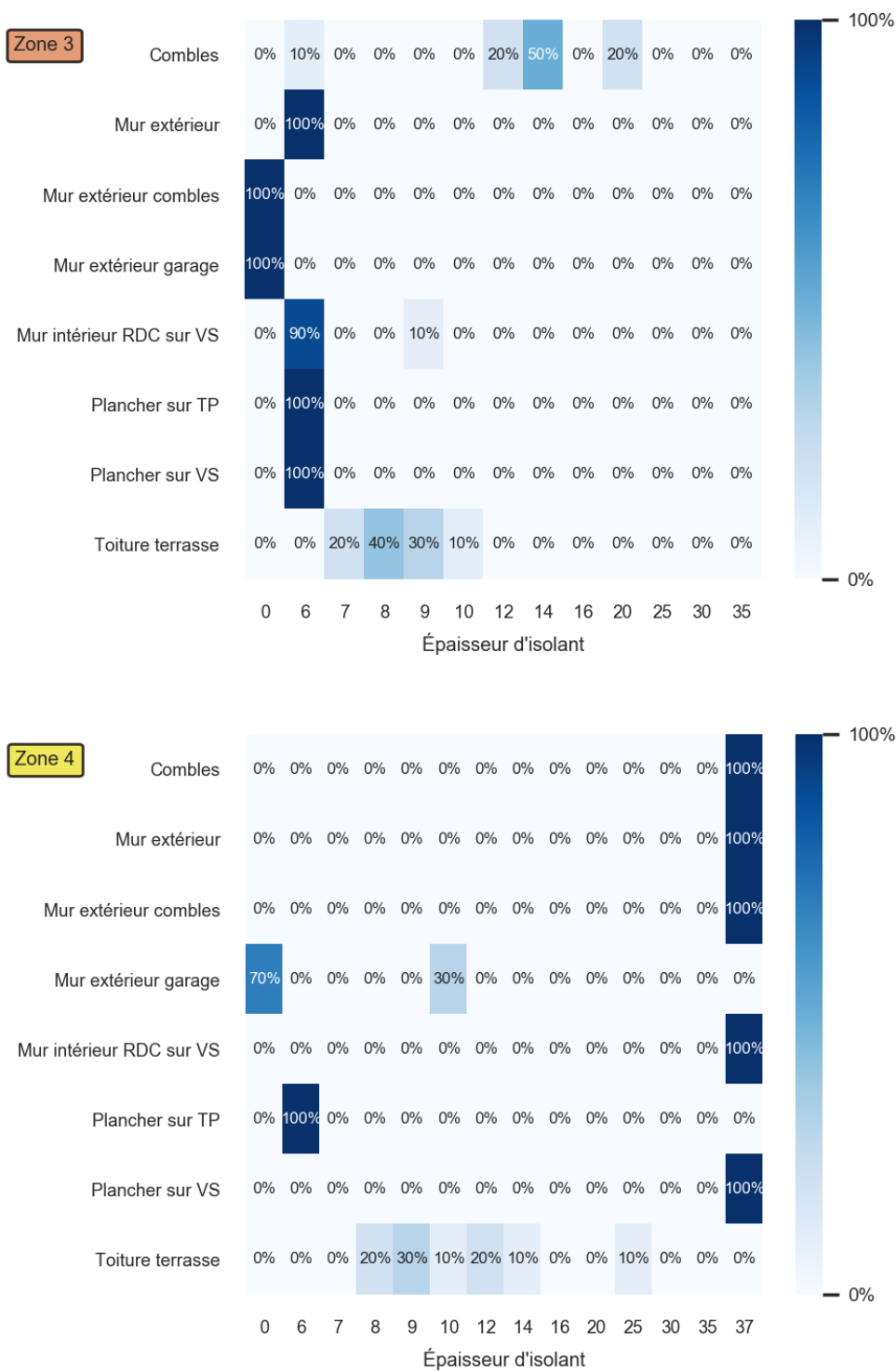
Figure 3.19 - Carte de chaleur des épaisseurs d'isolant dans les solutions (zones 3-4)
