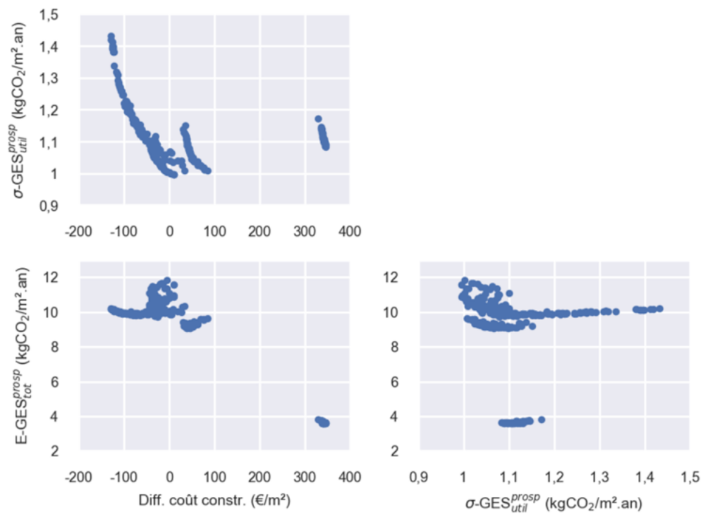
Figure 5.7 – Front de Pareto du POMR GES représenté par paire de fonctions objectif
