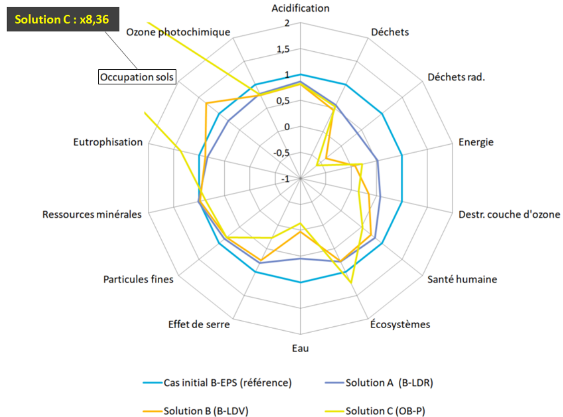
Figure 3.25 – Graphe radar des impacts environnementaux des solutions optimales A, B et C, et comparaison avec le cas initial
