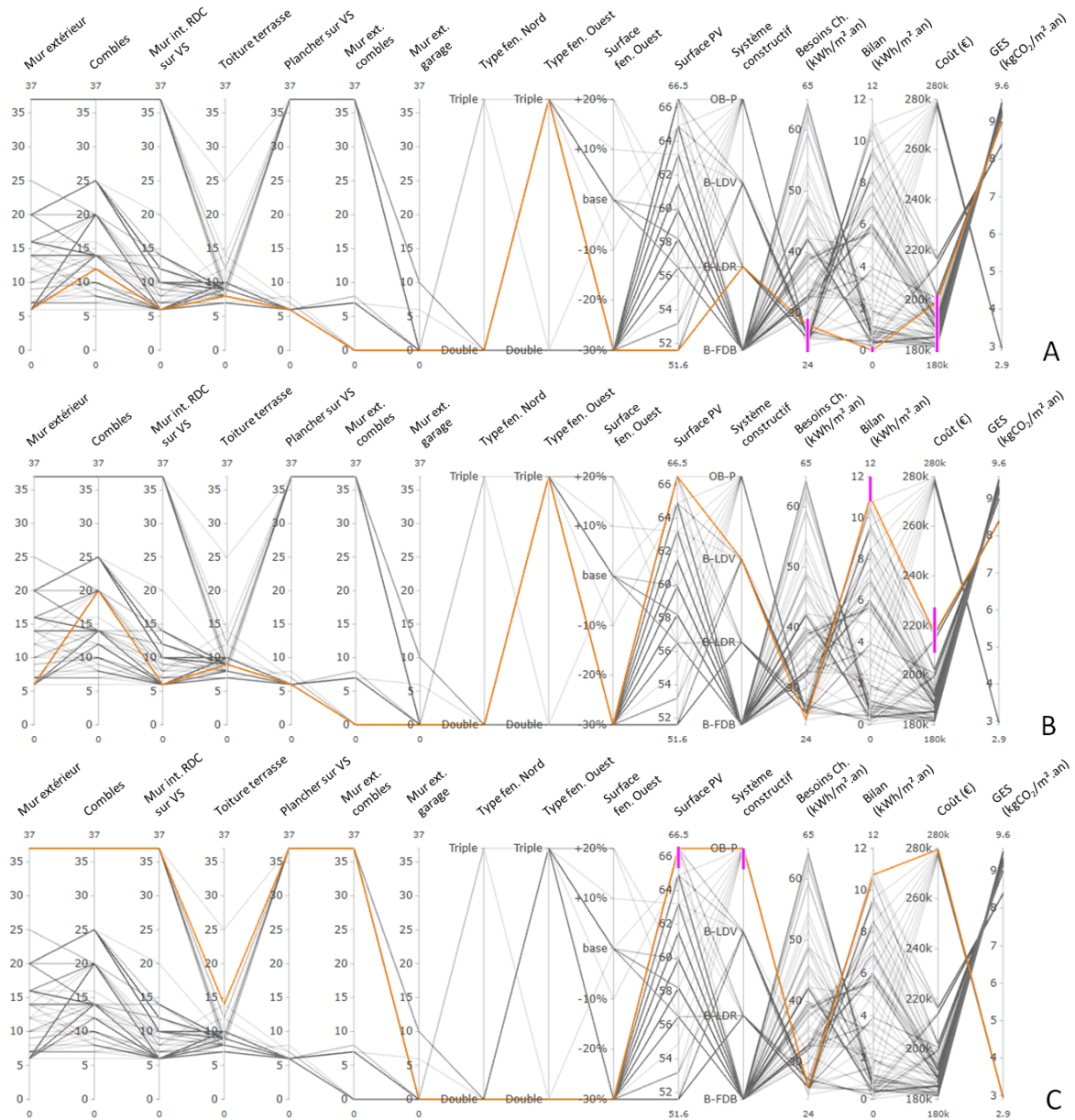
Figure 3.24 – Coordonnées parallèles et choix de trois décideurs A, B et C dans une prise de décision a posteriori de l'optimisation multicritère
