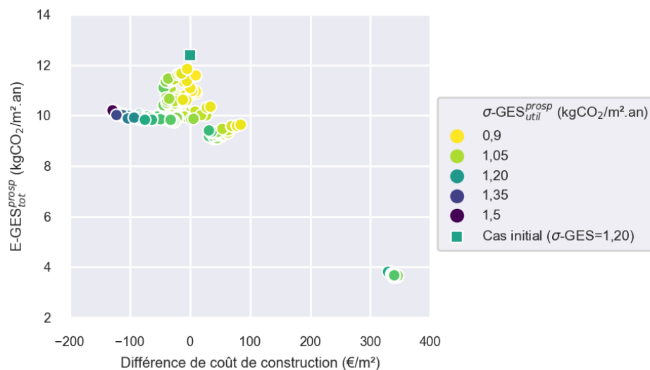
Figure 5.8 – Front de Pareto du POMR GES avec un gradient de couleur sur la valeur d'écart-type de l'émission de GES durant l'utilisation
