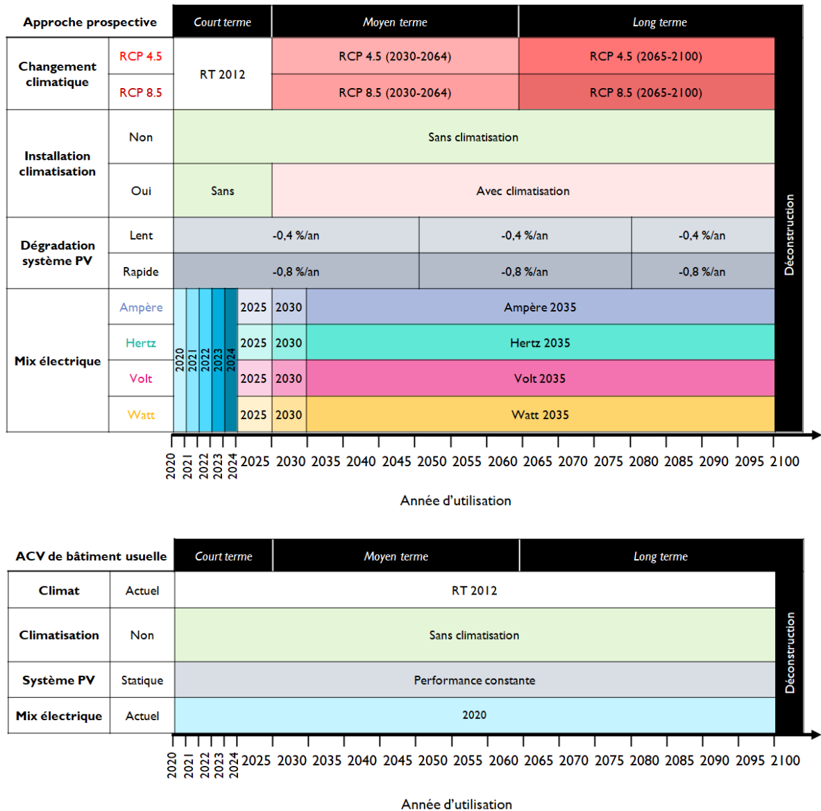
Figure 4.27 – Illustration des scénarios de cycle de vie de l'approche prospective et comparaison avec l'approche usuelle de l'ACV de bâtiment
