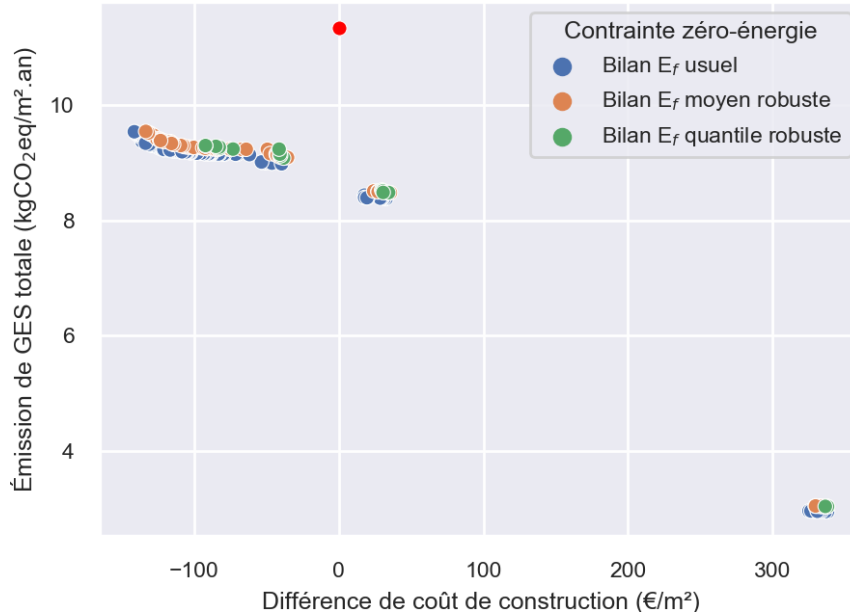
Figure 5.1 – Fronts de Pareto de POM/POMR avec différentes contraintes zéro-énergie
