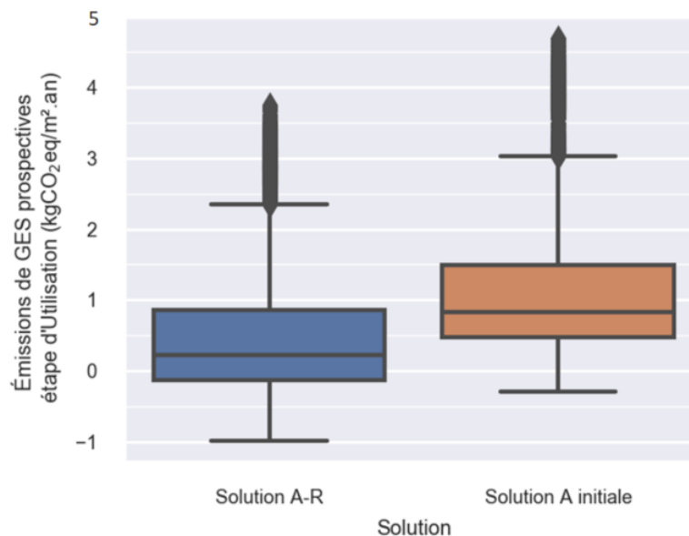
Figure 5.14 – Boîtes à moustaches des émissions de GES des années prospectives de l'étape d'utilisation pour les solutions A-R et A initiale
