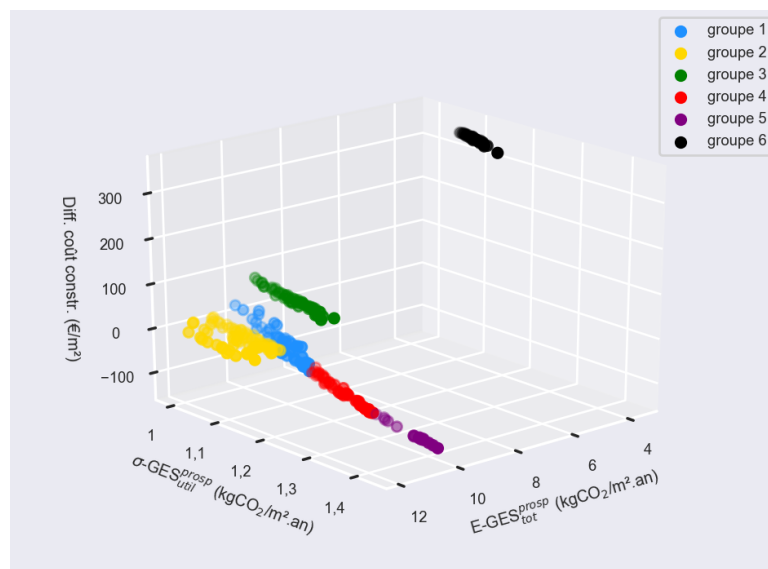
Figure 5.9 – Front de Pareto 3D du POMR GES avec visualisation des groupes
