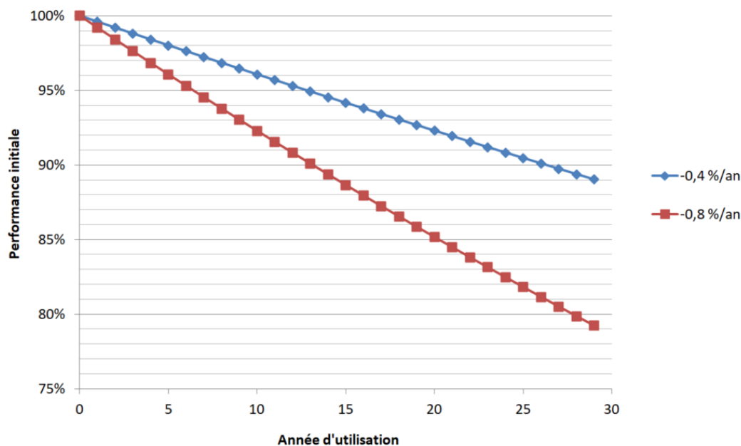
Figure 4.26 – Évolution de la performance d'un système solaire PV par rapport à sa performance initiale avec deux taux de dégradation annuelle
