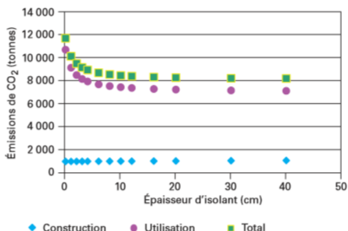
Figure 1.19 – Non-linéarité entre l'émission de CO 2 du cycle de vie d'un bâtiment et l'épaisseur d'isolant. Source : Peuportier (2014)
