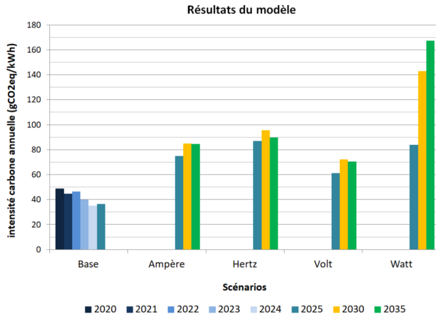
Figure 4.19 - Moyenne annuelle de l'émission de GES des scénarios d'après les résultats du modèle du système électrique
