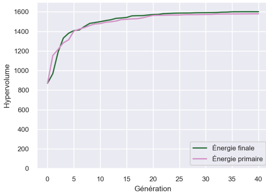
Figure 3.34 – Évolution de l'hypervolume des fronts des POM basés sur la contrainte du bilan d'énergie finale et du bilan d'énergie primaire
