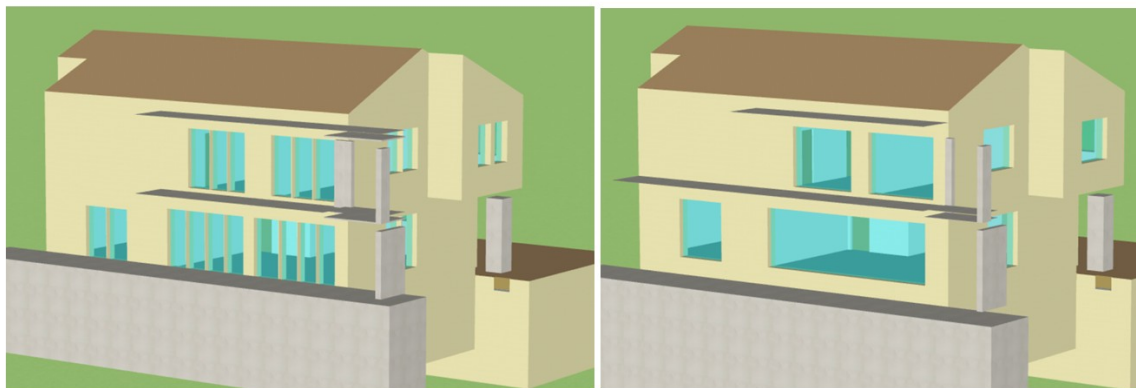
Figure 2.19 - Simplification des vitrages. Gauche : 17 fenêtres, droite : 9 fenêtres
