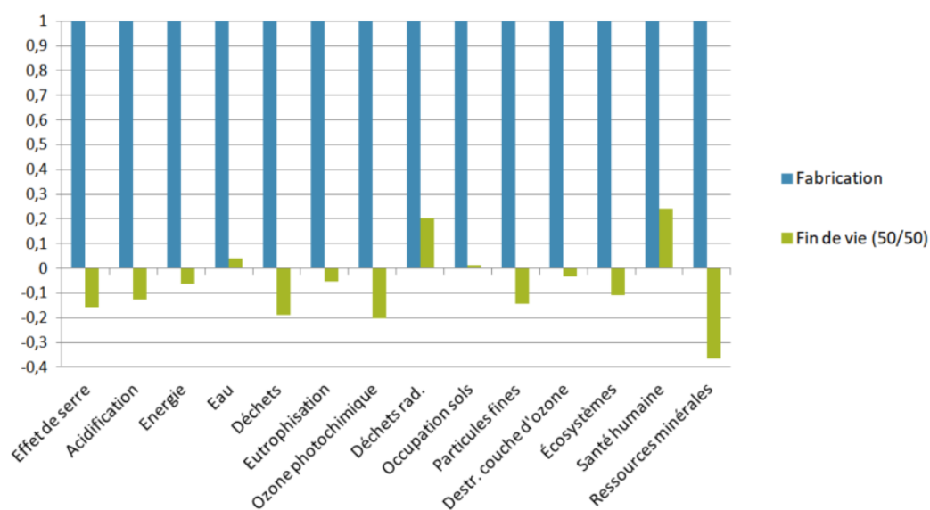
Figure 2.14 – Comparaison des impacts de fabrication et de fin de vie d’un ballon de stockage. Unité fonctionnelle de 1 L
