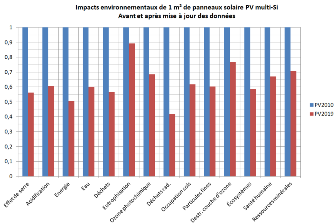
Figure 2.8 – Comparaison des impacts du système PV avant et après mise à jour
