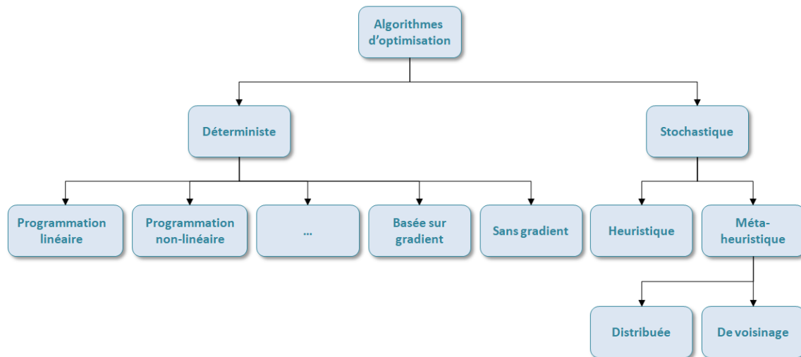
Figure 1.18 – Classification des algorithmes d'optimisation extrait de Xin-She Yang (2010)
