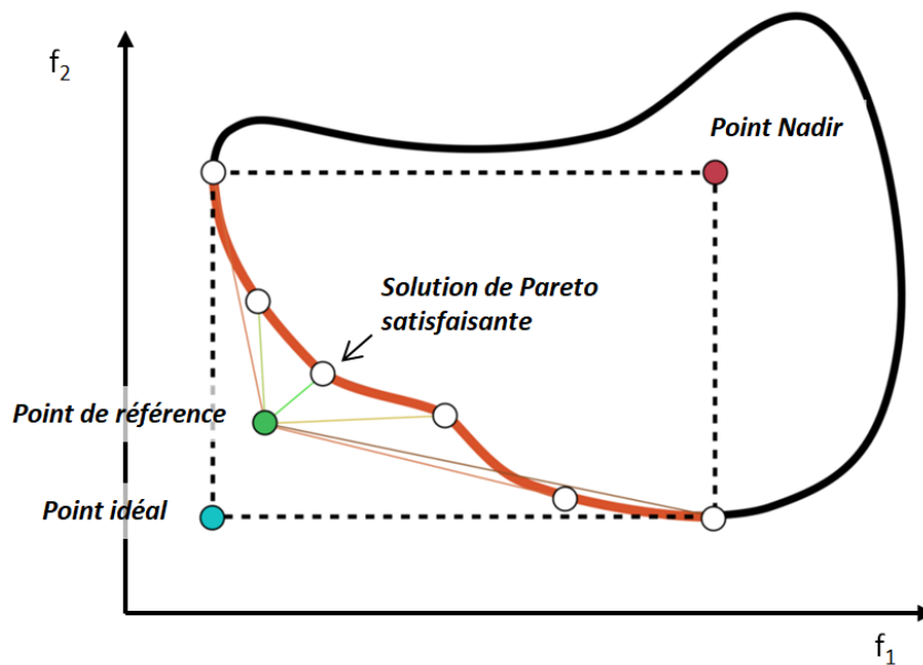
Figure 1.17 – Illustration des points idéal, de référence et Nadir, d'une solution de Pareto satisfaisante et de la frontière de Pareto
