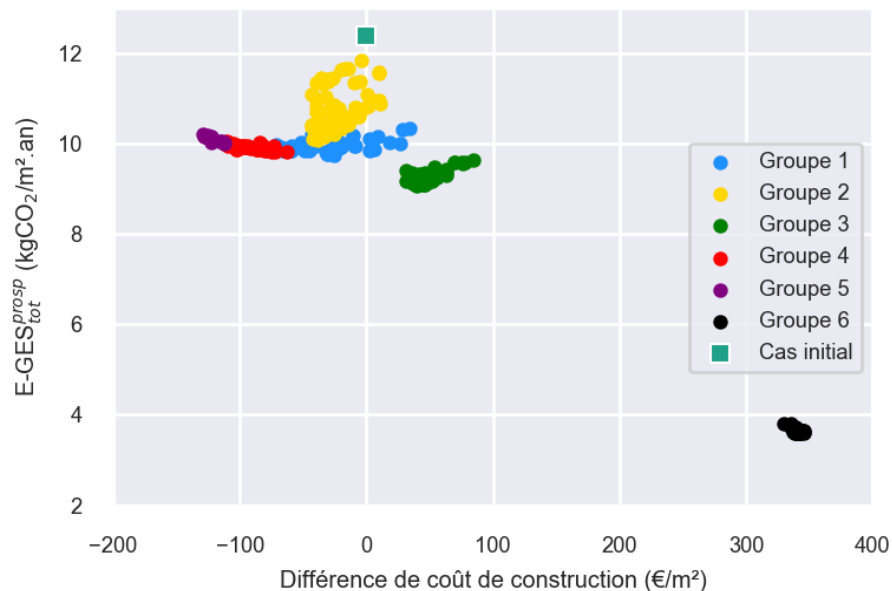
Figure 5.10 – Représentation en 2D du front de Pareto du POMR GES selon la moyenne des
