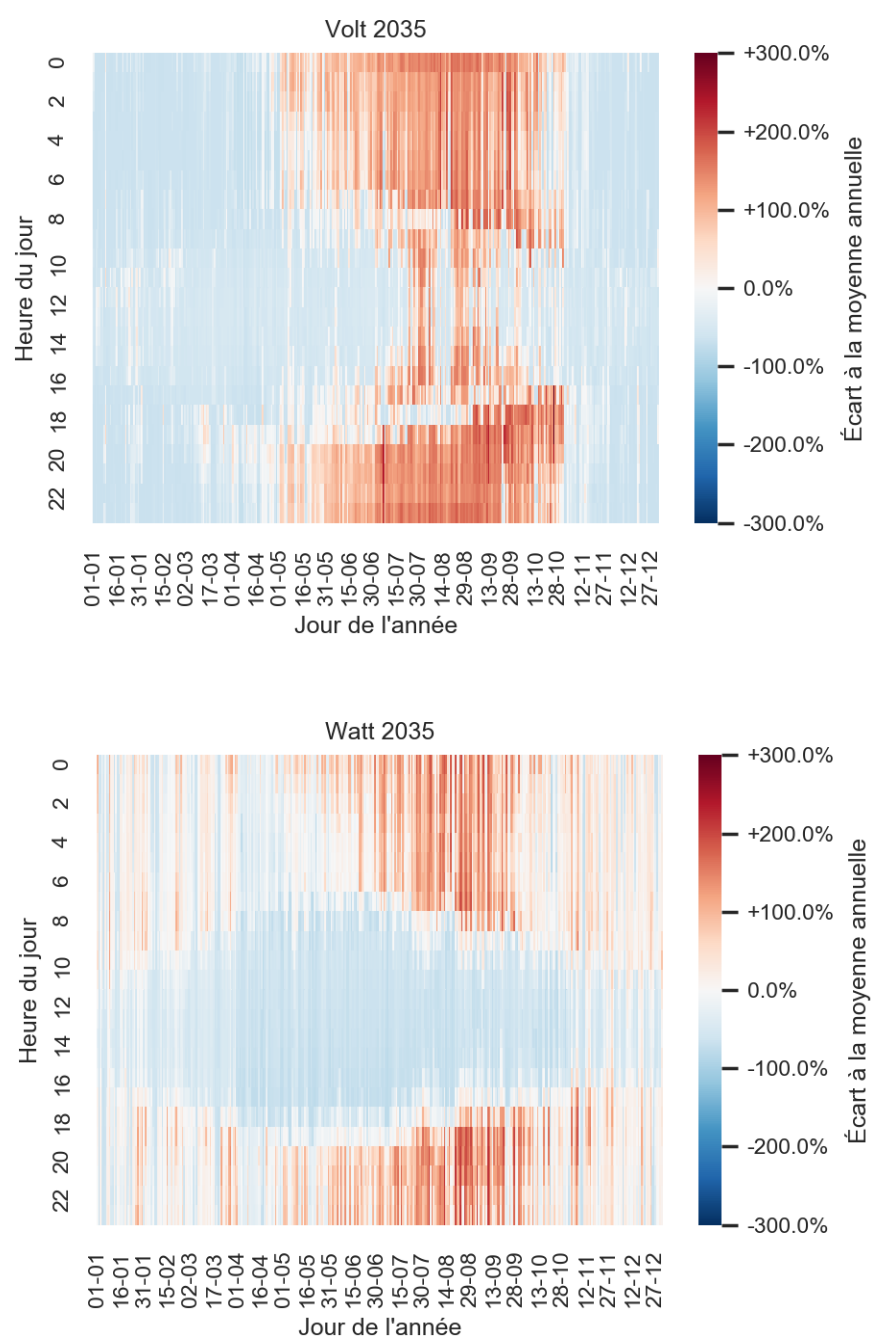
Figure 4.25 – Carte de chaleur de l'écart à la moyenne annuelle de l'intensité carbone d'un kWh d'électricité pour l'année 2035 et les scénarios Volt et Watt
