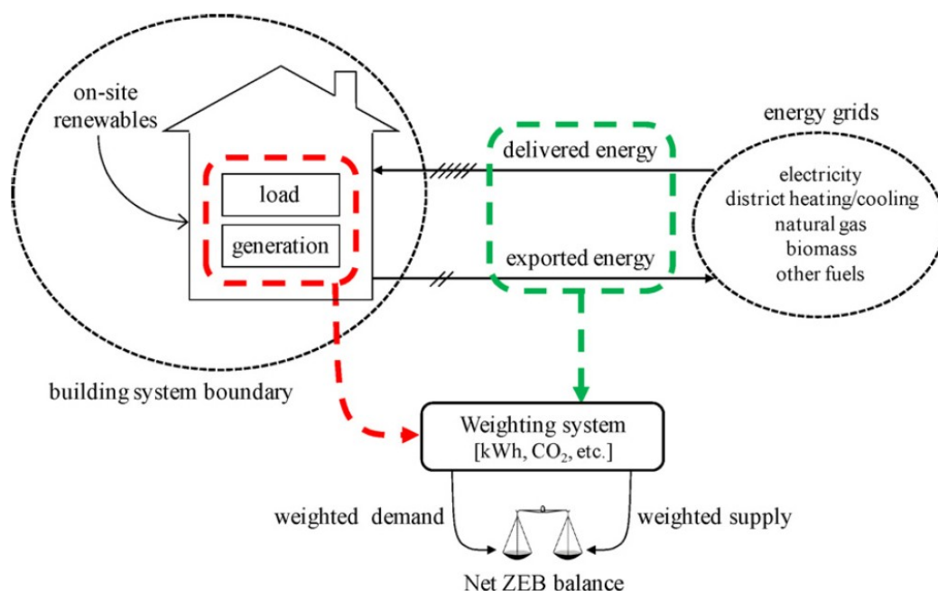
Figure 1.3 - Relations entre la frontière physique du bâtiment et les réseaux d'énergie. Illustration des types de bilan (Sartori et al. 2012)
