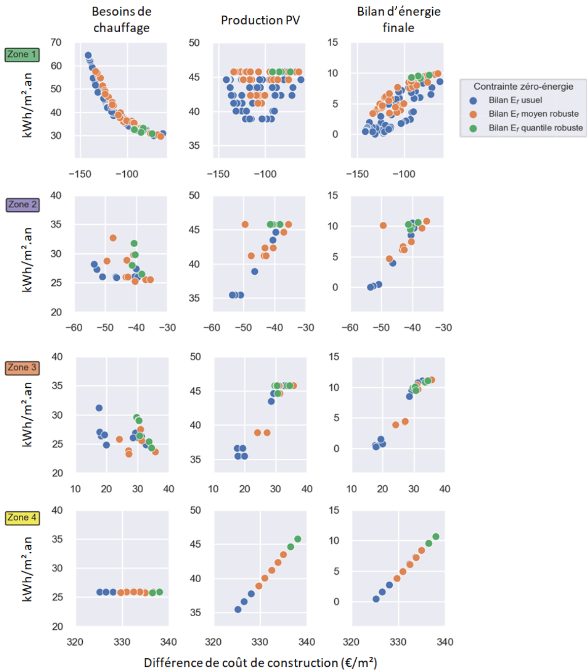
Figure 5.3 – Besoins de chauffage, production d’électricité PV et bilan d’énergie finale de la 1ère année d’utilisation des POM/POMR avec différentes contraintes zéro-énergie. Zone 1 : béton et fibre de bois, zone 2 : béton et laine de roche, zone 3 : béton et laine de verre, zone 4 : ossature bois et paille
