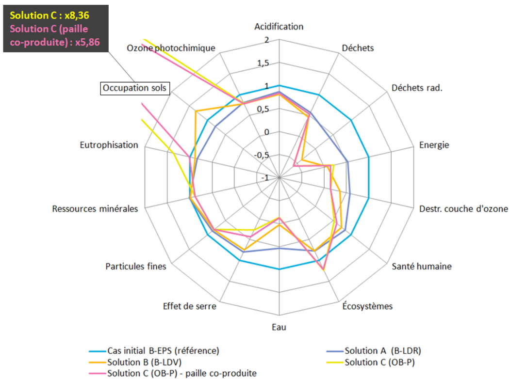
Figure 3.27 – Graphe radar comparant la solution C (OB-P) incluant de la paille co-produite avec les solutions initiales des décideurs
