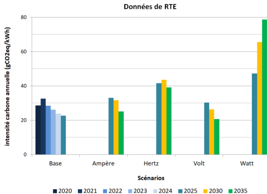
Figure 4.18 – Moyenne annuelle de l’émission de GES des scénarios d’après les BP 2017 et 2019 de RTE
