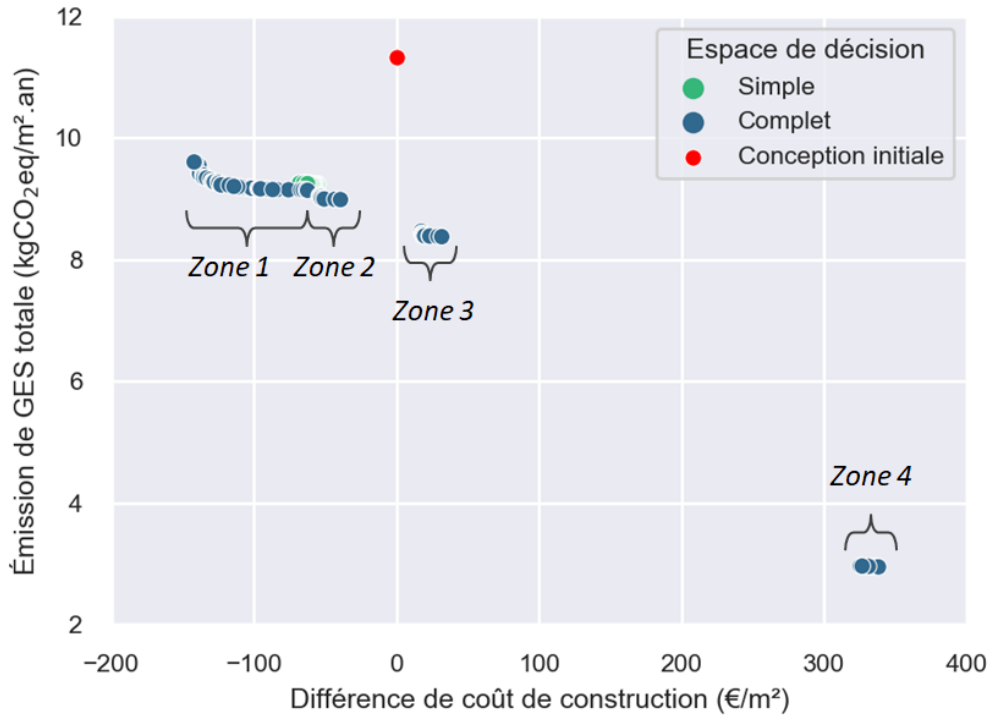
Figure 3.16 – Comparaison des fronts du POM Simple et du POM Complet
