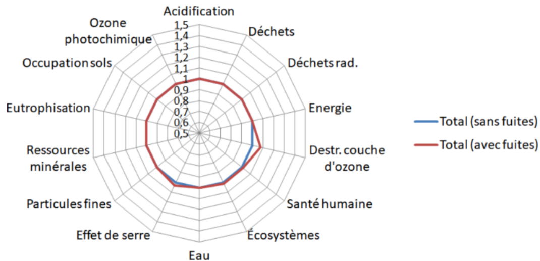
Figure 2.24 – Graphe radar des impacts totaux avec et sans prise en compte des fuites de fluide frigorigène
