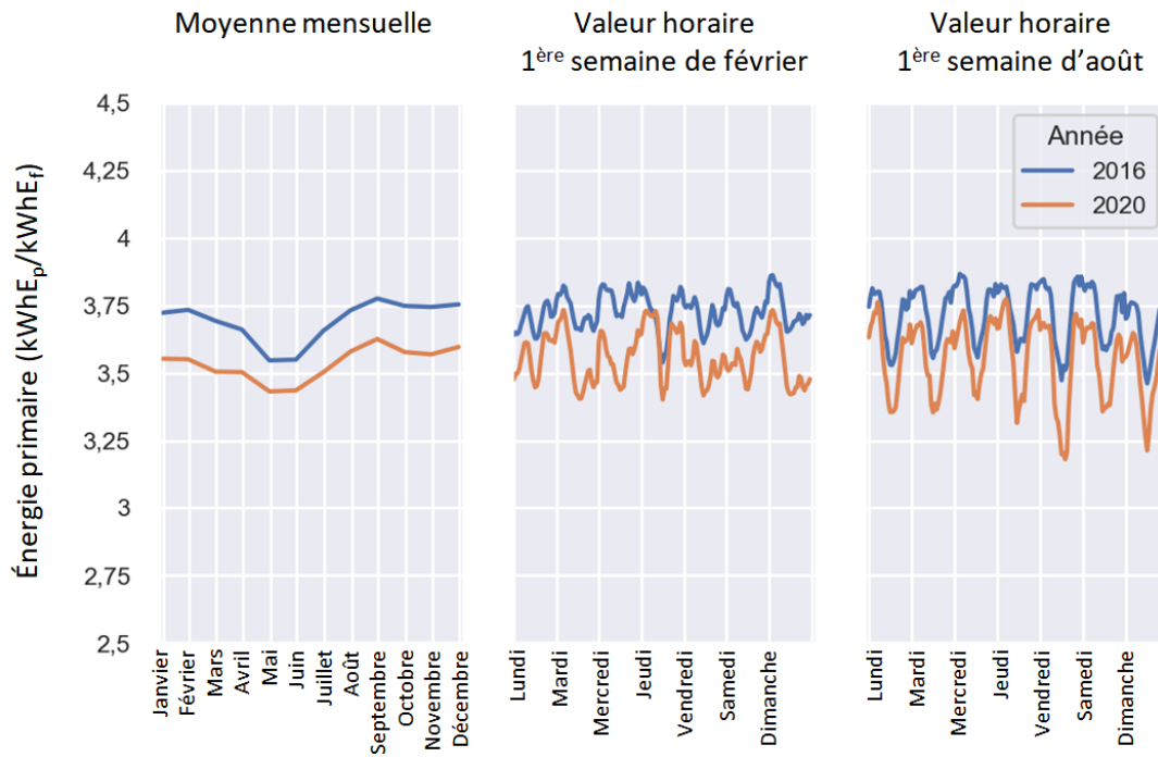
Figure 3.32 – Variabilité mensuelle et journalière du coefficient d'énergie primaire
