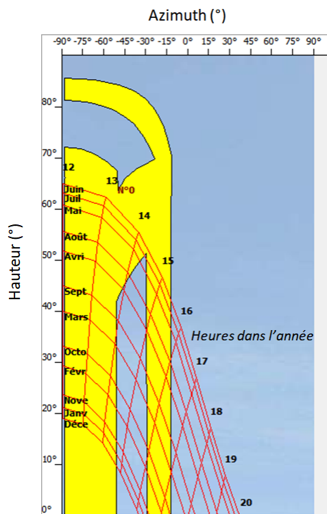
Figure 3.22 – Masque visible depuis la fenêtre Ouest durant l’année
