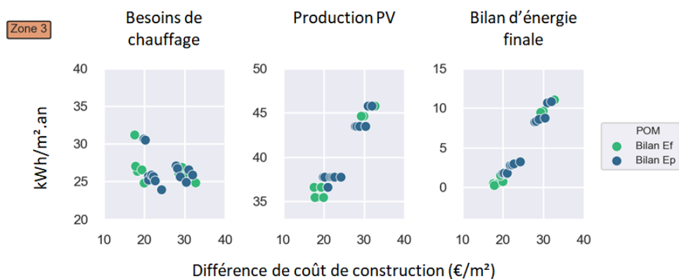
Figure 3.37 – Comparaisons de la zone 3 des POM avec bilan Ef et avec bilan Ep
