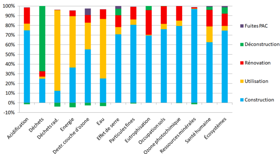
Figure 2.25 - Histogrammes des impacts par étapes du cycle de vie
