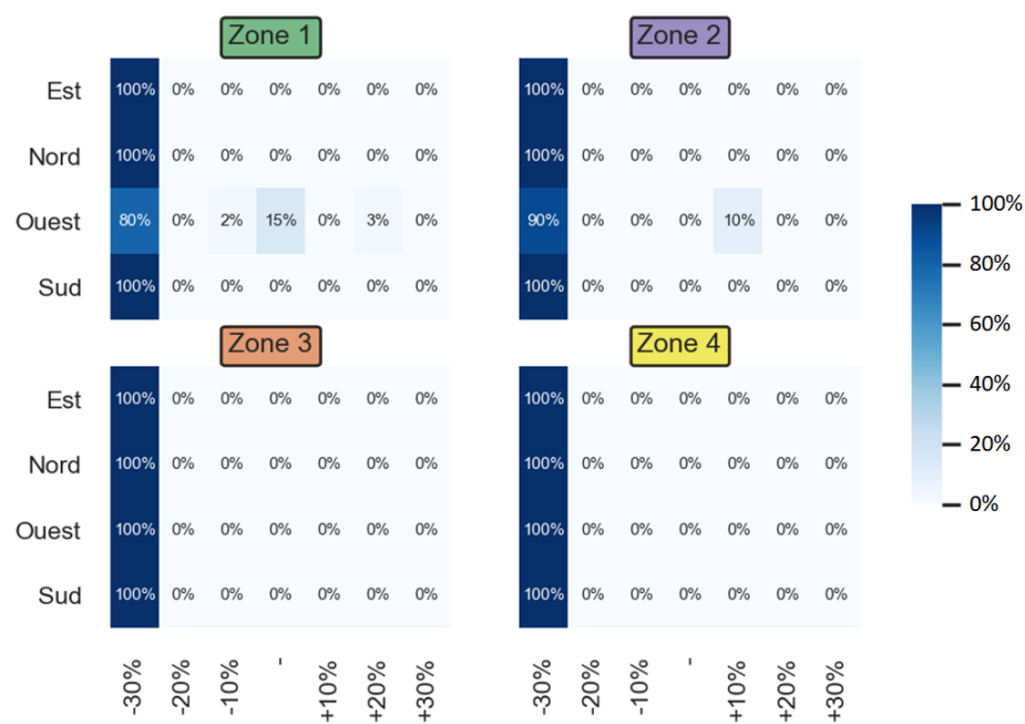
Figure 3.21 – Carte de chaleur du changement de surface vitrée par orientation dans les solutions des zones d’optimum local
