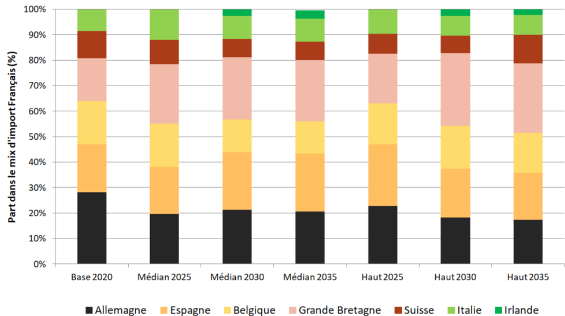
Figure 4.16 – Composition des imports d’électricité à partir de scénarios d’interconnexion
