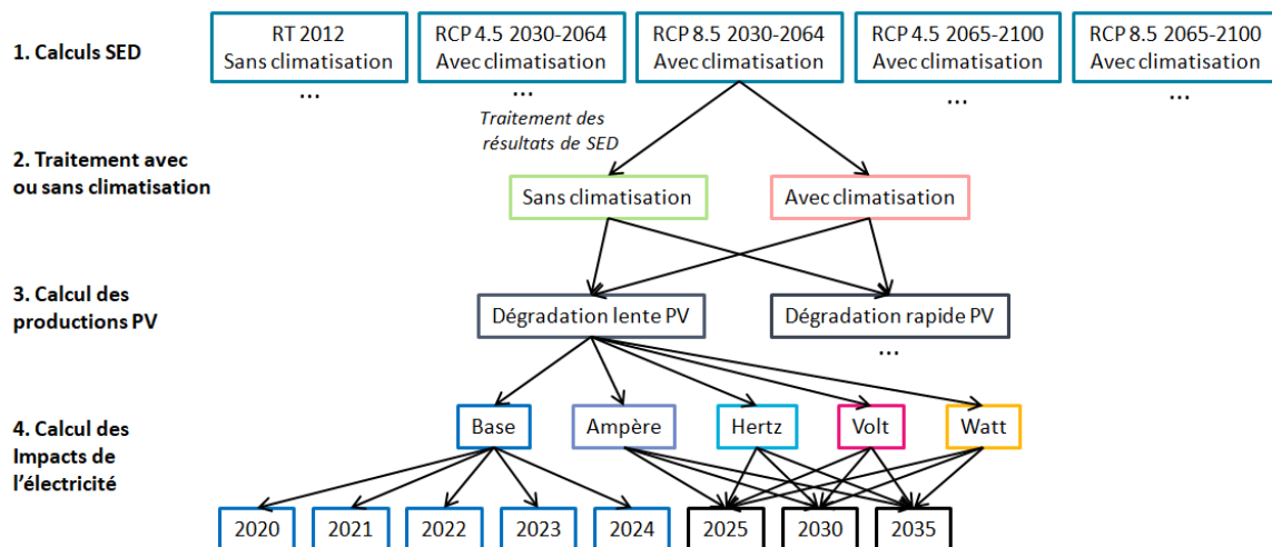
Figure 4.28 – Étapes et répartitions des calculs des années individuelles prospectives en optimisation multicritère robuste
