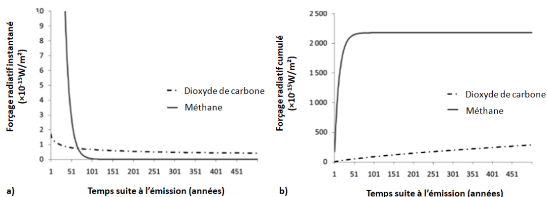
Figure 1.11 – Forçage radiatif instantané (a) et cumulé (b) de l'émission d'une masse unitaire de dioxyde de carbone et de méthane (Levasseur et al., 2010)
