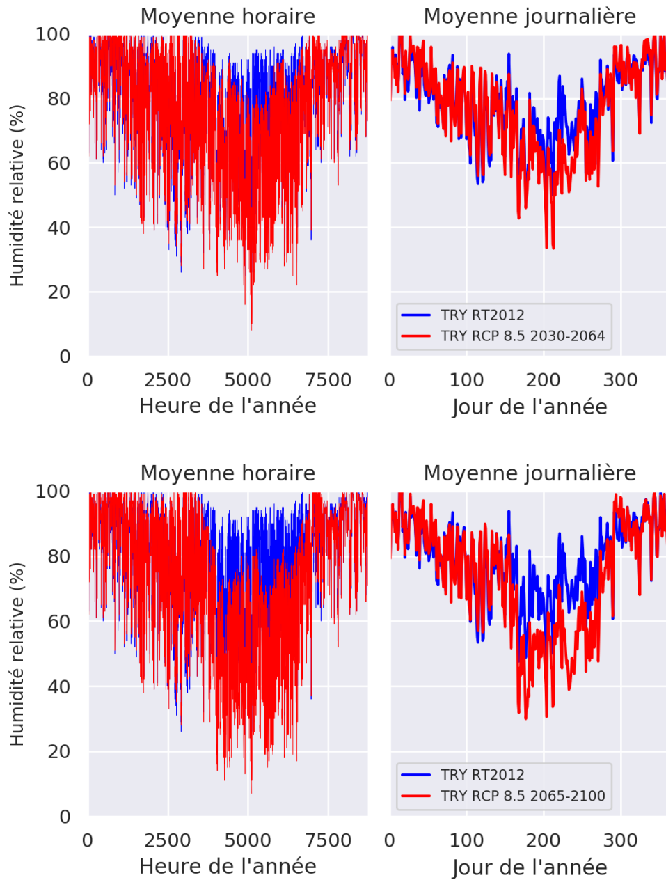
Figure 4.14 – Humidité relative dans les données issues du morphing appliqué à la station de Trappes (H1a), scénario RCP 8.5
