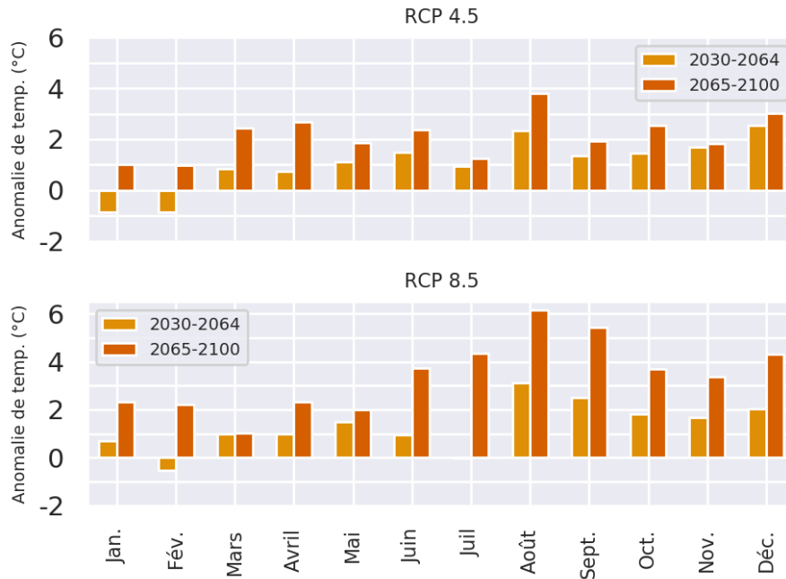
Figure 4.9 – Anomalies mensuelles moyennes de la température extérieure des données issues du morphing par rapport aux données climatiques de la RT2012 pour la station météorologique de Trappes
