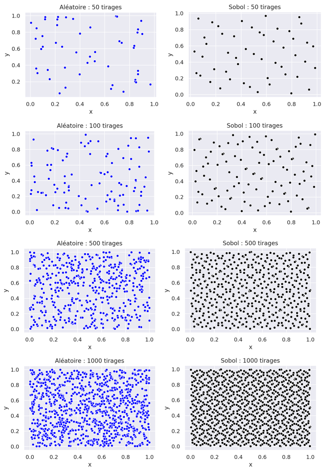
Figure 2.15 – Comparaison de tirages aléatoires et de séquences de Sobol
