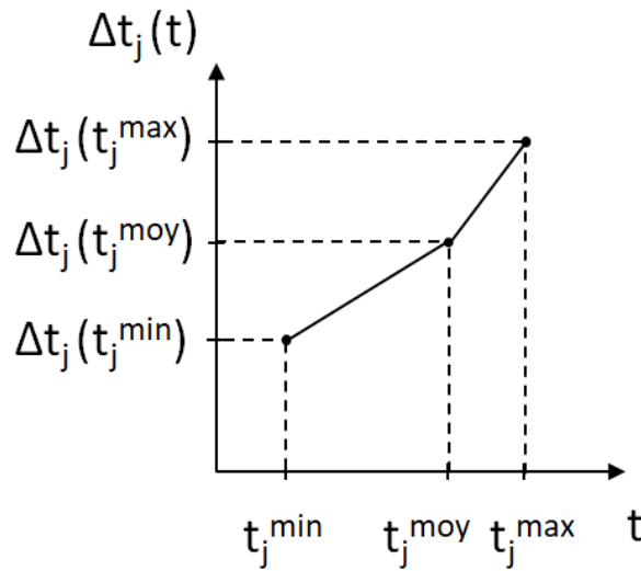
Figure 4.6 – Illustration du décalage absolu en fonction des températures d'un jour j donné
