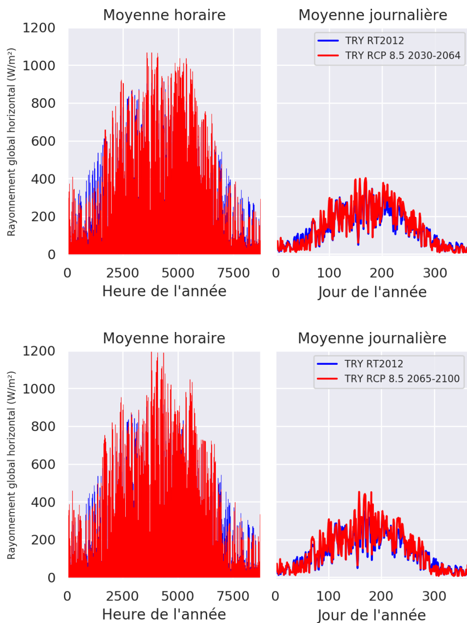
Figure 4.12 – Rayonnement global horizontal des données issues du morphing appliqué à la station de Trappes (H1a), scénario RCP 8.5
