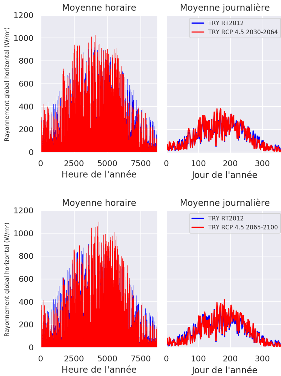
Figure 4.11 – Rayonnement global horizontal des données issues du morphing appliqué à la station de Trappes (H1a), scénario RCP 4.5
