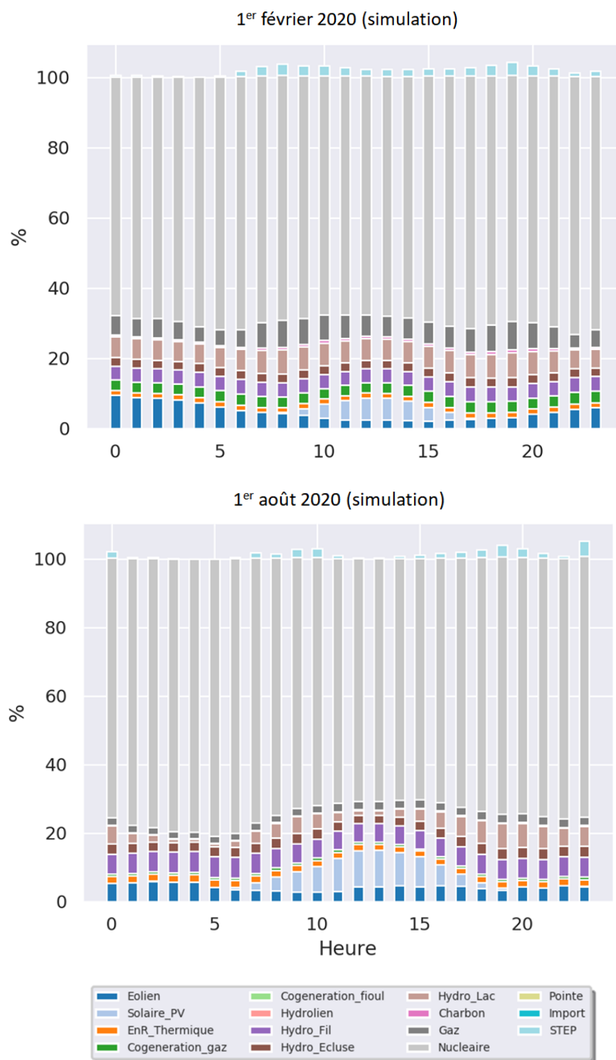
Figure 3.33 – Composition du mix électrique infra-journalier le 1 er février et le 1 er août de l'année 2020 simulée
