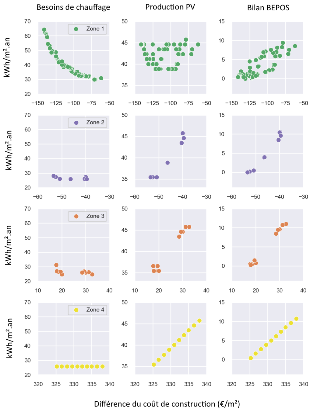
Figure 3.17 – Évolutions des besoins de chauffage, de la production PV et du bilan zéro-énergie/BEPOS en fonction du coût de construction des solutions des optimums locaux
