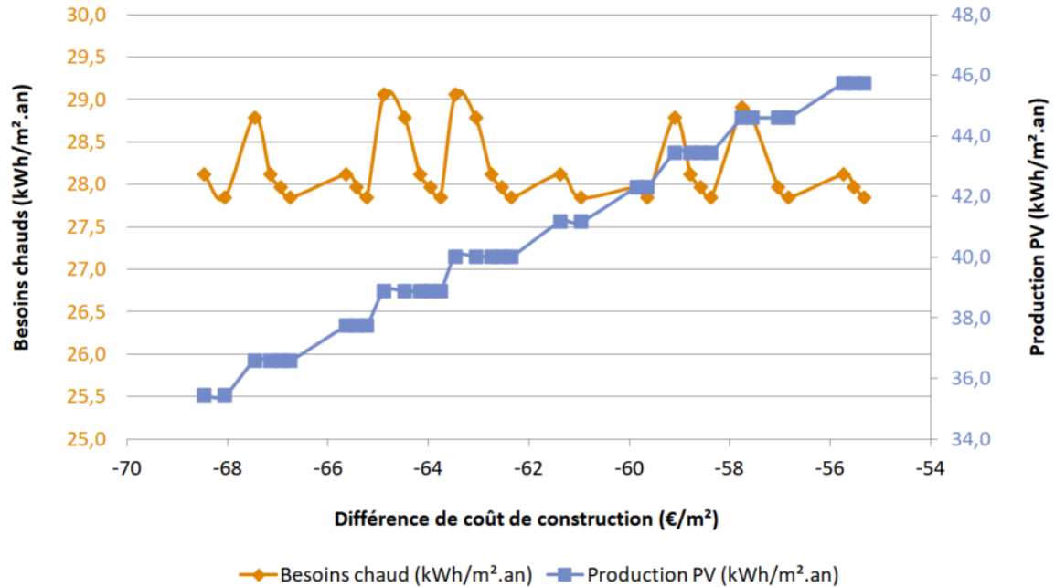
Figure 3.6 – Évolution des besoins de chauffage et de la production PV avec l'investissement dans les solutions du front du POM Simple
