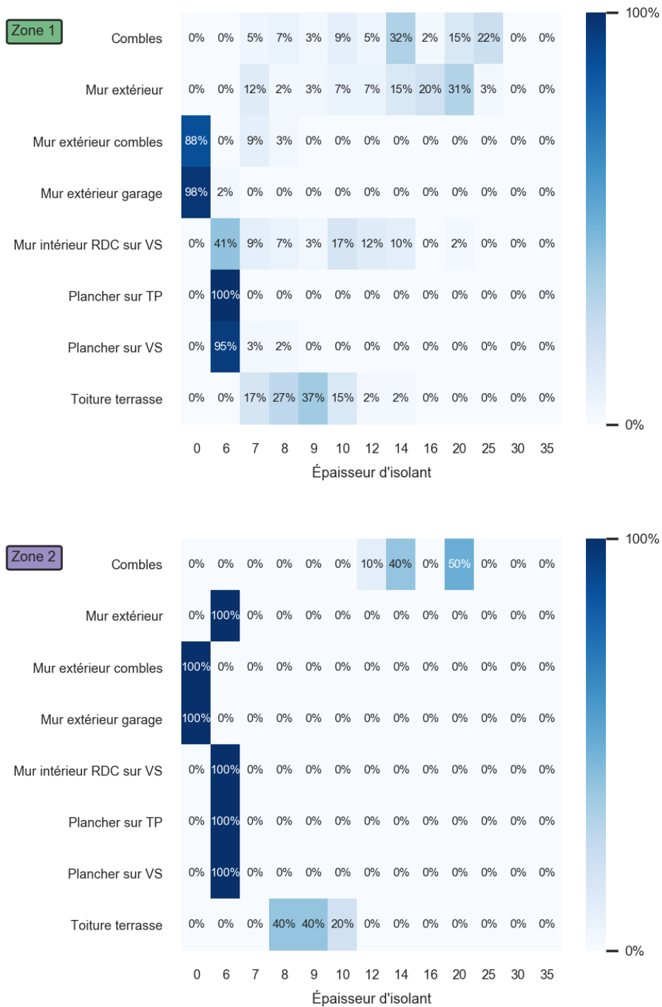
Figure 3.18 – Carte de chaleur des épaisseurs d'isolant dans les solutions (zones 1-2)
