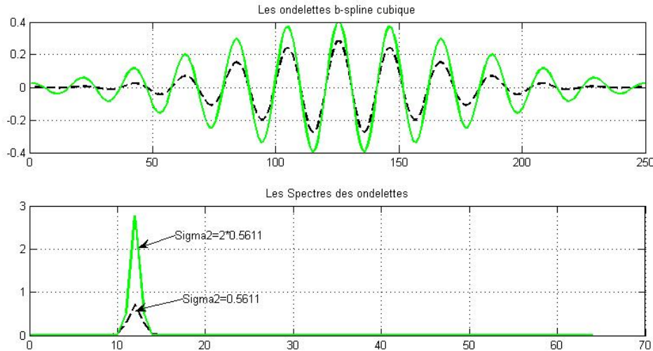
Figure 3-7 : L'influence du paramètre \sigma^2 de l'ondelette mère.
