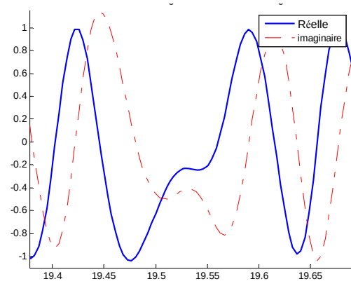
Figure 3-38 : Signal analytique du signal normalisé
