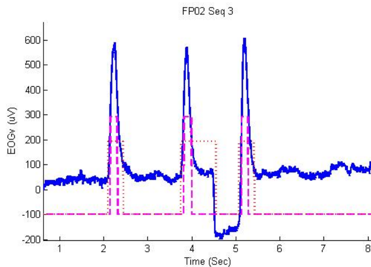
Figure 2-8: Proximité entre un mouvement d'oeil et un clignements d'œil
