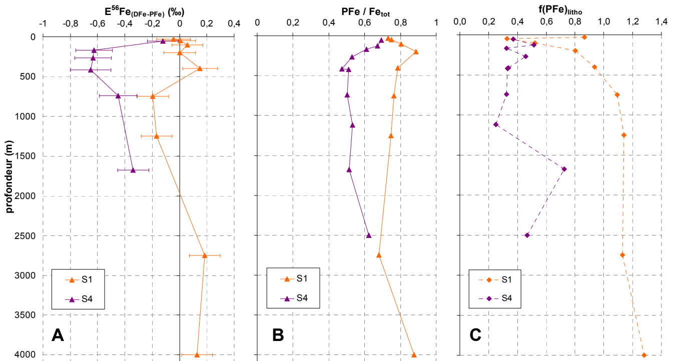
Figure 4.11 : A) profils de E^{56}\text{Fe}_{(\text{DFe-PFe})} (où E^{56}\text{Fe}_{(\text{DFe-PFe})} = \delta^{56}\text{DFe} - \delta^{56}\text{PFe} ). B) profils du rapport de concentrations \text{PFe}/\text{Fe}_{\text{tot}} (où \text{Fe}_{\text{tot}} = \text{DFe} + \text{PFe} ). C) profils de la fraction lithogénique des particules, notée f(\text{PFe})_{\text{litho}} , déduite du rapport [\text{PAI}] / [\text{PFe}] = 3.03 de la moyenne crustale (Taylor 1964 ; Chester, 1990).
