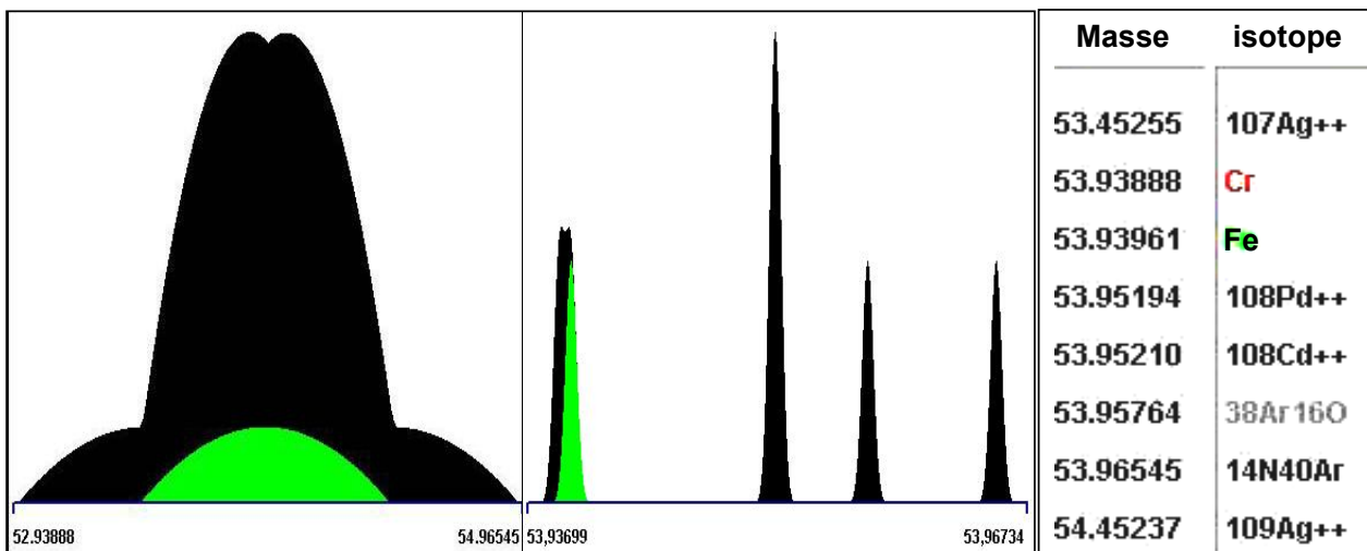
Figure 2.4 : Graphique du signal mesuré au voisinage de la masse 54 en fonction de la masse avec une basse résolution (à gauche) et une haute résolution (au milieu). La contribution du 54 Fe est représentée en vert et celle de ces interférences (listées à droite) en noir.
