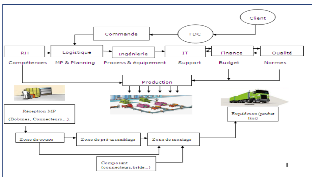
Figure 7: processus de fabrication des faisceaux
