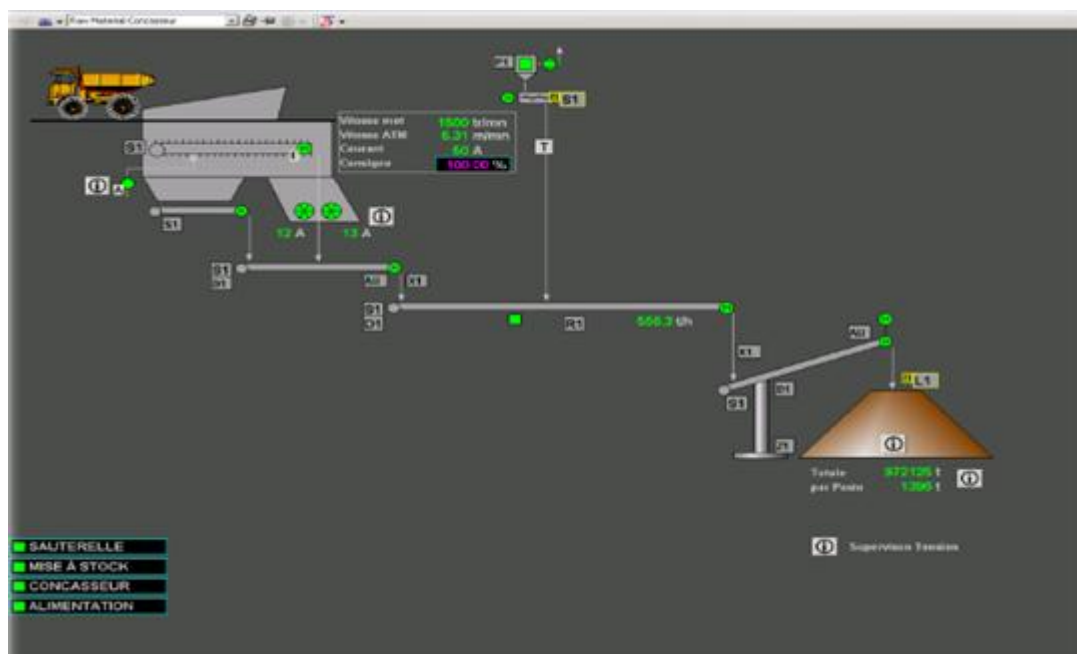
Figure 4: Flow sheet du concasseur
