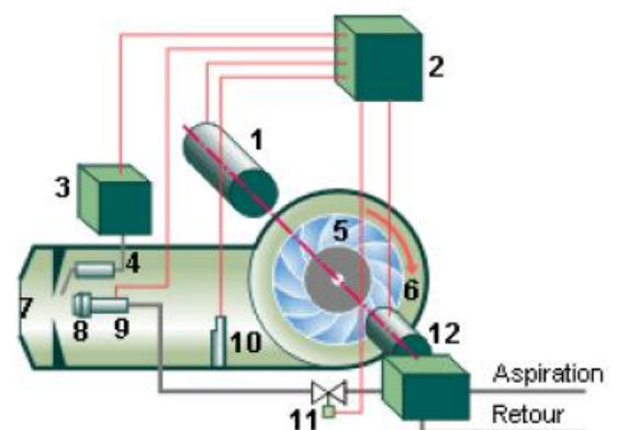
Figure 13 : Bruleur Fuel
