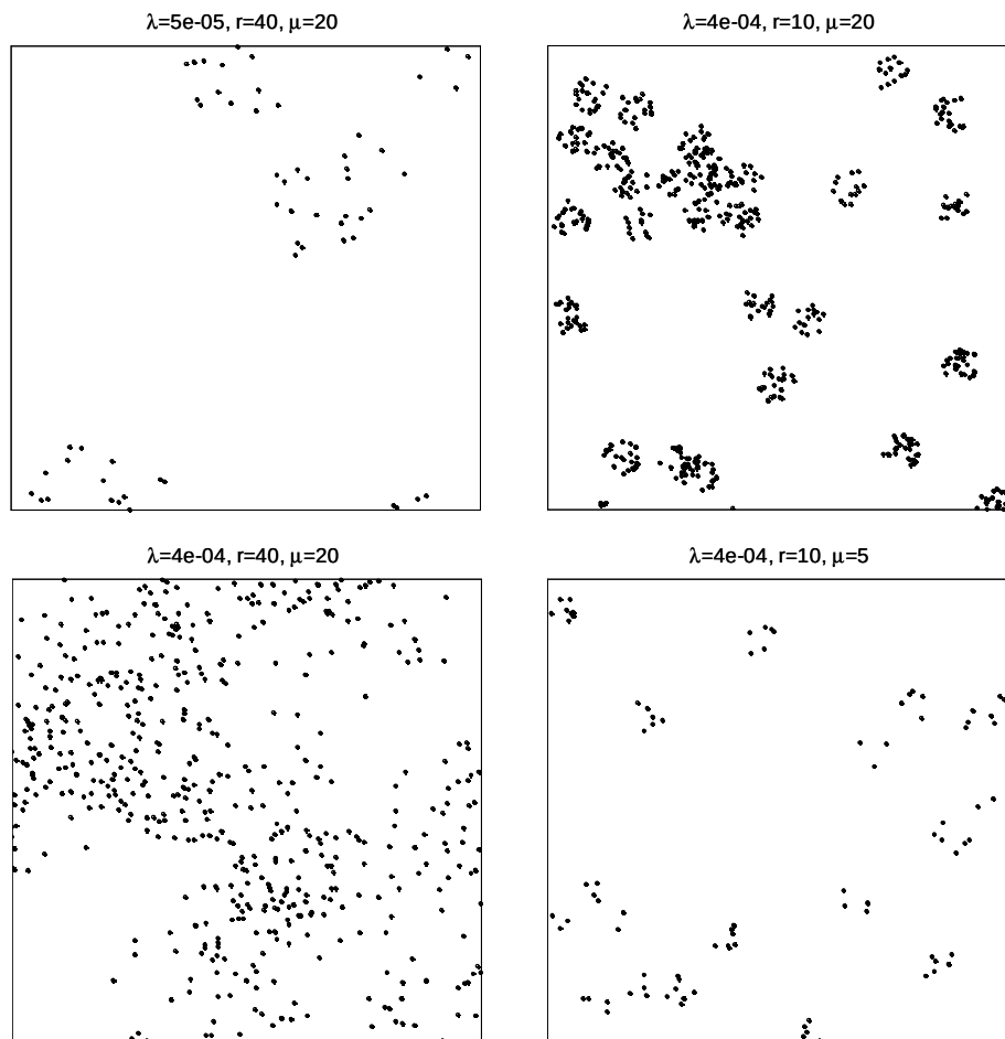
Figure 2-5 : Exemple de quatre semis de points simulés par un processus de Matérn.
