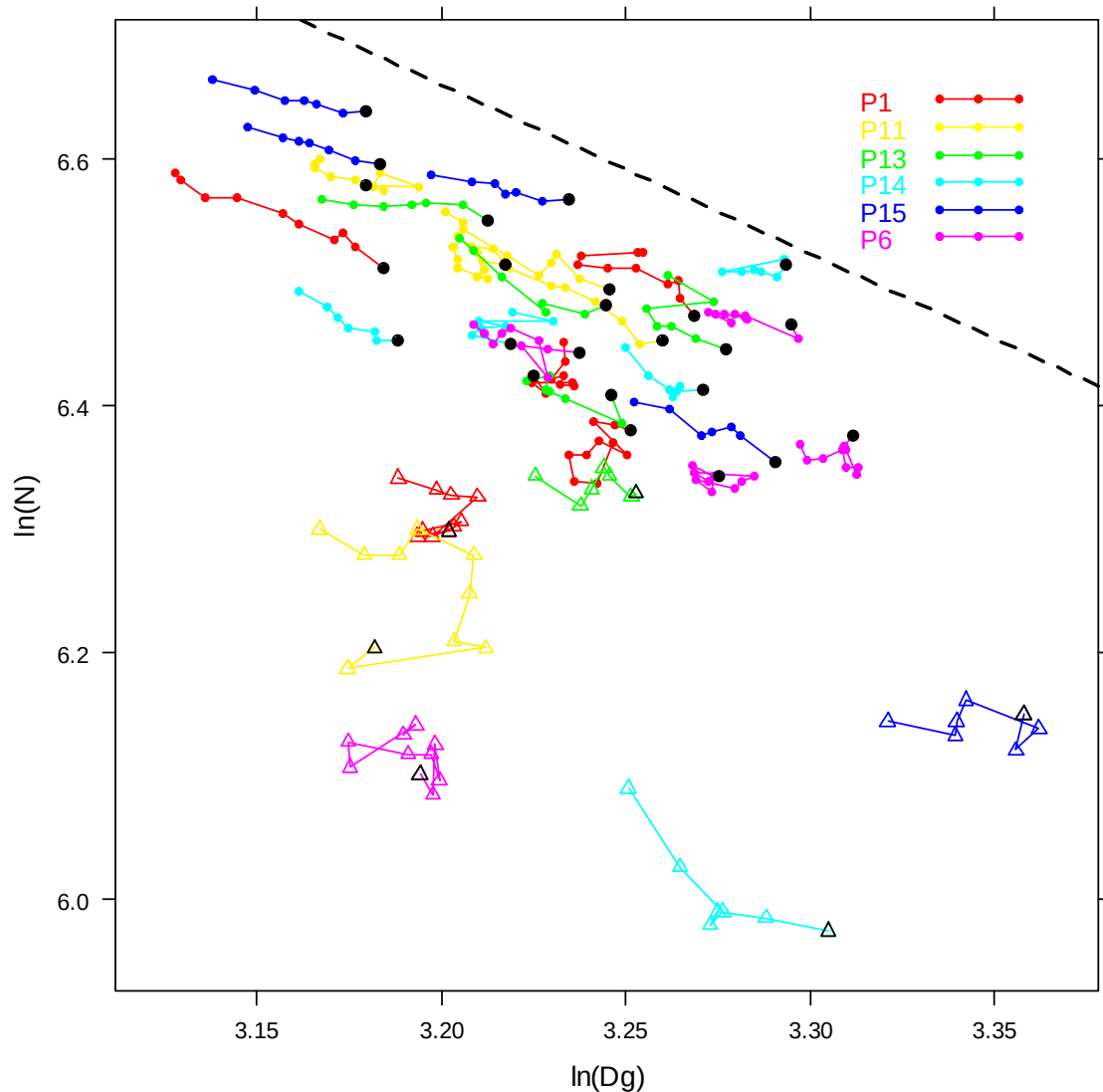
Figure 4-8 : Droite d'autoéclairecie ajustée sur les données des 6 parcelles témoin de Paracou. Chaque parcelle est découpée en 4 carrés hors bas-fond (points) et un bas-fond (triangle). Les symboles noirs identifient la dernière valeur du couple (d_g, N) , calculée en 2003. Les données de recrutement utilisées ont été lissées pour tenir compte des irrégularités (voir figure 1-7, p. 19).
