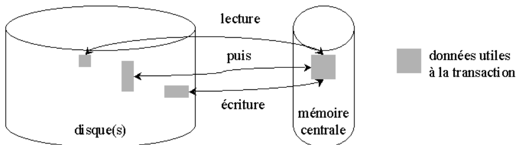
FIG. 7 – Traitement des données d'une transaction en mémoire
