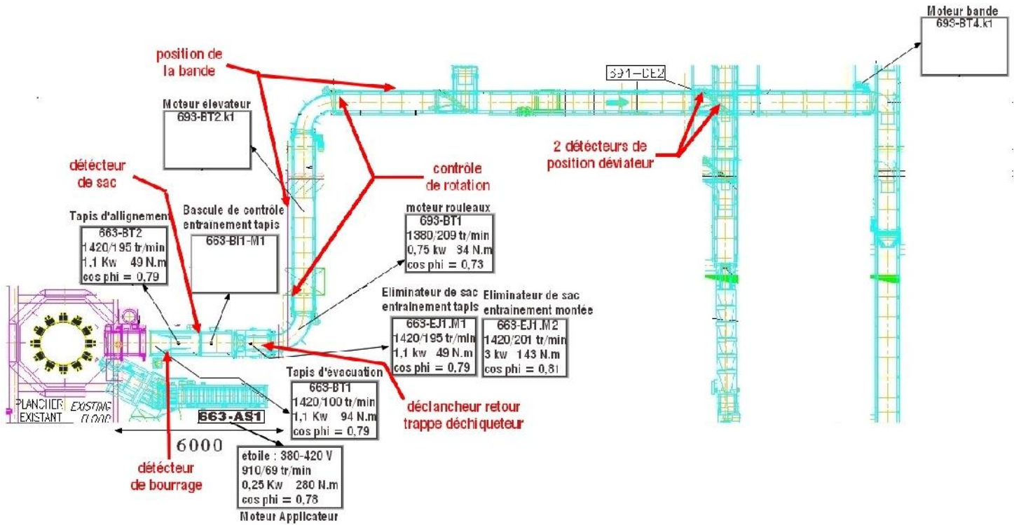
Figure 33: Schéma de la ligne Machine C – Caricamat A&B avec les détails des moteurs-réducteurs
