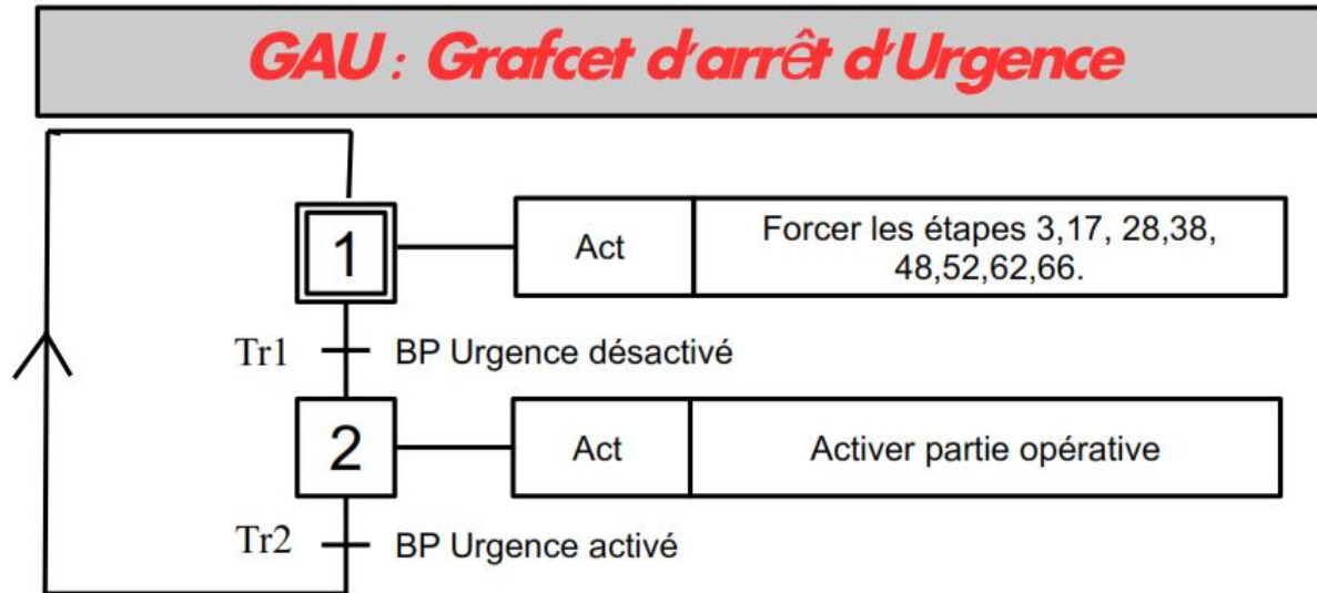
Figure 28: GAU – Grafcet d'arrêt d'urgence
