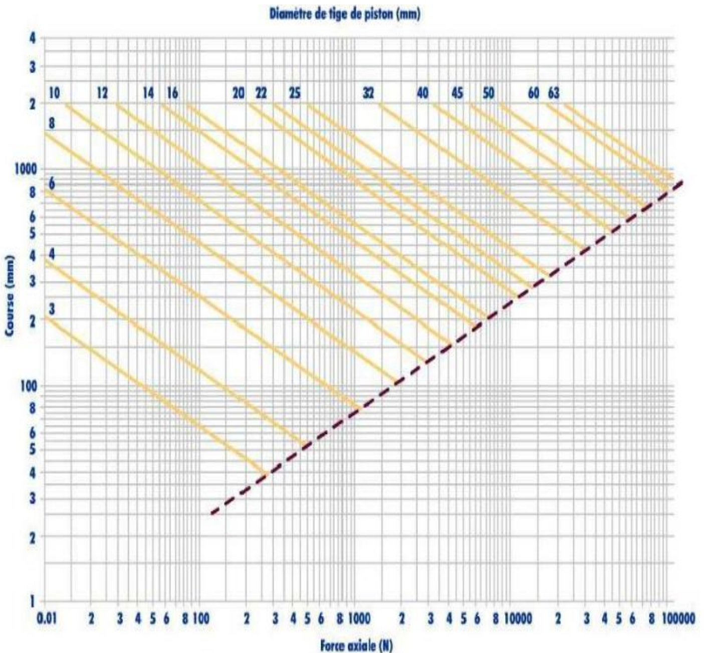
Figure 35: Diagramme du dimensionnement du vérin pneumatique à double effet
