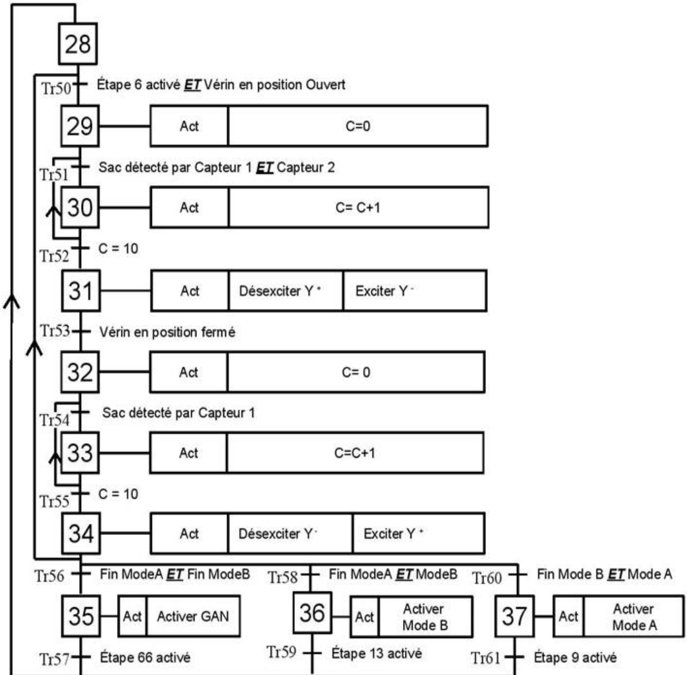
Figure 24: GEN1 – Grafcet d'expédition normale vers caricamat A et Caricamat B
