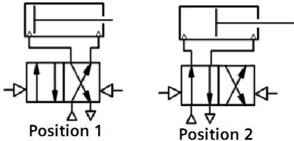
Figure 36 : Fonctionnement d'un vérin pneumatique à double effet avec un distributeur bistable 4/2
