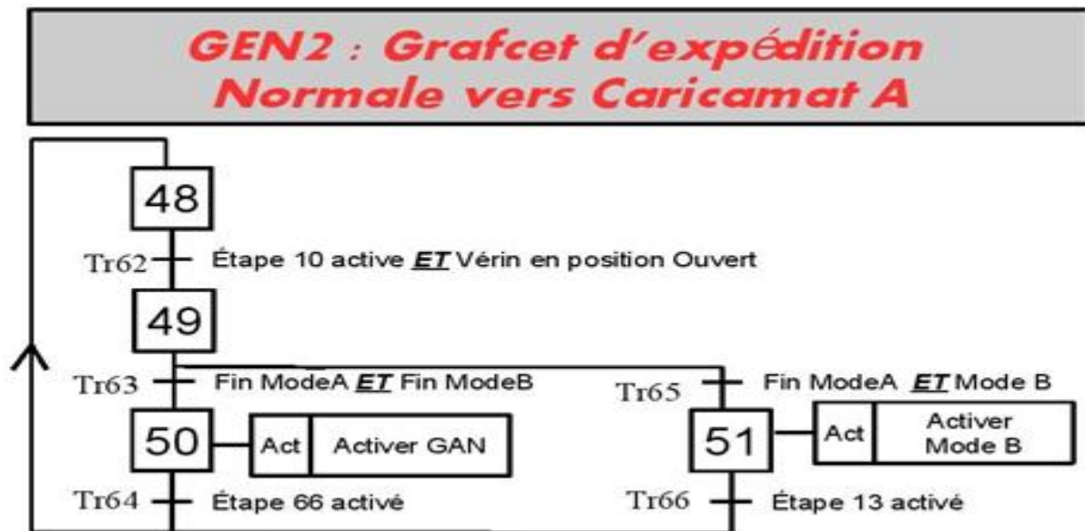
Figure 25: GEN2 – Grafcet d'expédition normale vers caricamat A
