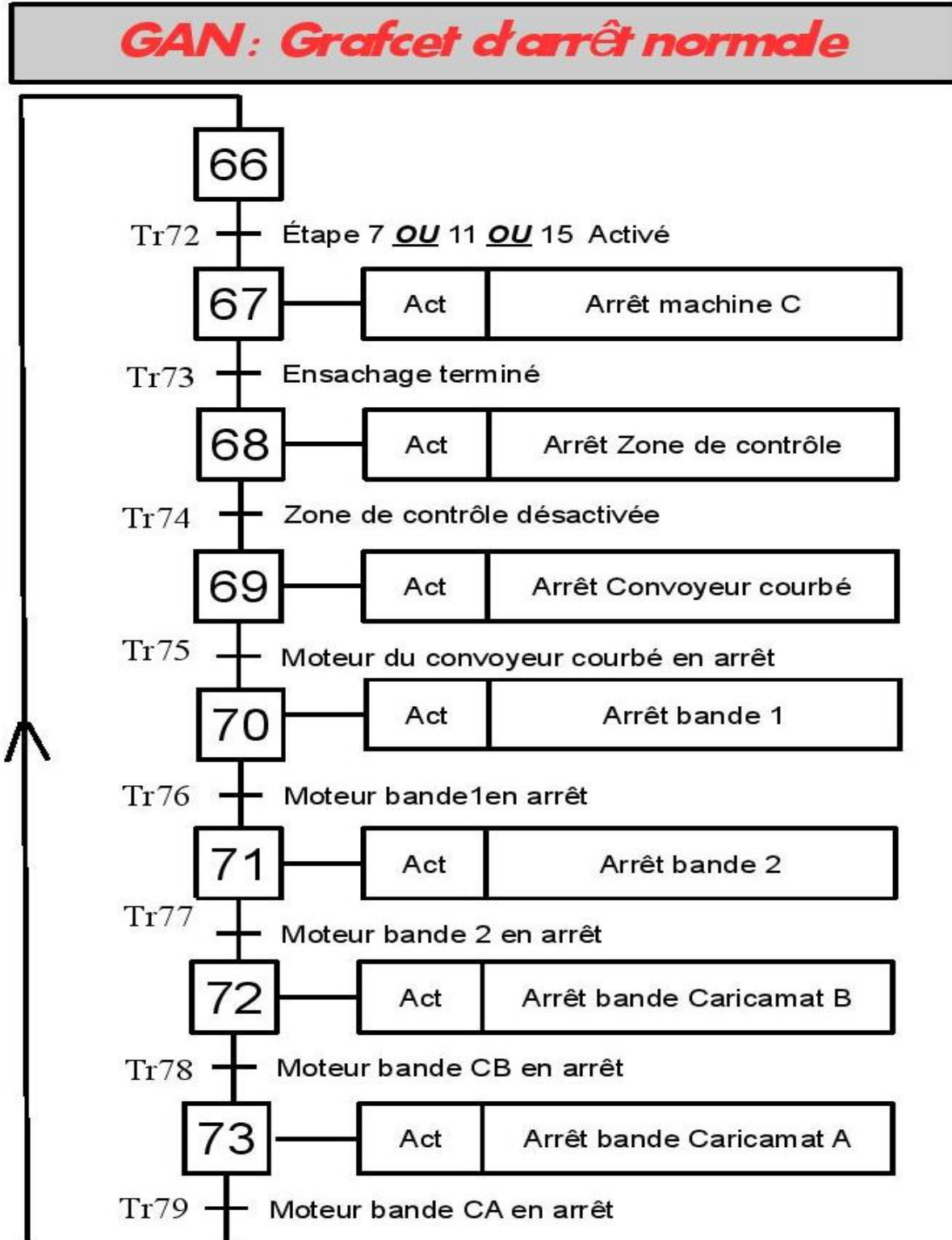
Figure 27: GAN – Grafcet d'arrêt normal
