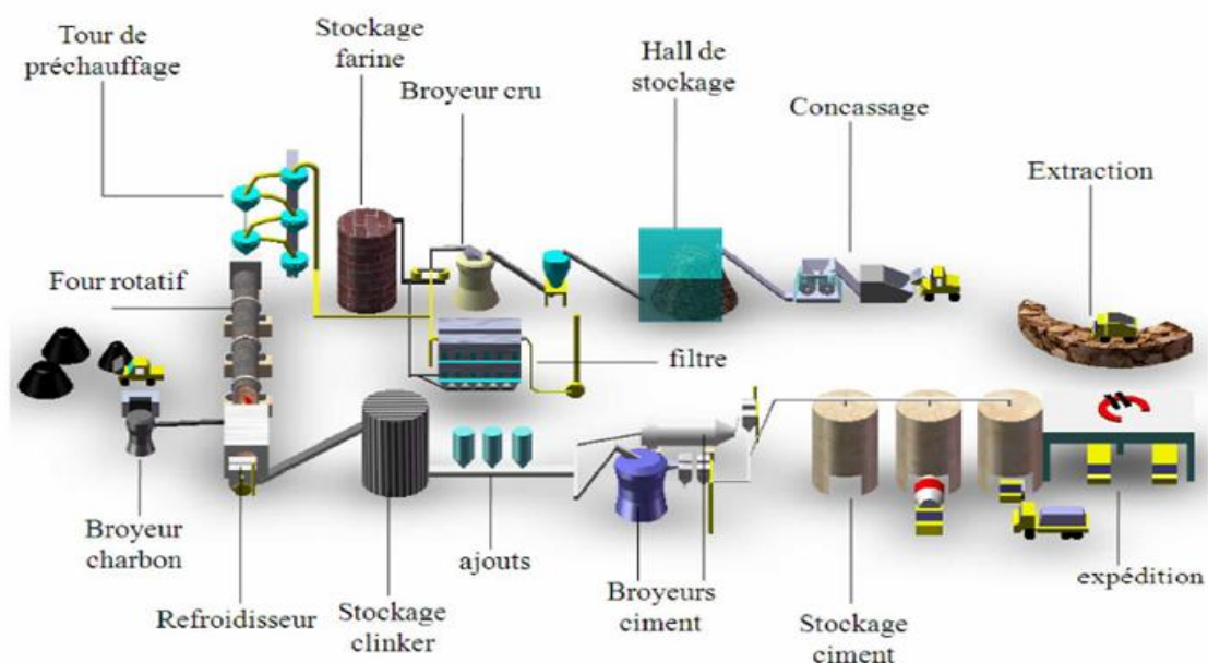
Figure 8 : Chaîne de production du ciment utilisé par Holcim Ras El Ma
