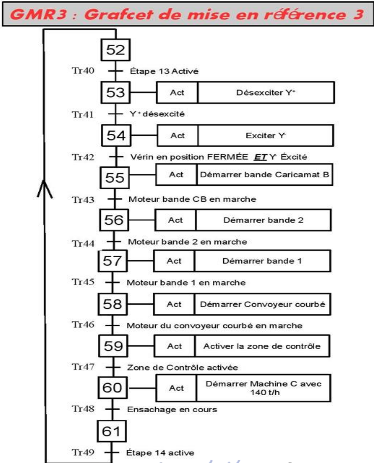
Figure 23: GMR3 – Grafcet de mise en référence 3
