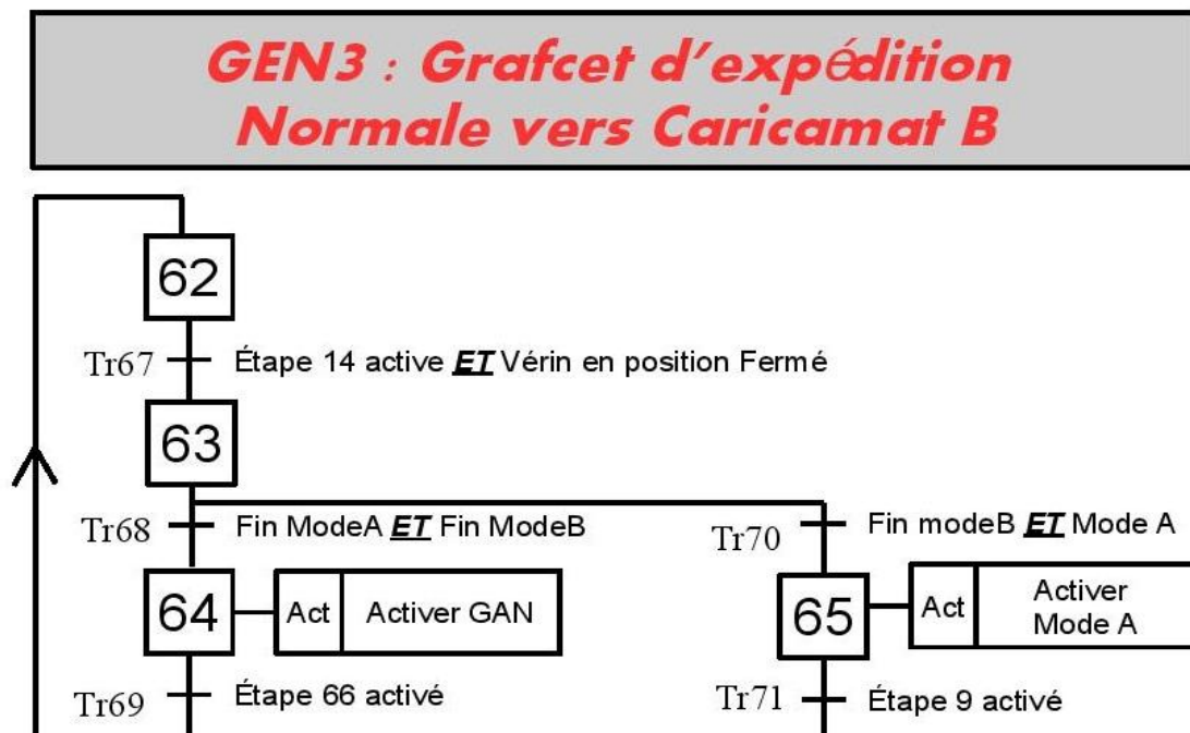
Figure 26: GEN3 – Grafcet d'expédition normale vers caricamat B
