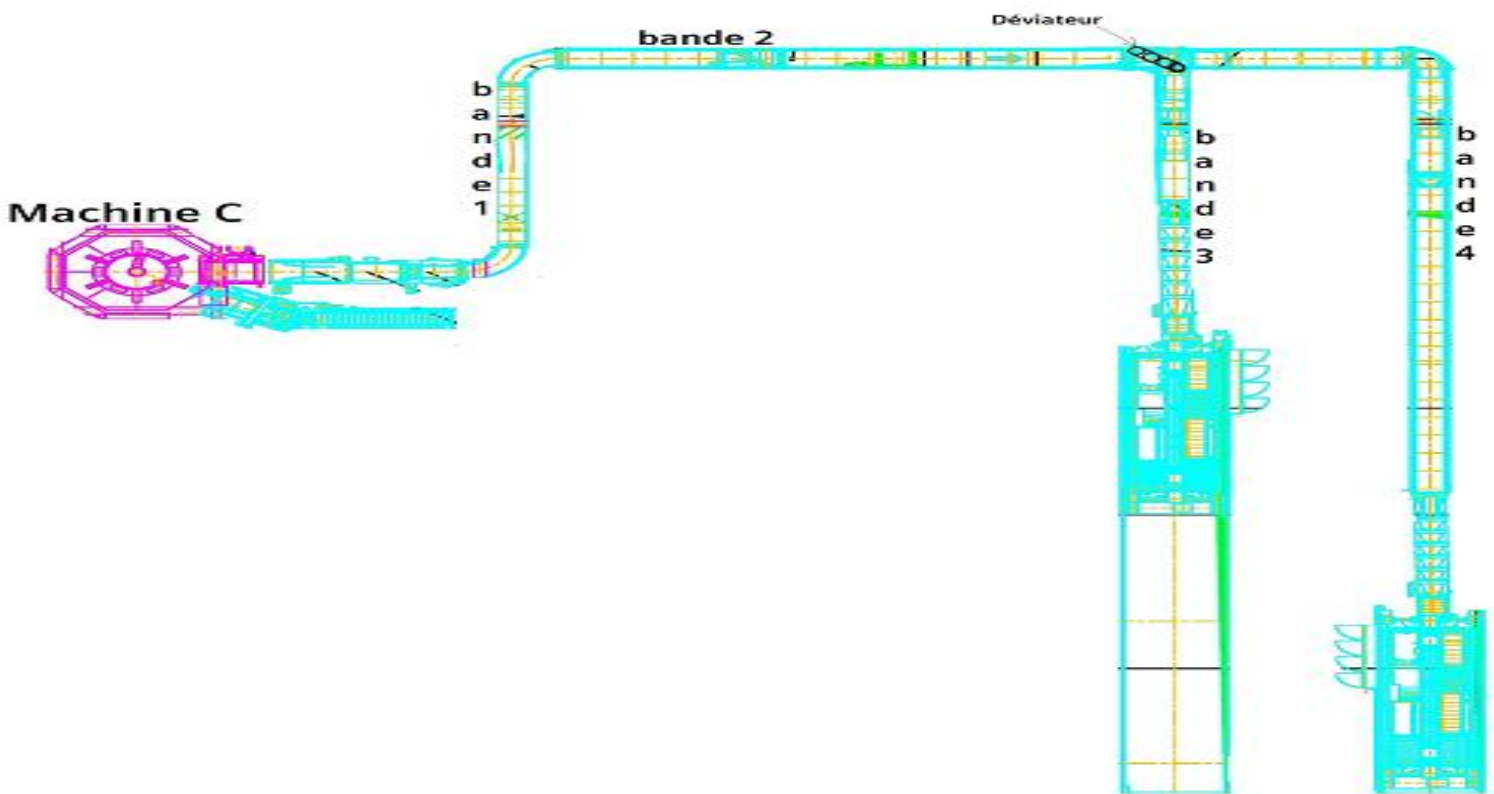
Figure 17 : Plan ligne machine C – Caricamat A&B
