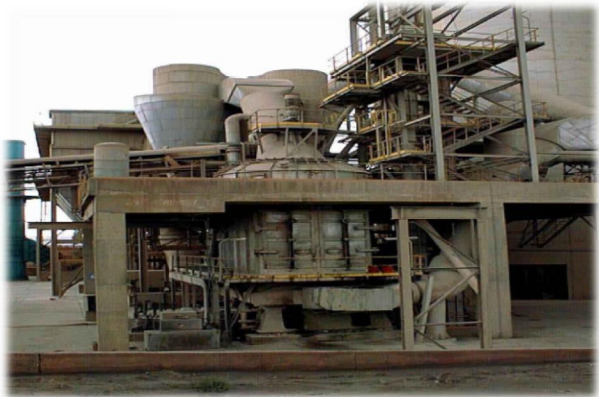
Figure 10 : broyeur vertical à deux paires de galets.
