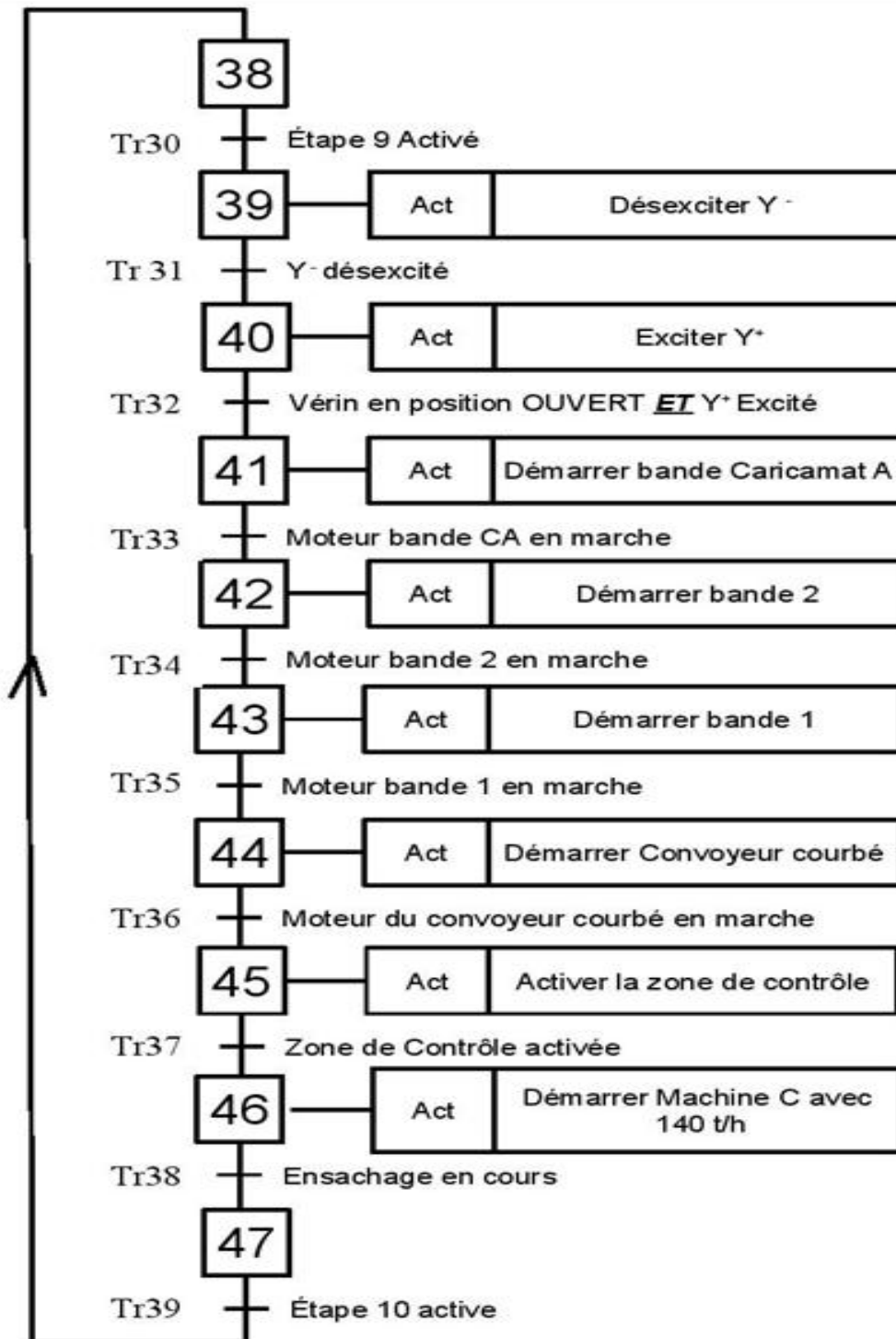
Figure 22: GMR2 – Grafcet de mise en référence 2
