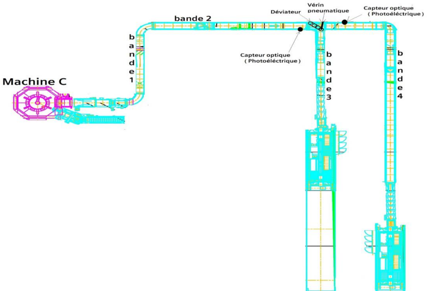
Figure 18 : Plan solution mécanique appliquée sur la ligne machine C – Caricamat A&B
