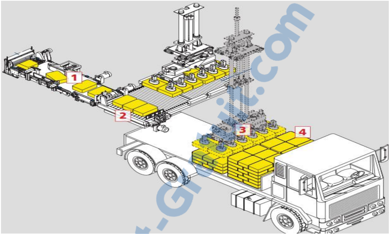
Figure 31: les phases de chargement d'une Caricamat AUTOMATIC Truck loader
