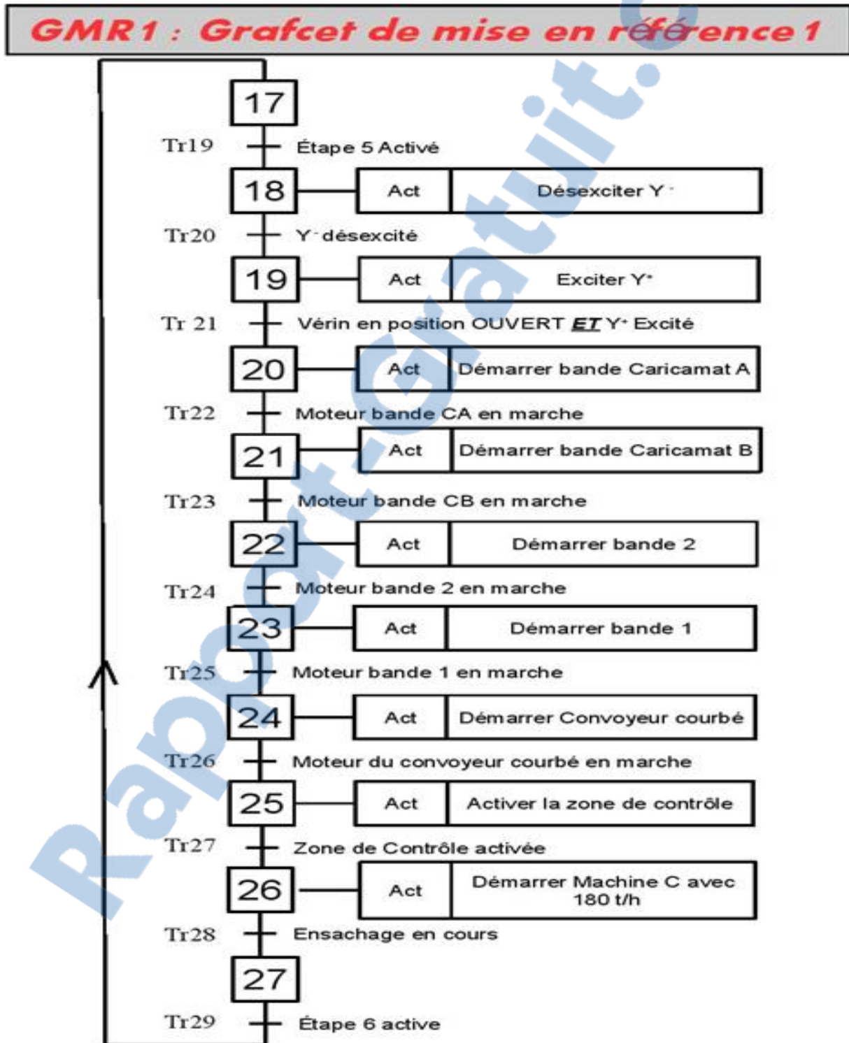
Figure 21: GMR1 – Grafcet de mise en référence 1
