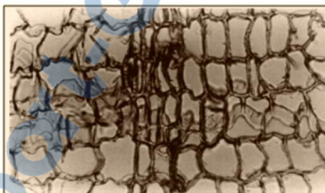
Figure 17 : Limite d'un cerne de liège, liège d'automne (à droite) et liège de printemps (à gauche) (Fortes, 2004)
