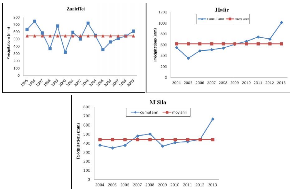
Figure 102: Précipitations annuelles dans 3 suberaies d'étude durant le cycle de production
