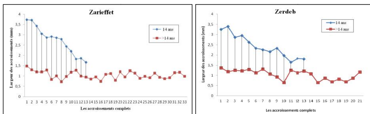
Figure 98 : Evolution des accroissements moyens annuels du liège au cours d'un autre cycle de 14 ans en dehors du cycle normal
