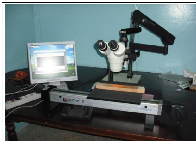
Figure 51: Dispositif de mesure des accroissements du liège LINTAB 5 (Photo originale)
