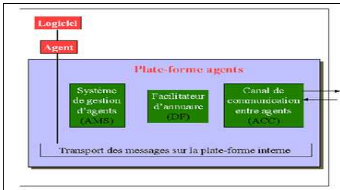
Figure III.1 Le modèle de référence pour une plate-forme multi-agents FIPA
