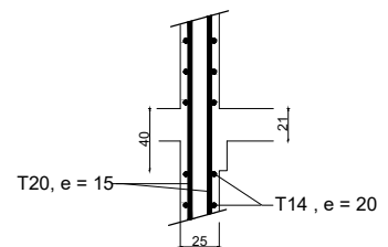
Coupe 7'-7'
