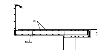
Coupe 4-4
