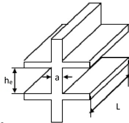
Figure 2.7 Coupe de voile
