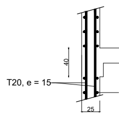
Coupe 3-3
