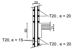
Coupe 9-9
