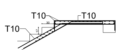
Coupe 10-10
