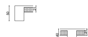
Coupe 6'-6'
