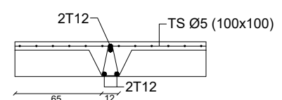
Coupe transversale d'une Poutrelle
