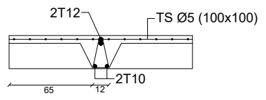
Coupe transversale d'une Poutrelle
