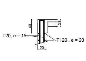
Coupe 3-3
