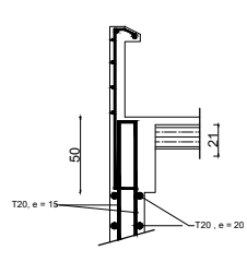
Coupe 9-9
