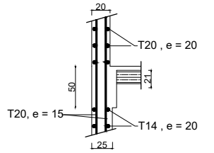
Coupe 9-9
