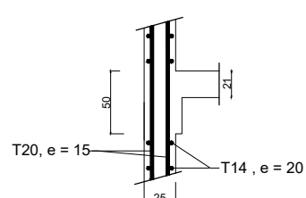
Coupe 4-4
