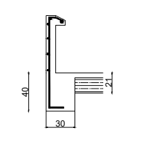
Coupe 3-3
