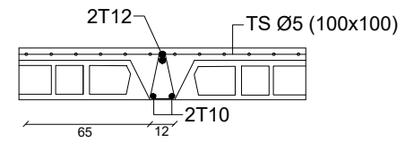
Coupe 12-12
