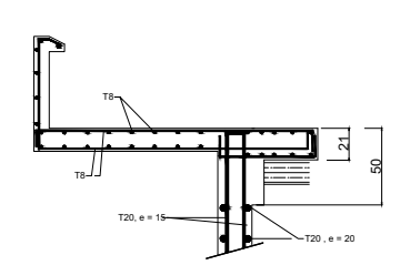
Coupe 4'-4'
