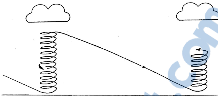
Figure 5 : Exploitation d'une ascendance thermique par un vautour fauve, d'après Pennycuik, 1973 (52).
