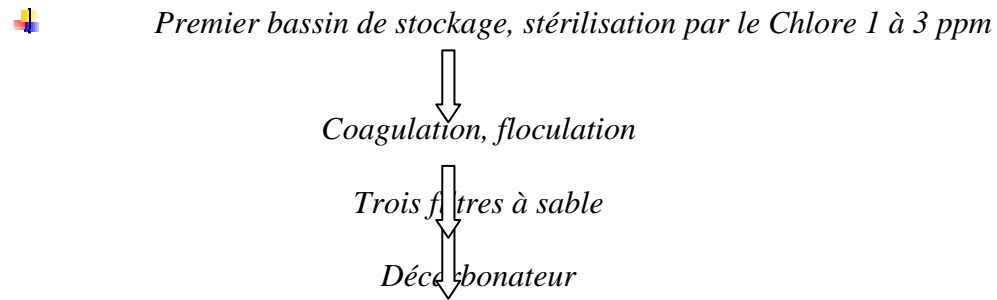
Figure 3 : Première phase du traitement de l'eau
