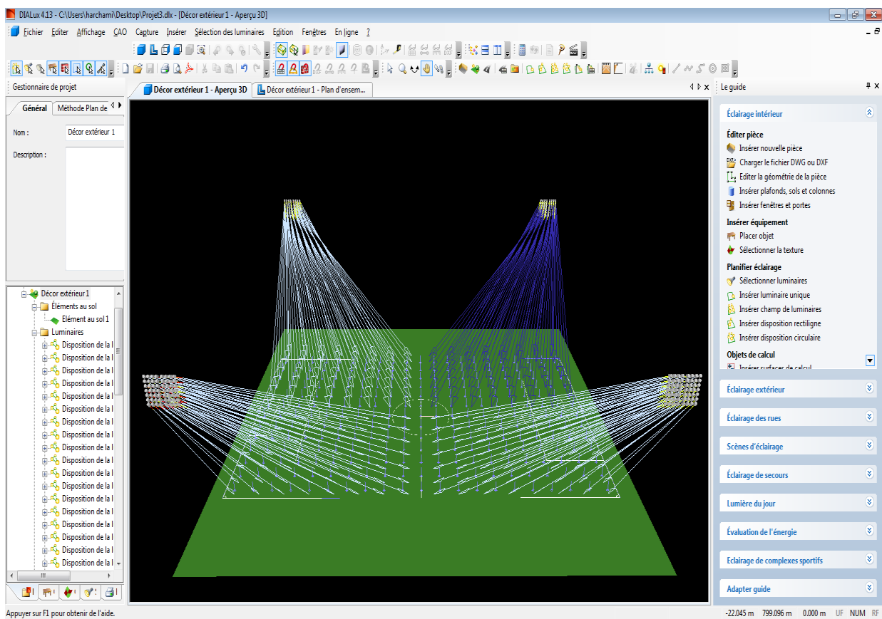
FIGURE 06 : Points d'illumination des projecteurs.
