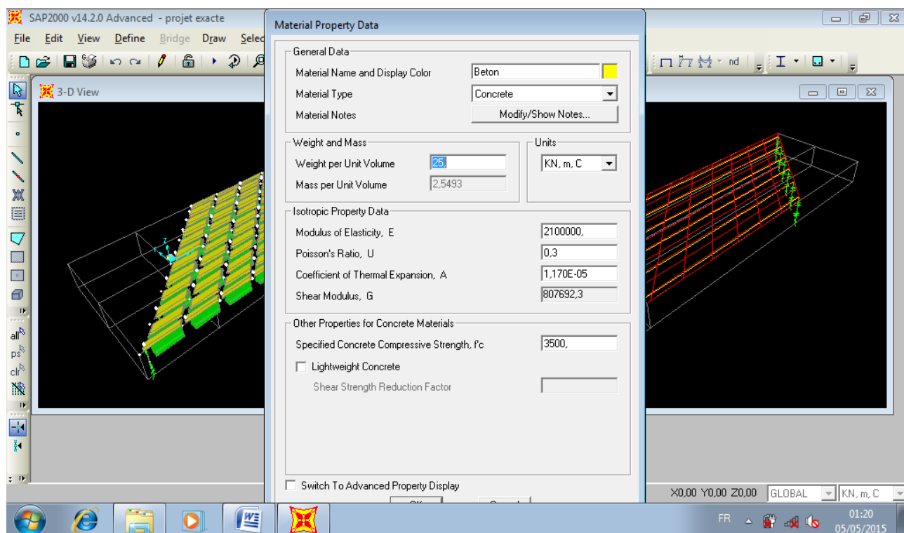
Fig.4.6 : définition de matériaux de réalisation de bridge
