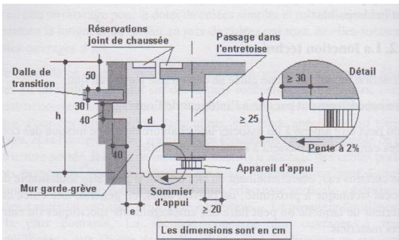
Fig. 8.1 : les différents éléments d'une tête de culée
