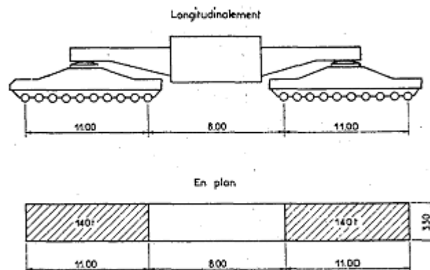
Fig 3-5 : Disposition du système D
