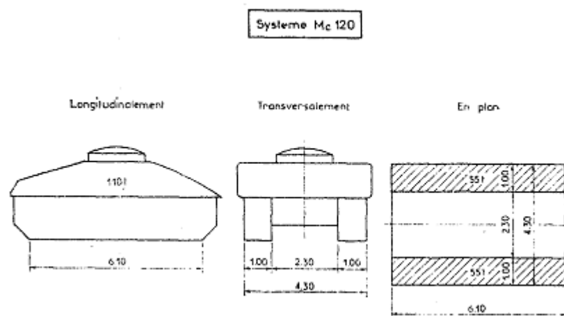
Fig 3-3 : Disposition du système Mc 120
