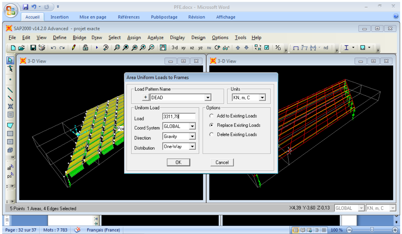
Fig.4.17: chargement du tablier
