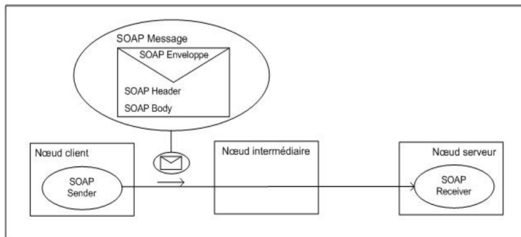
Figure 1.2 : Structure d'un document SOAP
