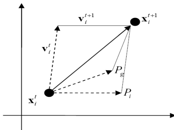
Figure 2.5 : Schéma de principe du déplacement d'une particule
