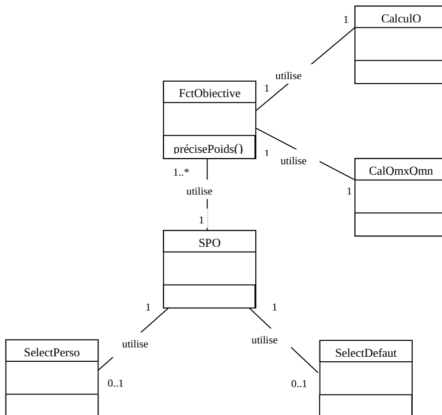
Figure 3.3 : Diagramme de classes
