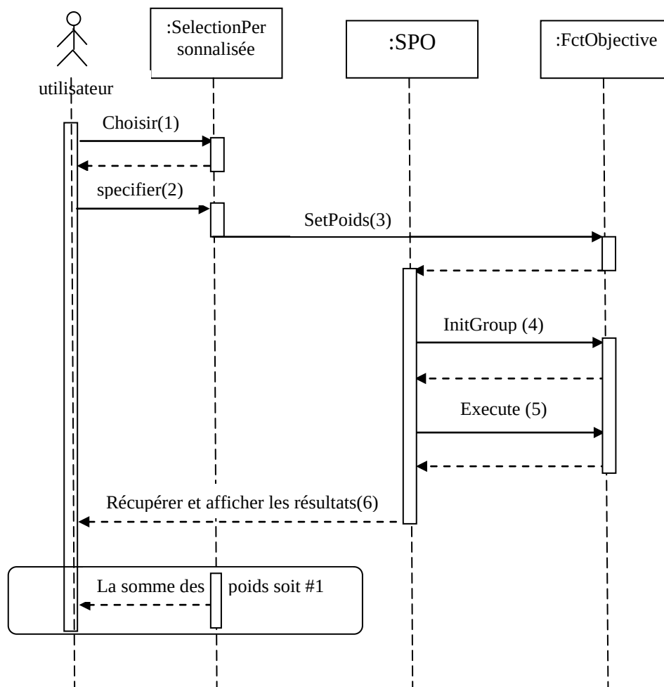
Figure 3.2 : Diagramme de séquence (exemple de sélection personnalisée)
