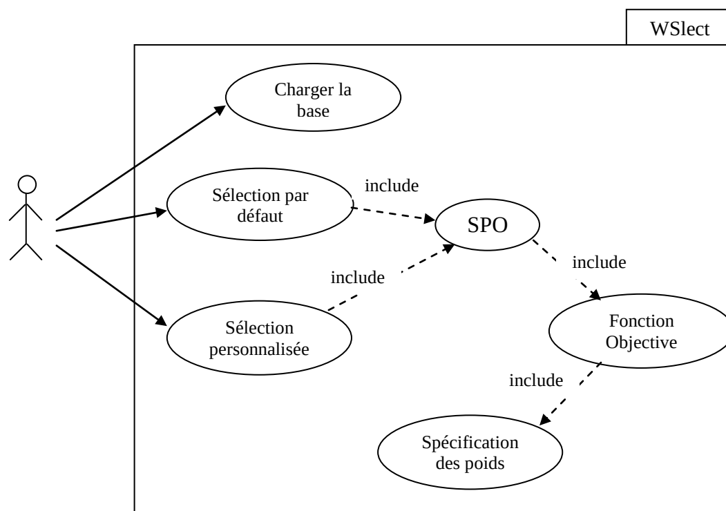
Figure 3.1 : Diagramme de cas d'utilisation
