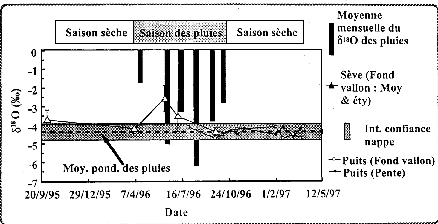
Figure 31 : Evolution saisonnière de \delta^{18}\text{O} des pluies, des nappes et de la sève brutes des faidherbias.
