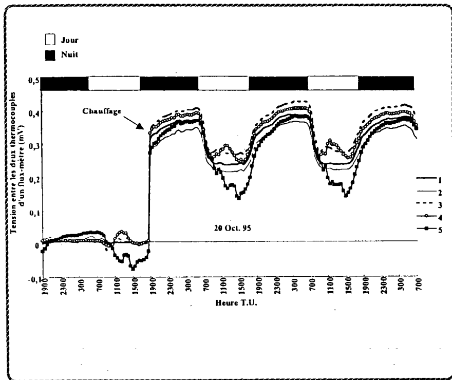
Figure 17 : Enregistrement de la tension électrique aux bornes de 5 fluxmètres avant et après chauffage.
