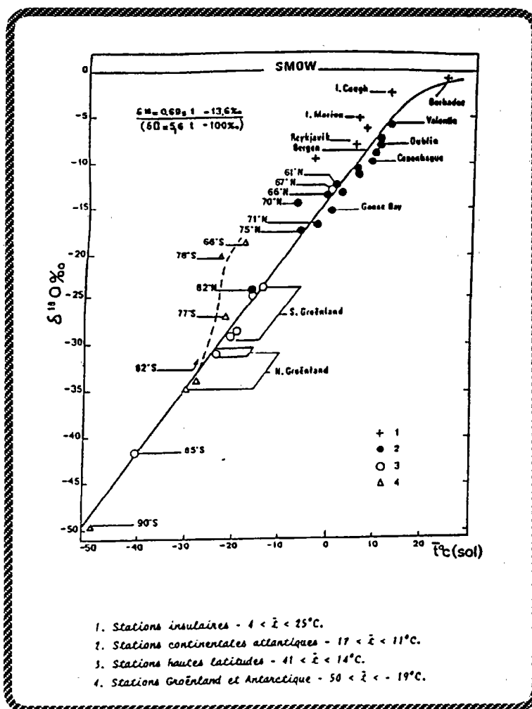
Figure 22 : Relation entre la composition isotopique annuelle moyenne des pluies ( \delta^{18}\text{O} ) et la température annuelle moyenne du sol.
