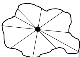
Figure 3 : Exemple d'un barycentre
