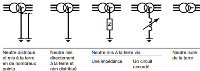
Figure 8 : Différents régimes de neutre dans le monde
