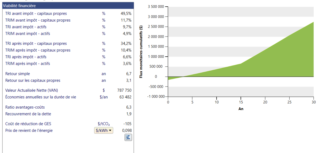
Figure 16 : Résultats de la simulation financière sur 20 ans avec réseau électrique
