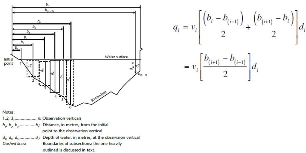
Figure 2 : Méthode de calcul des débits partiels
