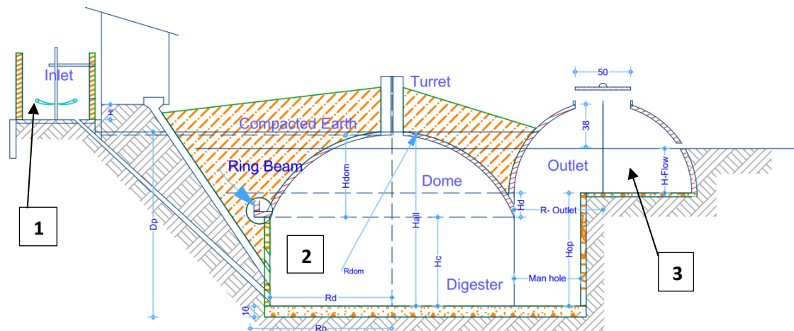
Fig. 4 : plan de construction d'un digesteur domestique à dôme fixe tel qu'installé par le programme FONERWA au cours de l'année 2017. Selon les plans originaux, ces plans sont adaptés de 4 à 10 m 3 . Source [9].
