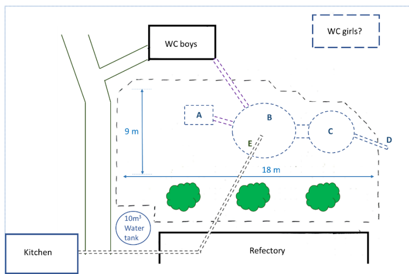
Fig. 25: plan du digesteur issu de l'étude de faisabilité présentée en annexe 22. Légende : A) chambre d'alimentation, B) chambre de digestion, C) chambre d'évacuation, D) conduite d'évacuation du digestat, E) conduite de gaz. Les toilettes pour filles (en haut à droite) sont un projet à l'étude afin d'augmenter l'apport en substrat.
