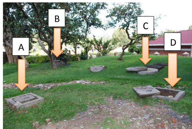
Fig. 5 : digesteur de l'hôpital de Karongi. (A) et (D) : regards sur chambres d'évacuation secondaires, (B) : évacuation du digestat, (C) : chambre d'évacuation principale. Photo prise le 29.05 à l'hôpital de référence de Karongi.
