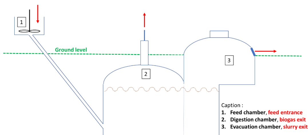
Fig. 11: schéma simplifié d'un digesteur à dôme fixe du projet FONERWA, d'un volume total d'environ 4m 3 .
