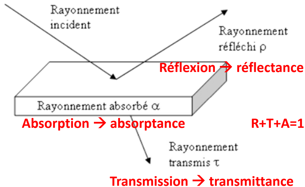
FIG. 2.3 – Absorption, réflexion et transmission (Bonn et Rochon, 1993)
