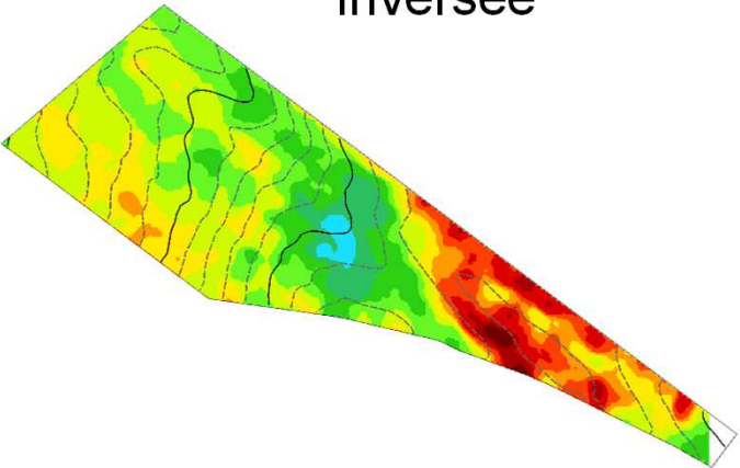
Carte de résistivité inversée
