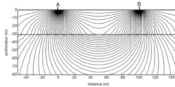
Résistif sur conducteur
