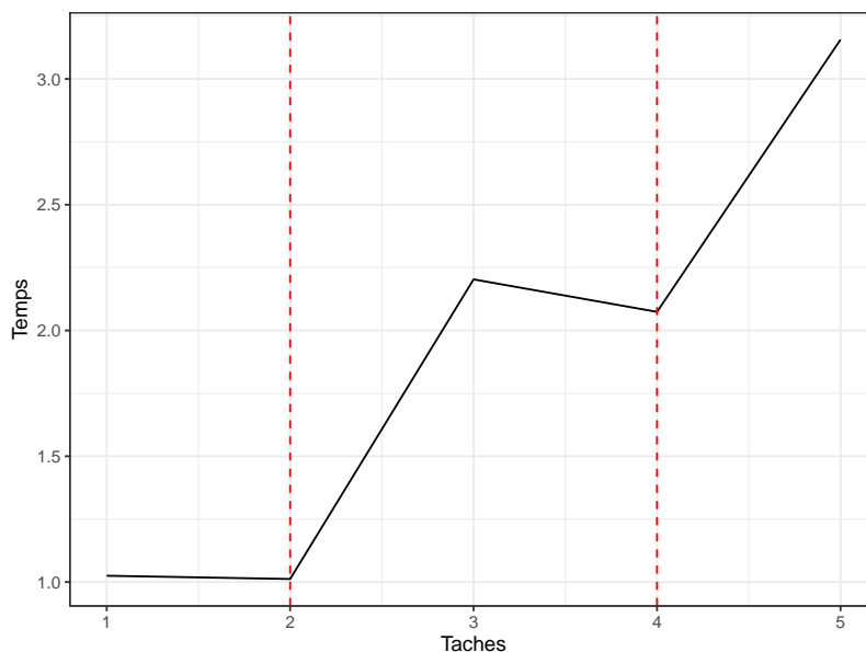
FIG. 2.2 : Temps d'exécution en parallèle de tâches nécessitant une seconde (chaque tâche est une pause d'une seconde). Le nombre de tâches varie de 1 à deux fois le nombre de coeurs utilisés (égal à 2) plus une.
