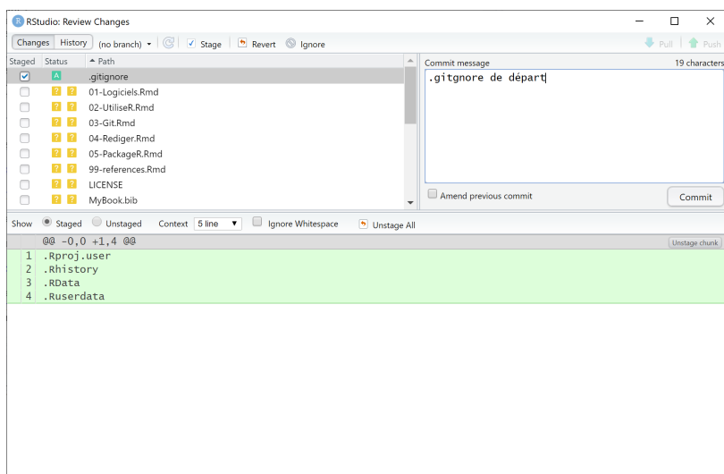
FIG. 3.4 : Fenêtre de validation des modifications prises en compte.
