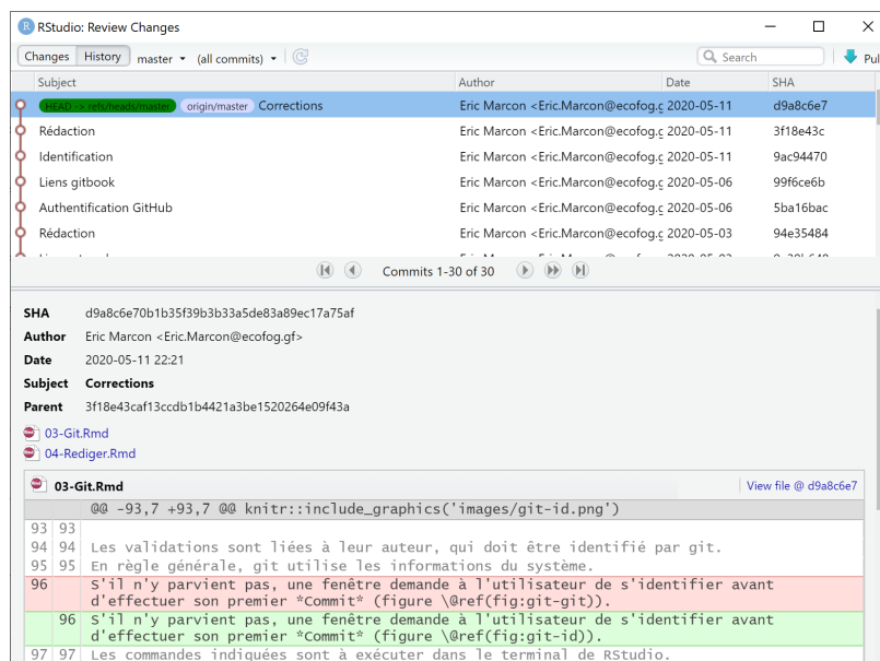
FIG. 3.12 : Historique des validations dans le dépôt.
