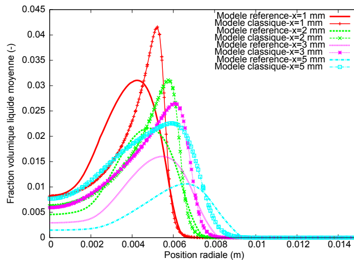
FIG. V.18 : Comparaison des profils transversaux de la fraction volumique liquide moyenne \bar{c} (-) près de la sortie de buse : modèle de référence et modèle classique
