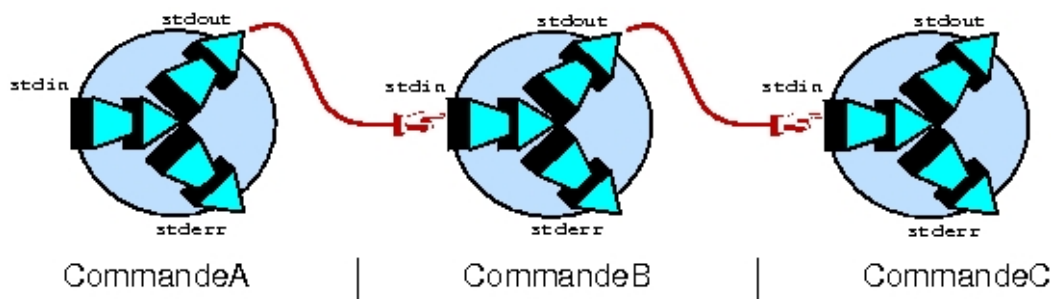
FIG. 4.2 – Enchaînement de commandes, mécanisme du pipe .
