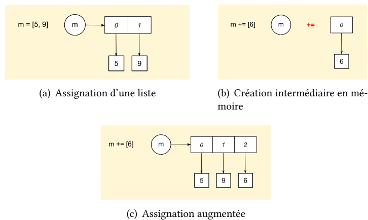
FIGURE 4.2 – Assignation augmentée d'un objet modifiable.
