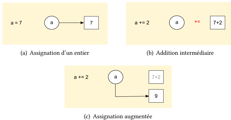
FIGURE 4.1 – Assignation augmentée d'un objet non modifiable.
