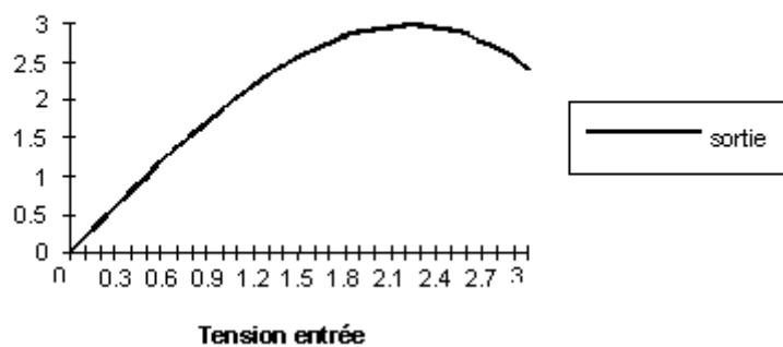
Caractéristique statique non-linéaire
