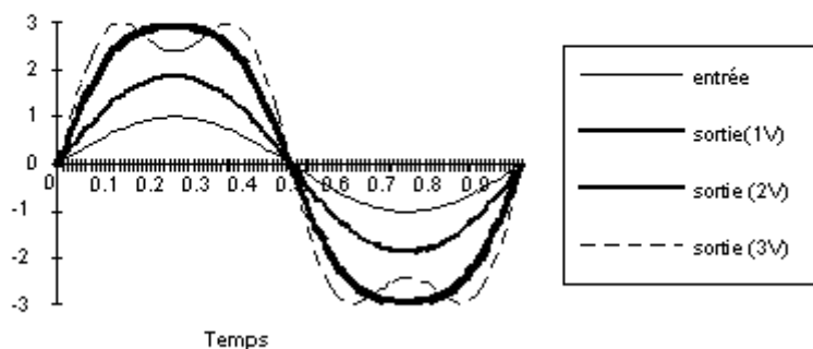
Réponse d'une caractéristique statique linéaire
