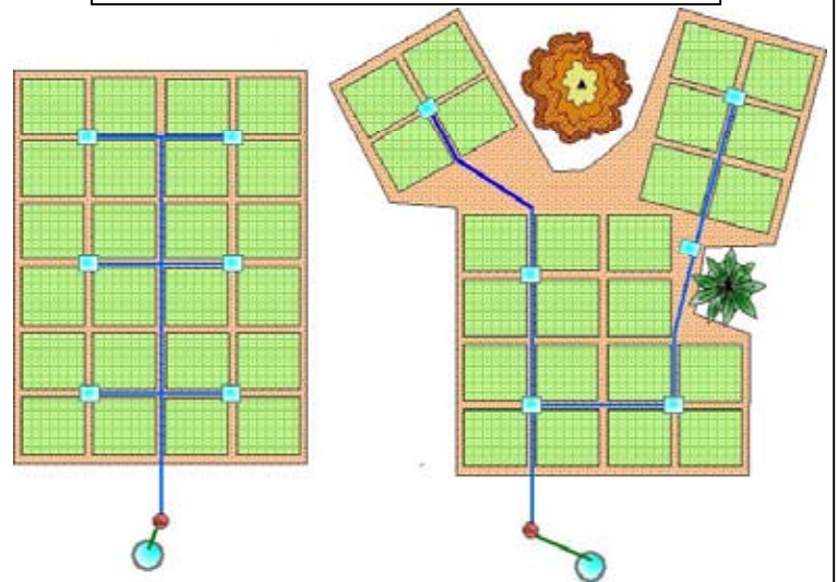
Exemple de disposition des champs irrigués
