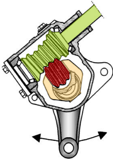
A vis globique et galet
