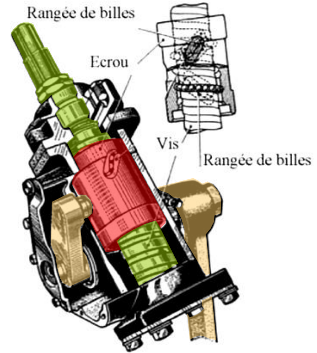
A recirculation de billes
