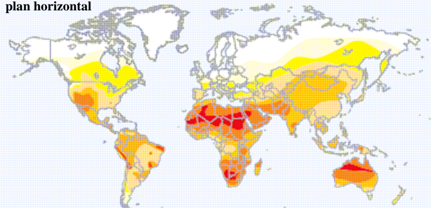
Carte du monde de l'irradiation moyenne annuelle en \text{kWh/m}^2/\text{jour} sur un plan horizontal
