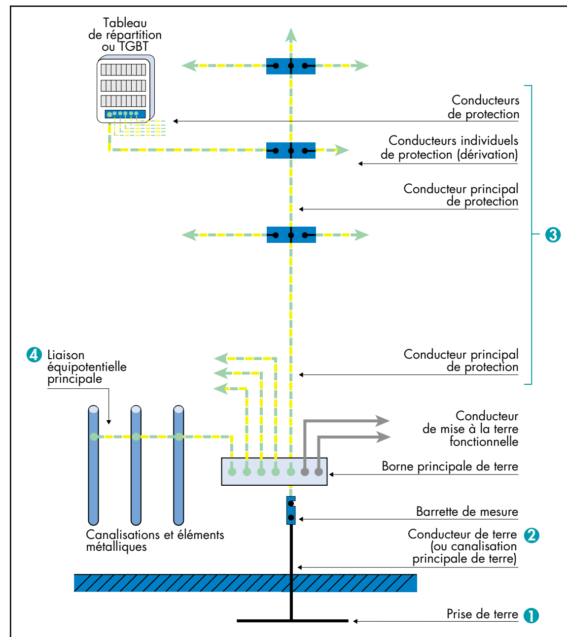
Circuits de terre en bâtiment collectif
