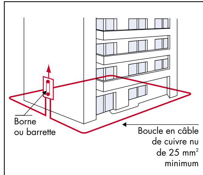
Boucle à fond de fouille
