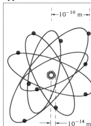
Figure 5.21. Modèle simple d'un atome. Sous l'influence de forces électriques, les électrons chargés négativement sont en orbite autour d'un noyau de petite taille mais de masse importante. Le noyau, qui n'est pas représenté à l'échelle, comprend deux types de nucléons: des protons chargés positivement et des neutrons sans charge.
