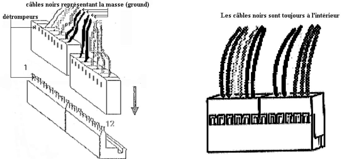
Figure 6 : Connecteurs d'alimentation.
