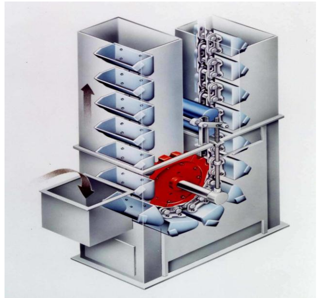
Figure 5: Elévateur à godets.
