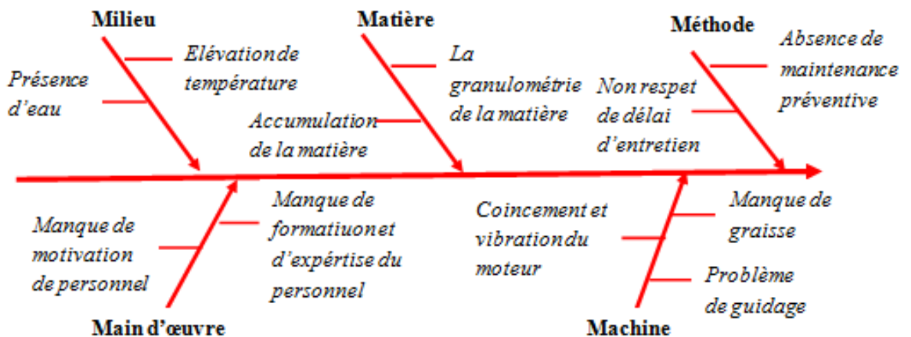
Figure 14: Diagramme d'ISHIKAWA
