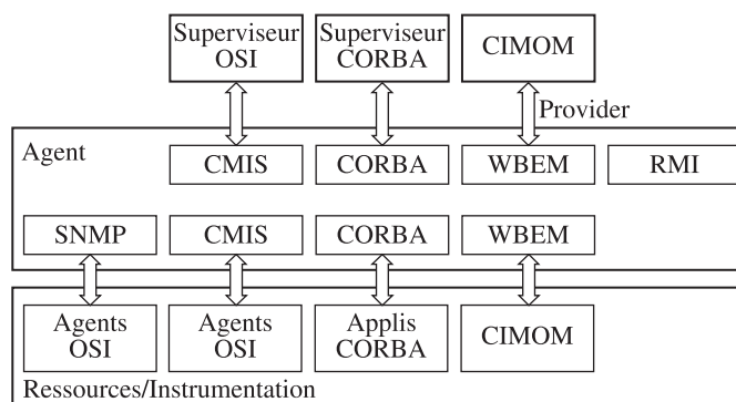
Figure 6.11. Interopérabilité JMX / approches standard
