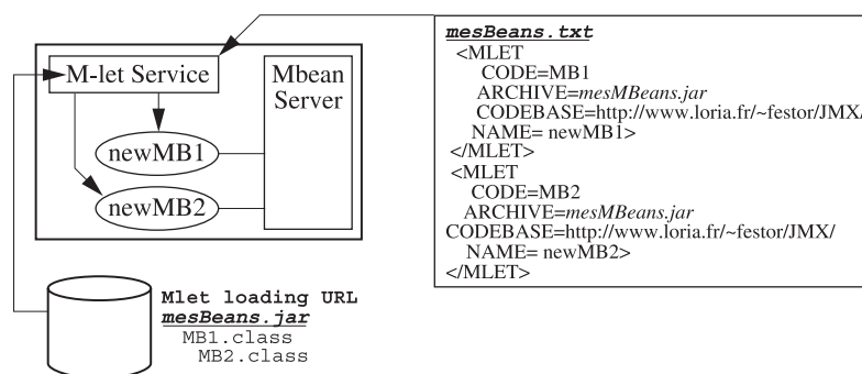
Figure 6.10. Chargement d'objets gérés distants par le service Mlet
