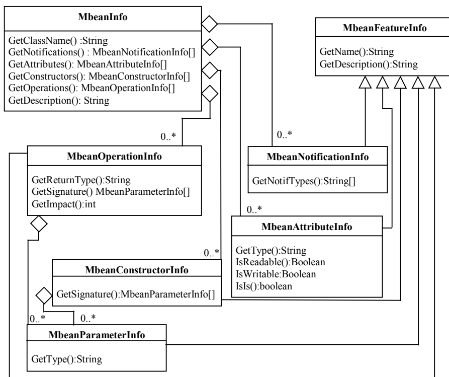
Figure 6.4. Les composants de l'interface MbeanInfo
