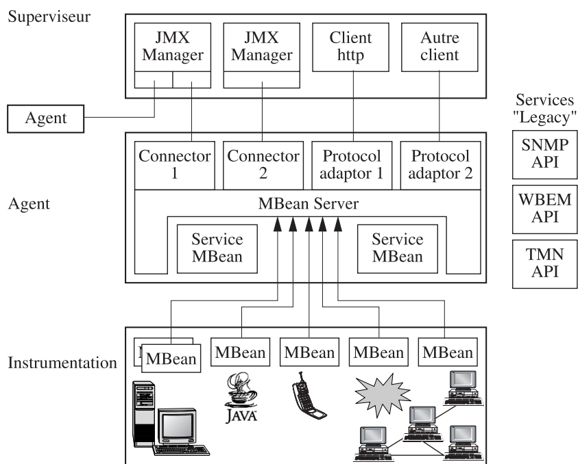
Figure 6.1. L'architecture générale de JMX
