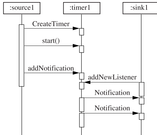
Figure 6.8. L'instanciation et l'exploitation du service de timer
