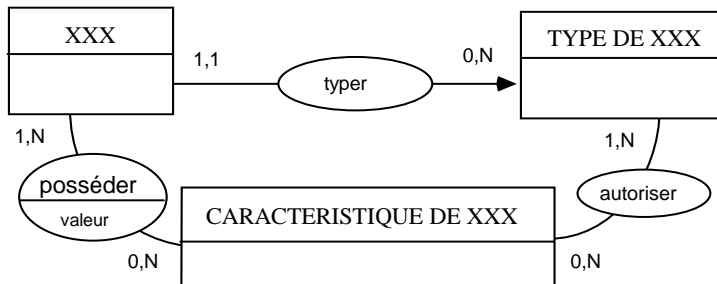
MCD replié
