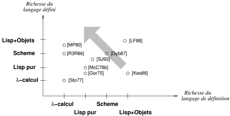
FIG. 1.1 – Classification de quelques évaluateurs
