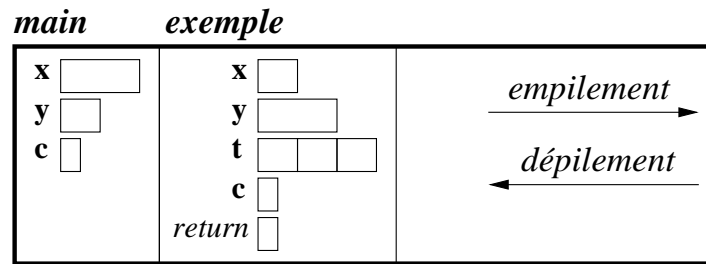
FIG. 13.2 – La pile pendant l’appel de fonction exemple
