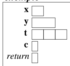
FIG. 13.1 – Zone de mémoire occupée par la fonction exemple
