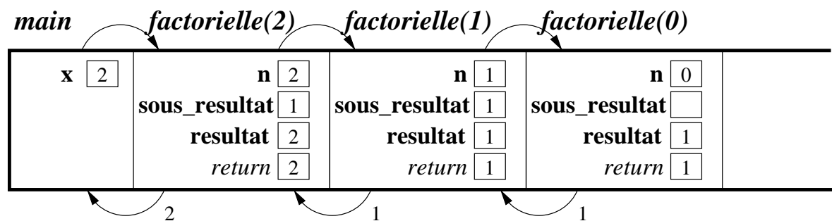
FIG. 13.3 – Enchaînement des appels récursifs pour factorielle(2)
